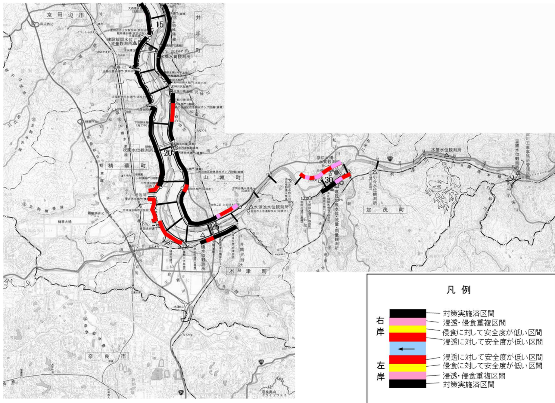
木津川下流 堤防詳細点検及び対策位置図（2／2）（令和3年8月時点）
