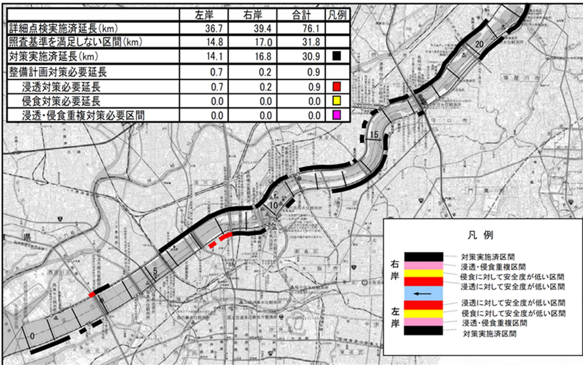
淀川 堤防詳細点検及び対策位置図（1 / 2）（令和3年8月時点）
