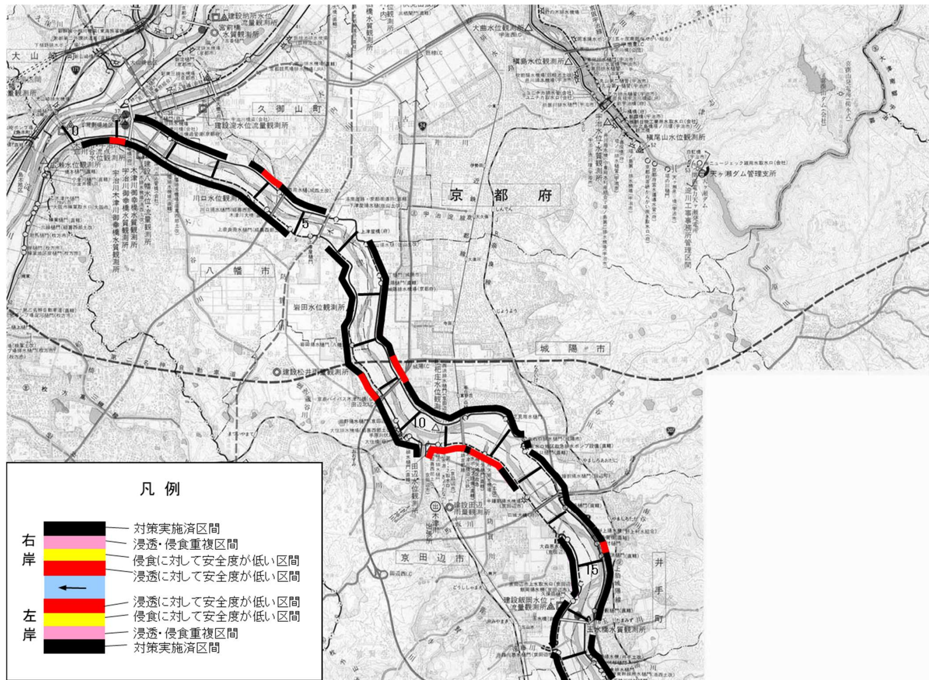
木津川下流 堤防詳細点検及び対策位置図（1 / 2）（令和3年8月時点）
