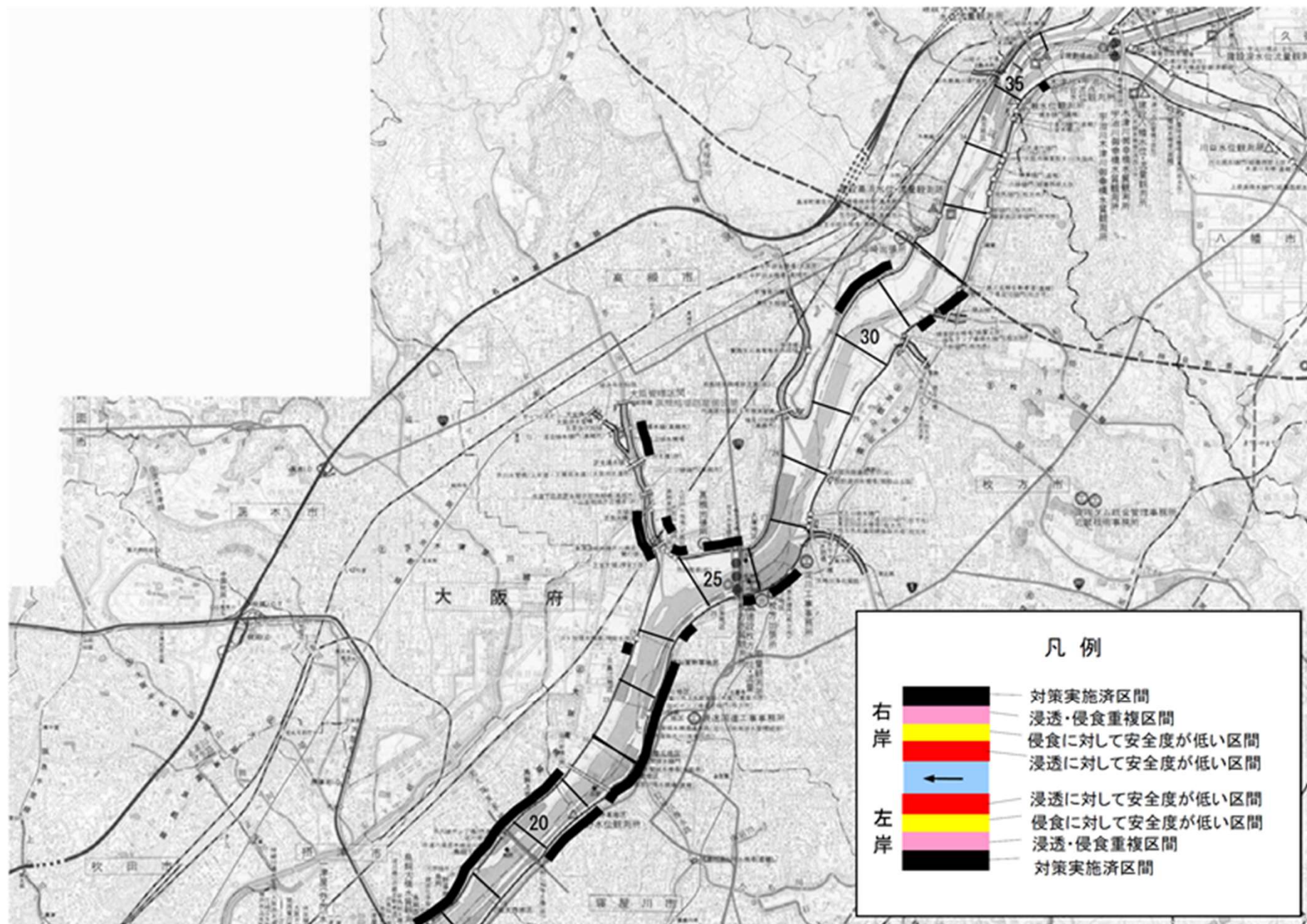
淀川 堤防詳細点検及び対策位置図（2／2）（令和3年8月時点）
