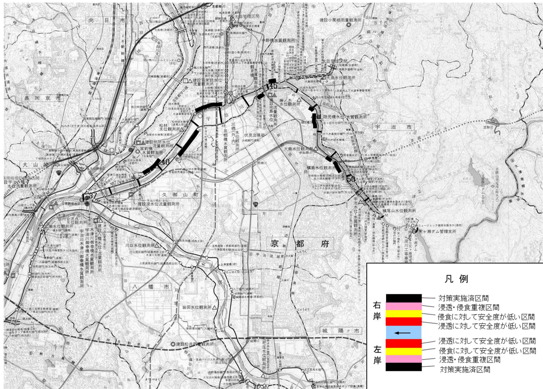
宇治川 堤防詳細点検及び対策位置図（令和3年8月時点）
