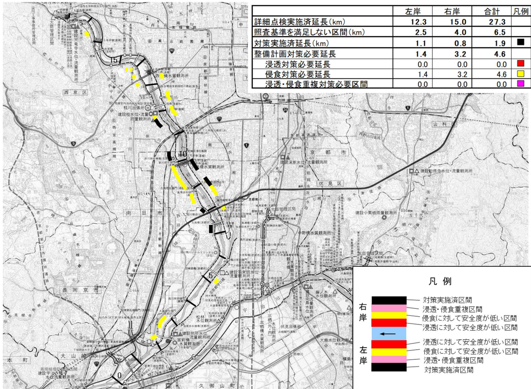
桂川 堤防詳細点検及び対策位置図（令和3年8月時点）
