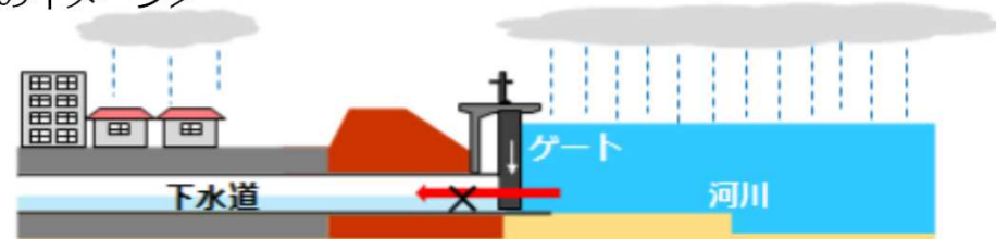
＜樋門による逆流防止のイメージ＞
