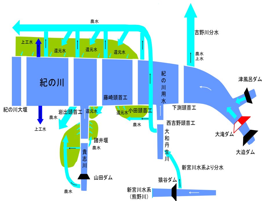
図 2. 2. 2 利水概要図
