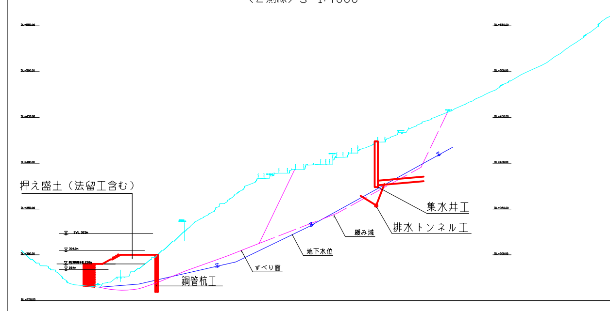
第1案 押え盛土+鋼管杭+地下水排水工案 断面図 (2測線) S=1:4000
