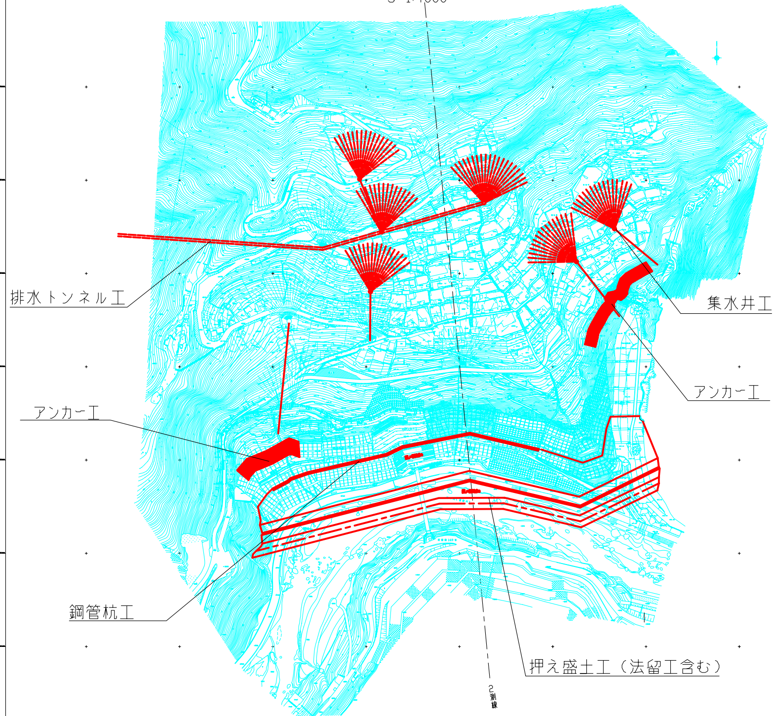
第1案 押え盛土+鋼管杭+地下水排除工案 平面図
