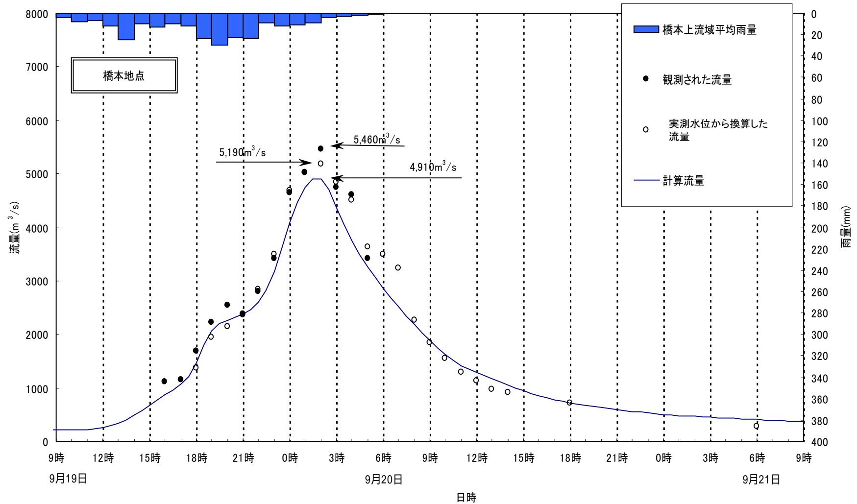
平成2年9月 ハイドログラフ(実測流量と計算流量)
