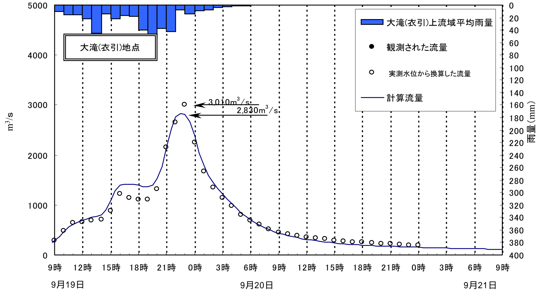
平成2年9月 ハイドログラフ(実測流量と計算流量)
