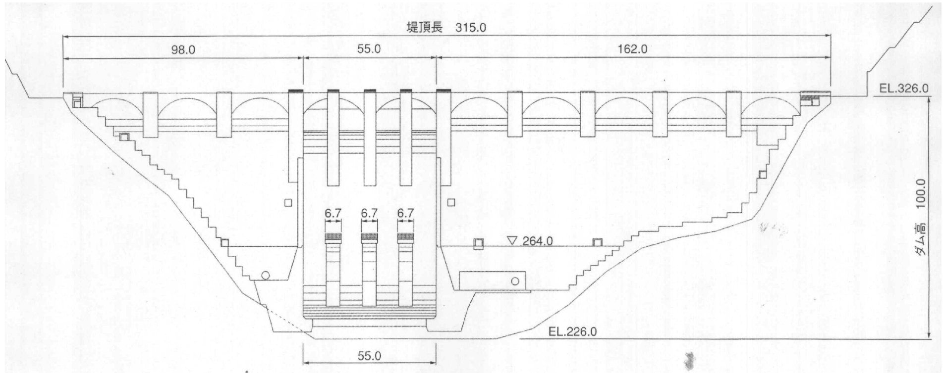
図 1 2 大滝ダム堤体図 (ダム下流面図)
