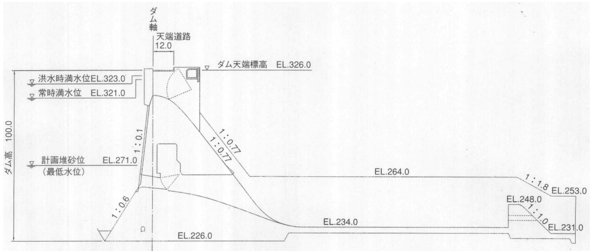
図 1 3 大滝ダム堤体図 (堤体断面図)
