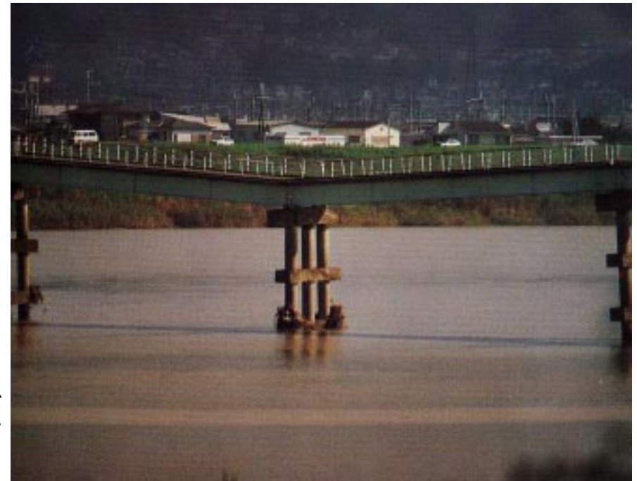
平成2年 台風10号 床上浸水 5戸 床下浸水 95戸 (水害統計より) 写真は、洪水により河床が えぐり取られて陥没した南 海橋
