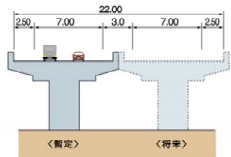
■橋梁部
