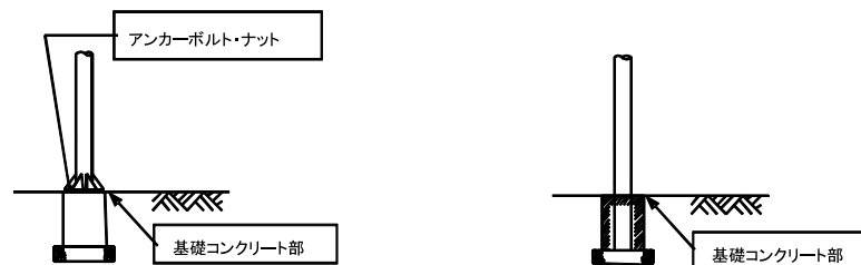
【ベースプレートが露出している場合】
