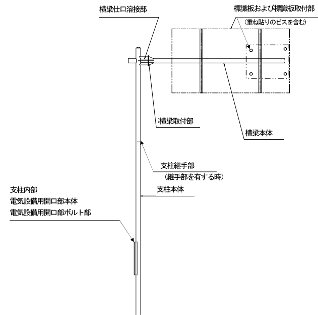
付図-1-4 主な点検箇所 (逆L型)
