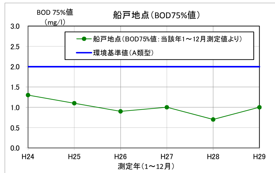
▲紀の川本川の水質状況 (船戸地点・近5ヶ年)
