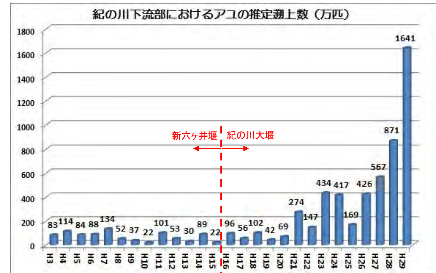
▲紀の川大堰魚道におけるアユの推定遡上数
