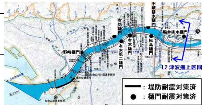
▲ 堤防・樋門の耐震対策実施状況
