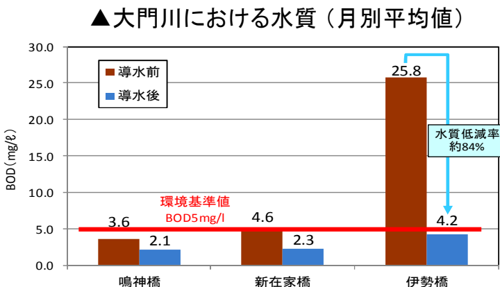
▲大門川における試験導水前後の水質 (H28)
