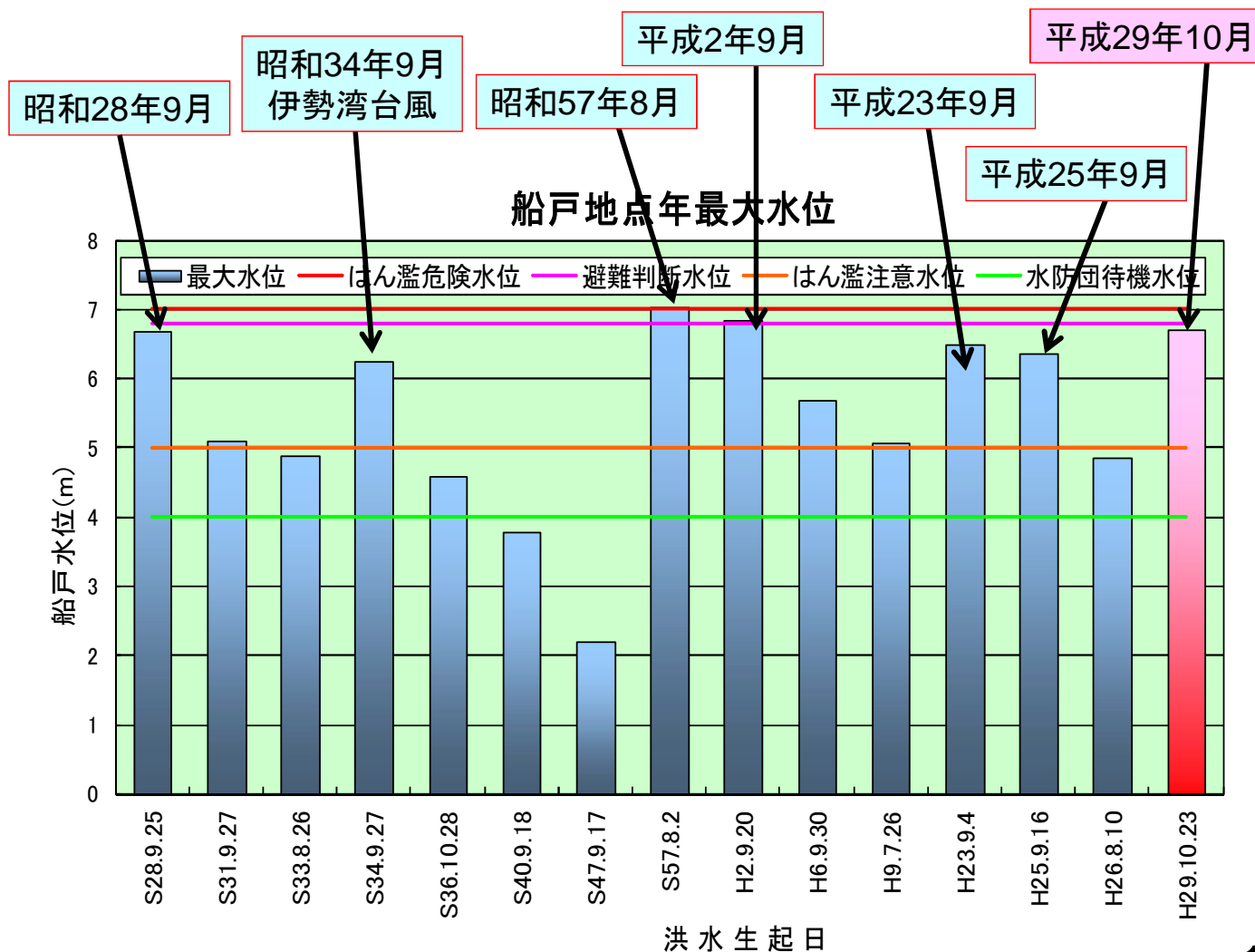
主要洪水最高水位(毎正時)
