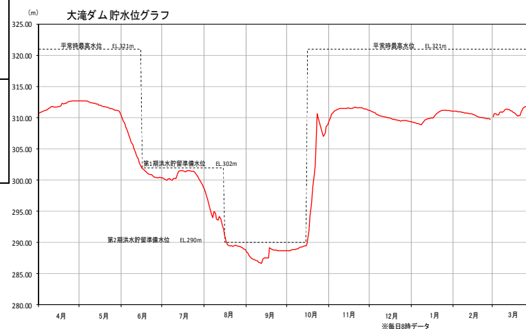
▲大滝ダム貯水池運用図(平成29年)
