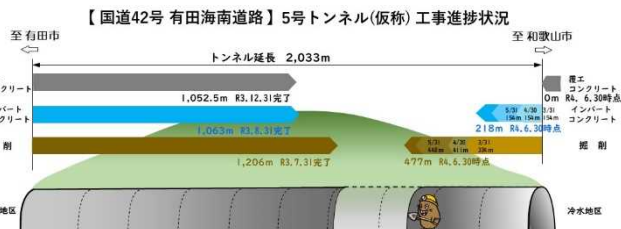
トンネル工事進捗状況(冷水地区側)
