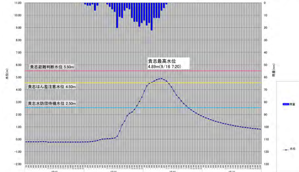
出水概況図(貴志川)
