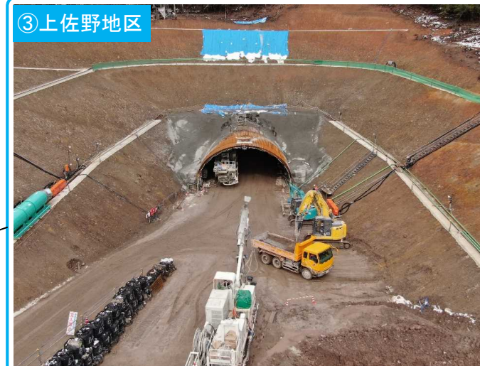
③上佐野地区 佐野トンネルでは、現在坑口から約37m付近まで掘削が進んでいます。今後も安全に配慮しながら工事を進めていきます。
