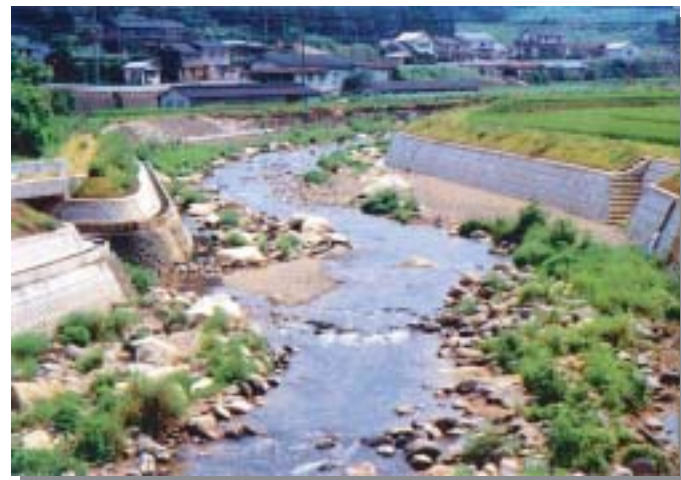
河床への転石再配石 養父町三谷(ポケットパーク三谷)
