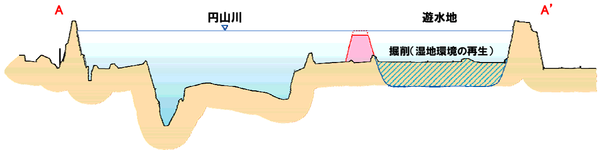
図 4.1.8 遊水地横断面図
