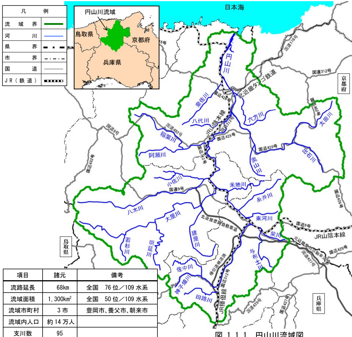
図 1.1.1 円山川流域図
