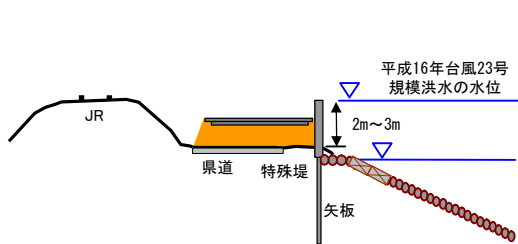
図 4.1.3 堤防の施工横断イメージ
