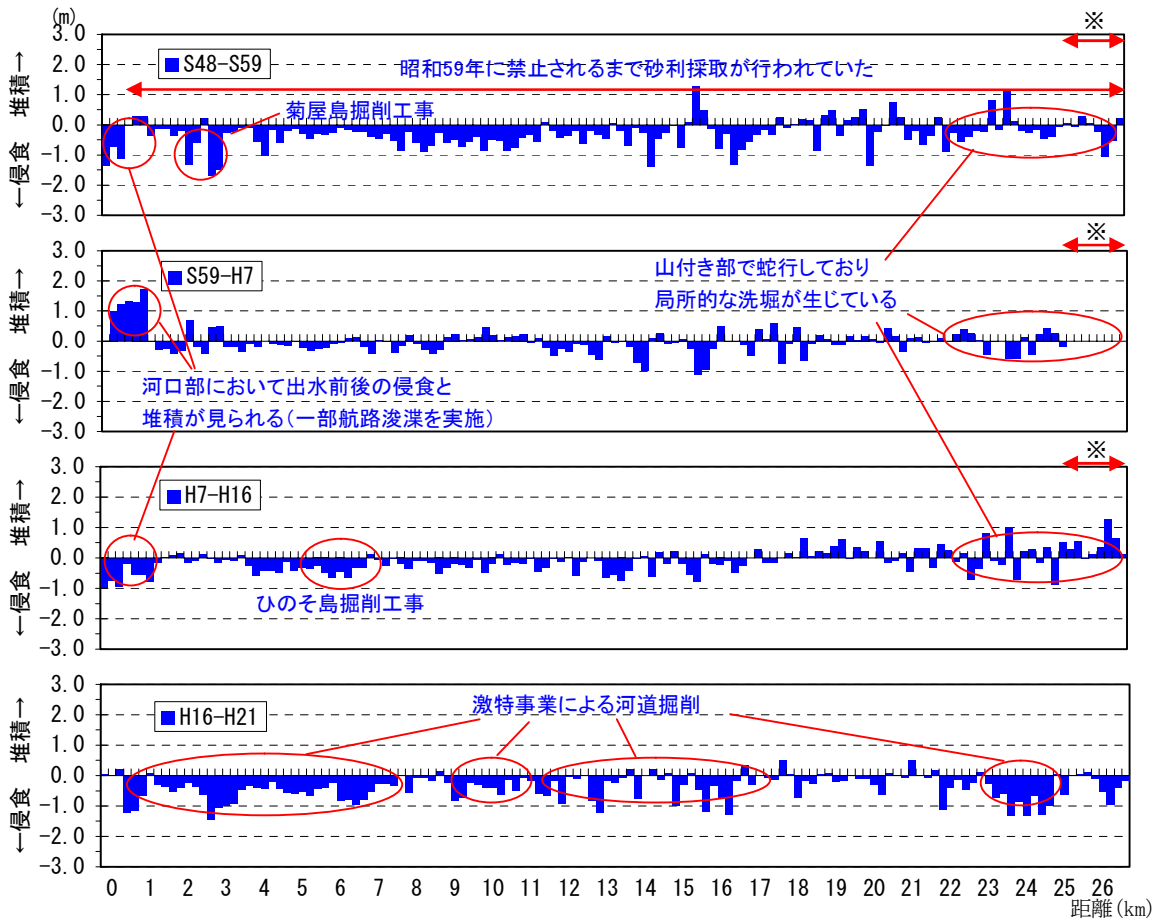
図 2.4.10 河床の経年変動（昭和 48 年度～平成 21 年度）
