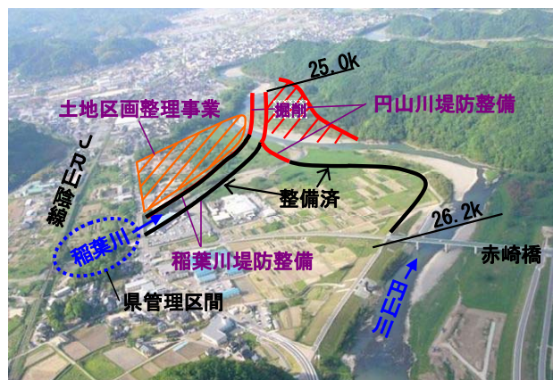
図 4.1.4 稲葉川合流部無堤対策の概要図
