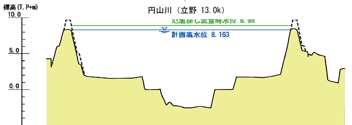
図 2.1.10 市街地区間における洪水位 (平成 16 年 10 月洪水)
