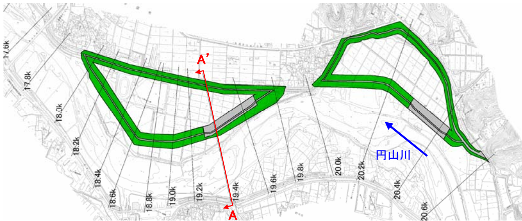
図 4.1.7 遊水地平面図
