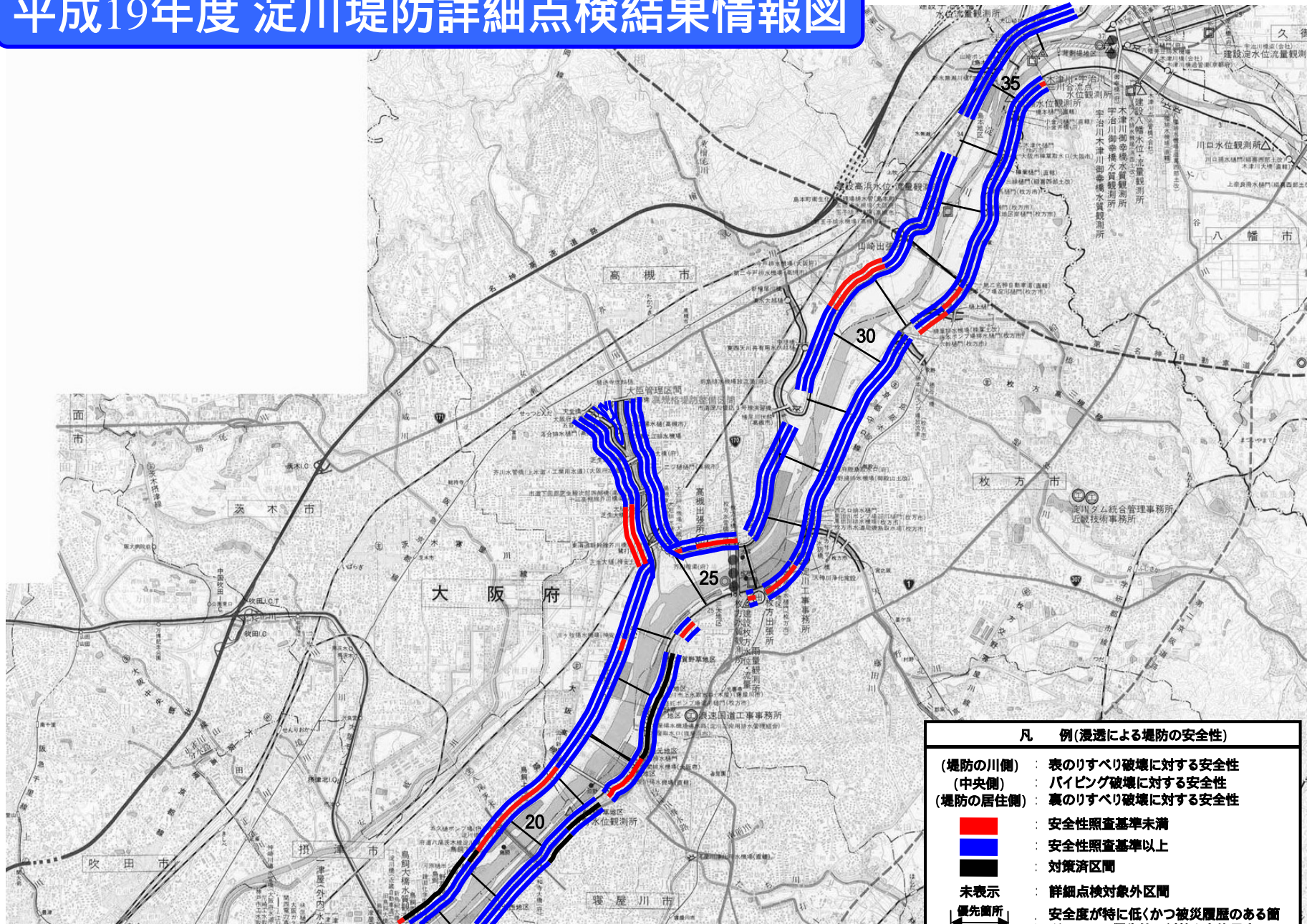
浸透に対する詳細点検結果 淀川(2)
