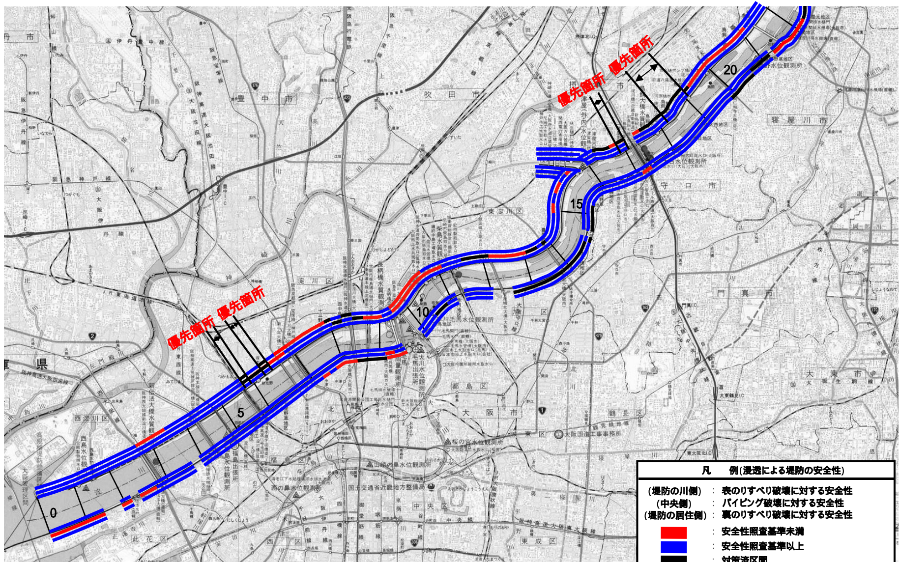
浸透に対する詳細点検結果 淀川(1)
