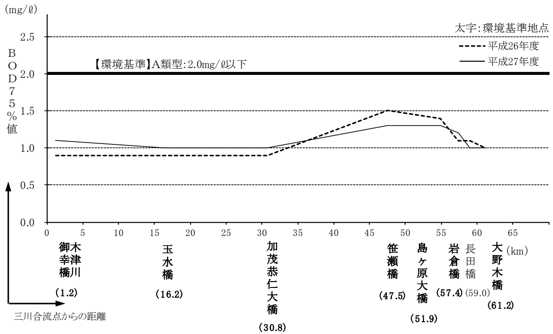
図-1.42 木津川の水質縦断面図（BOD75%値）
