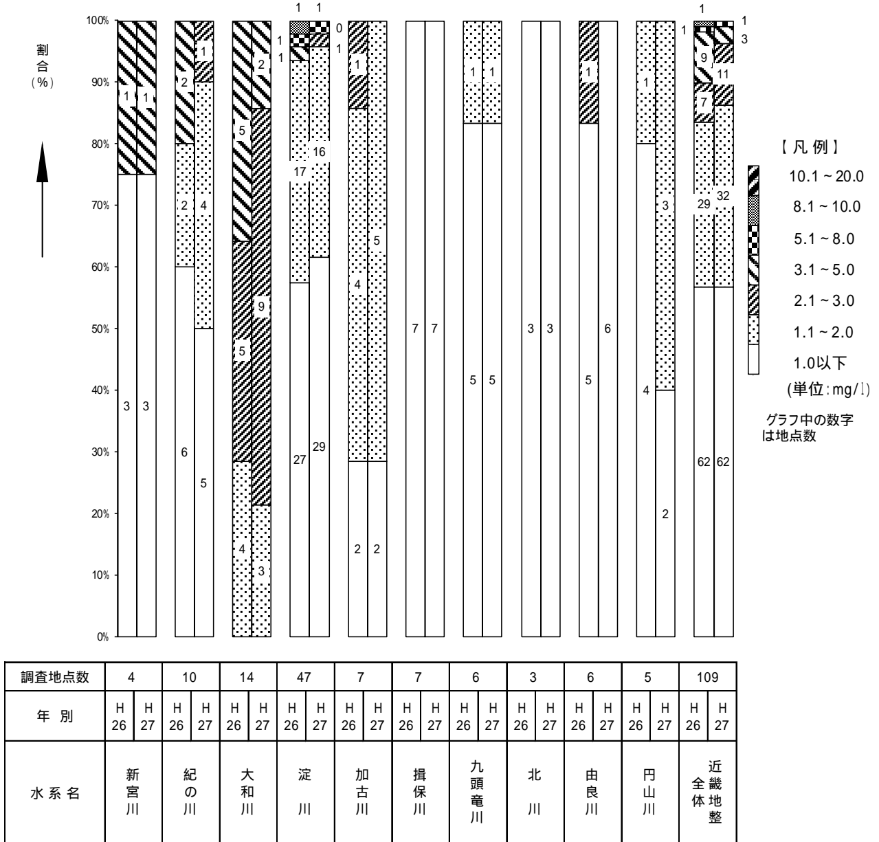
図 - 1.6 水系別BOD75%値のランク別割合（平成26年 109地点，平成27年 109地点）
