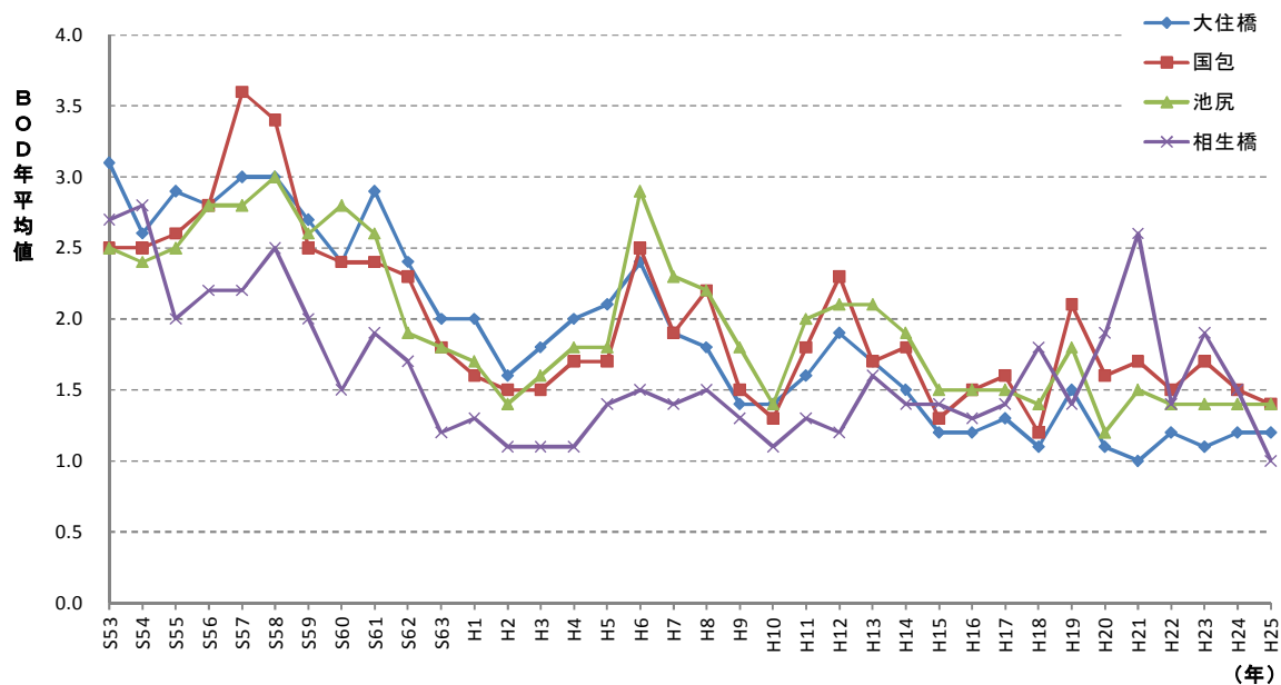
図-1.23 加古川の水質経年変化 (BOD年平均値)
