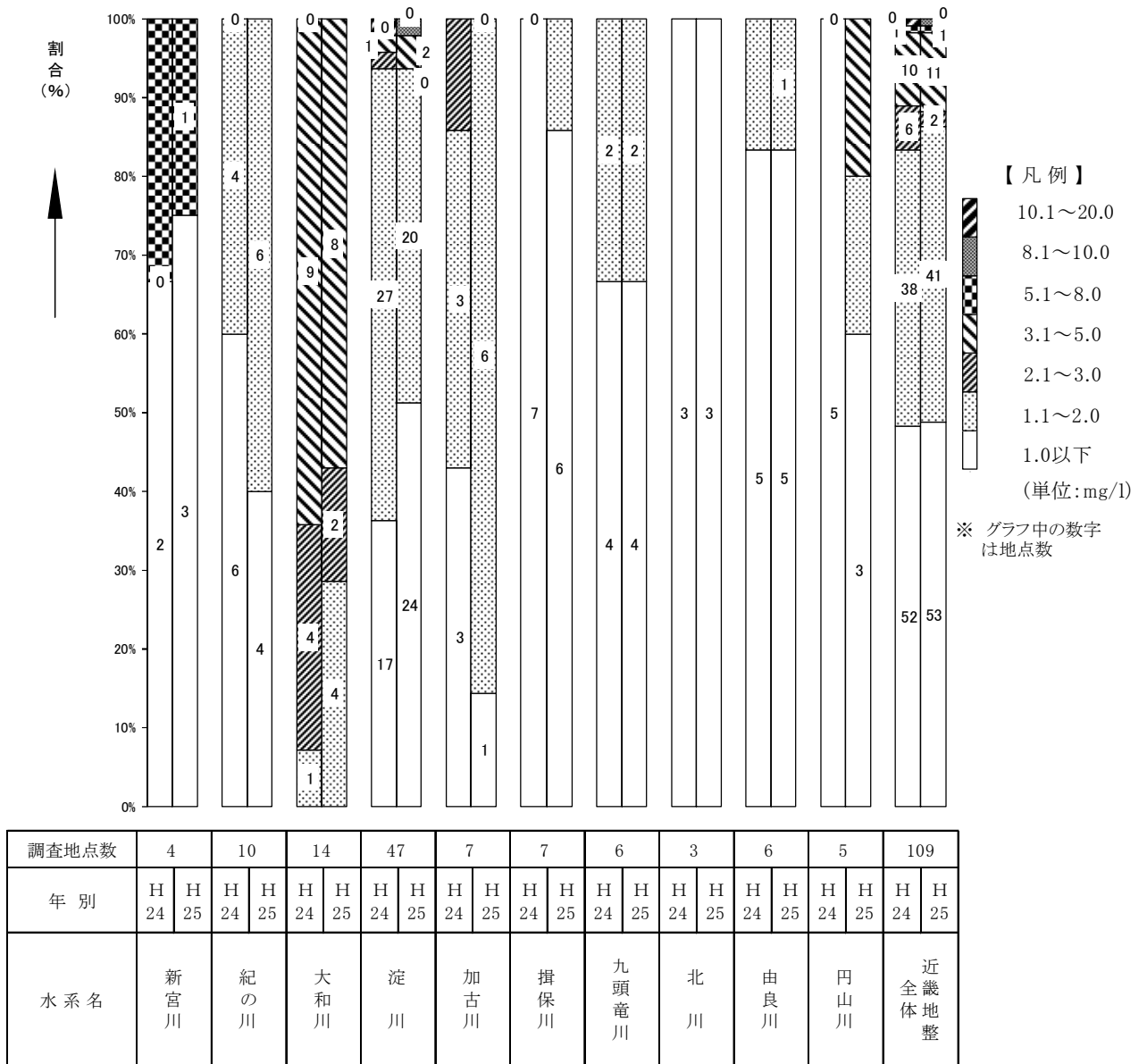
図-1.6 水系別BOD75%値のランク別割合（平成24年 108地点，平成25年 109地点）
