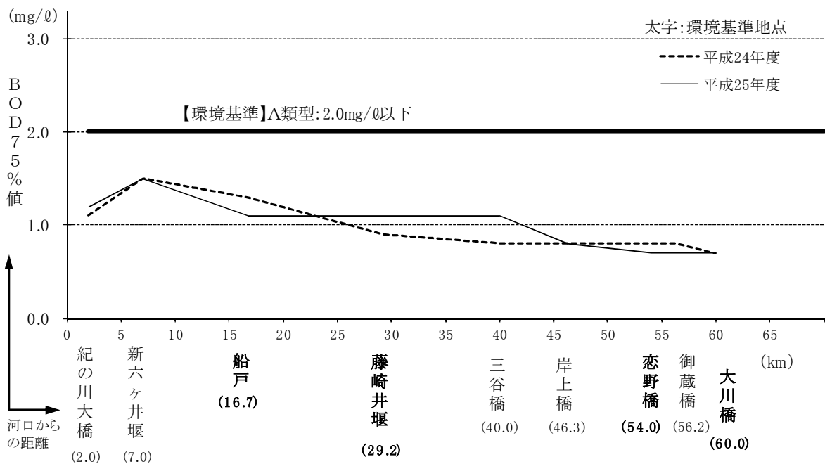
図-1.33 紀の川の水質縦断図（BOD75%値）
