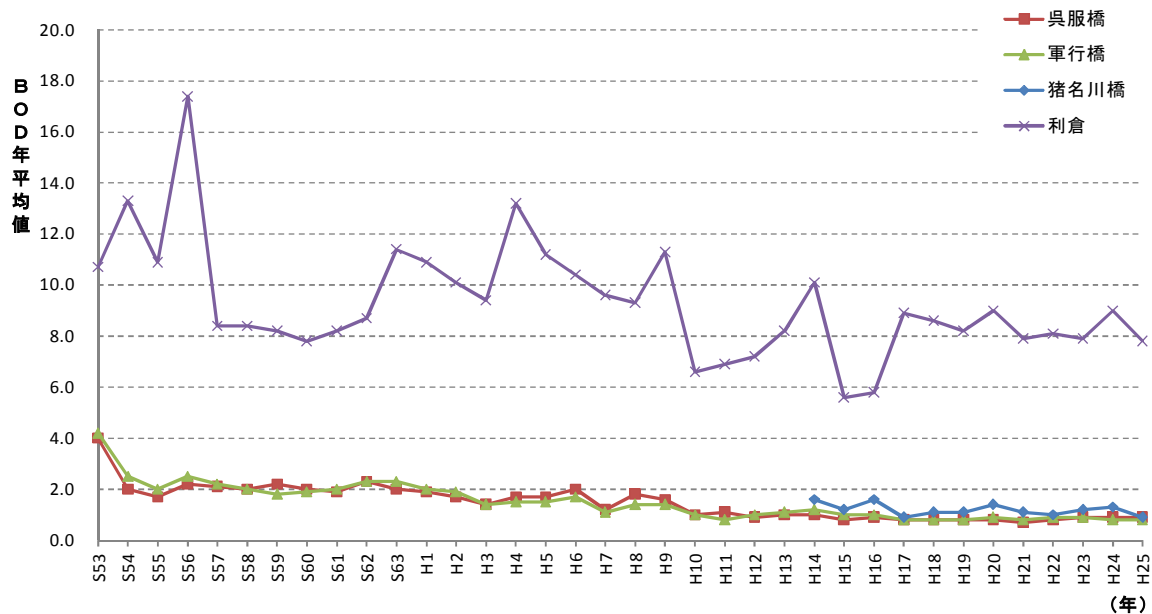
図-1.22 猪名川の水質経年変化 (BOD年平均値)
