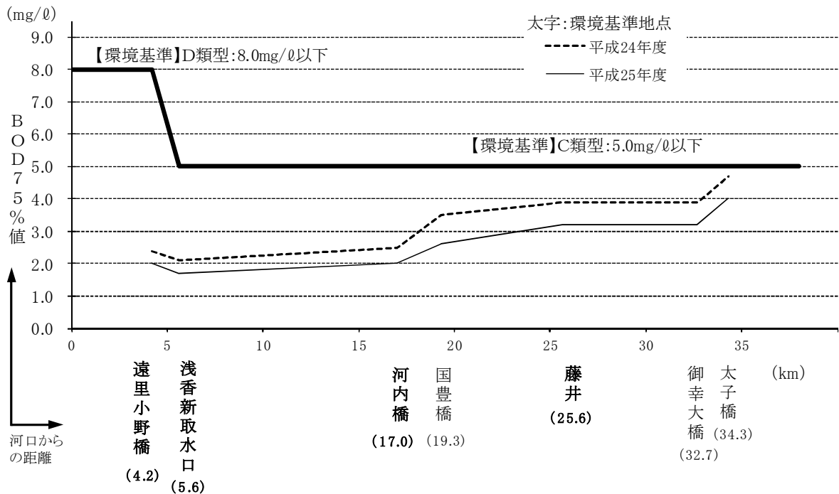
図-1.35 大和川の水質縦断面図（BOD75%値）
