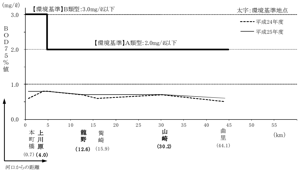
図-1.48 揖保川の水質縦断面図（BOD75%値）
