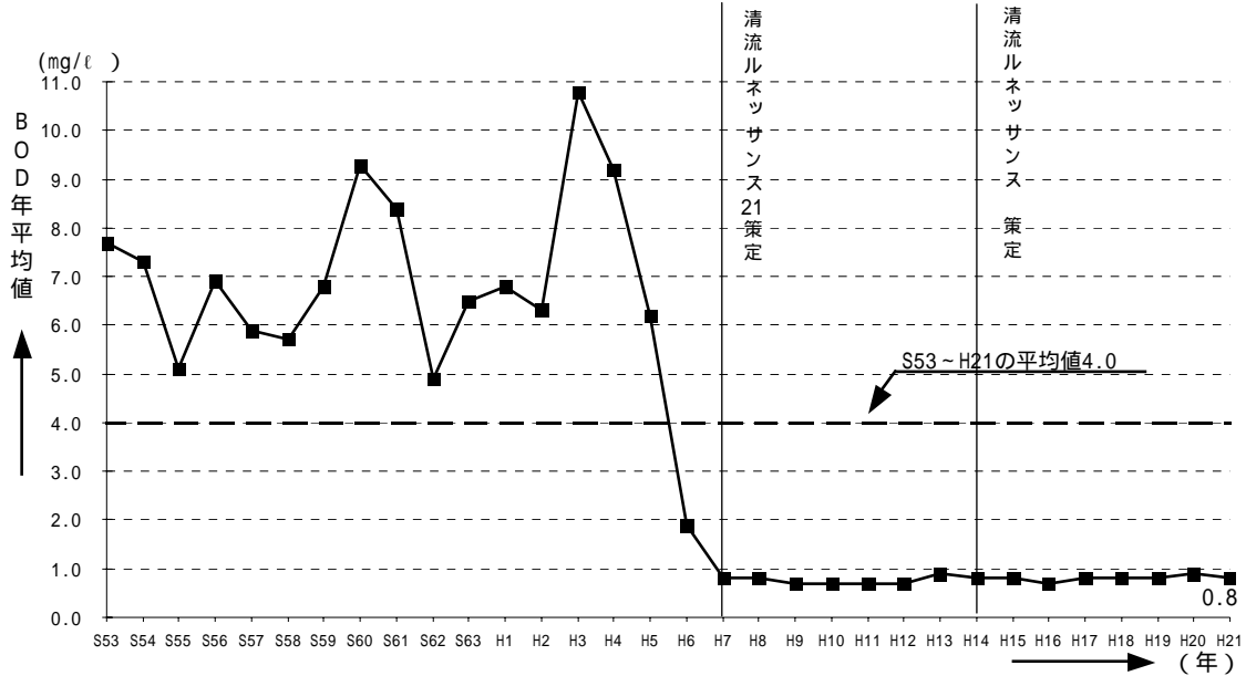
図 - 4.22 揖保川の水質経年変化（BOD年平均値）
