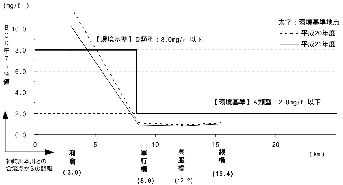
図 - 4.43 猪名川の水質縦断図（BOD75%値）
