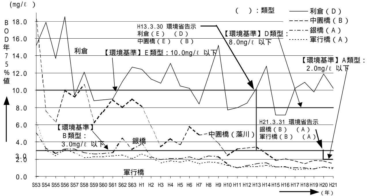
図 - 4.42 淀川水系（猪名川、藻川）の環境基準地点の水質経年変化（BOD75%値）
