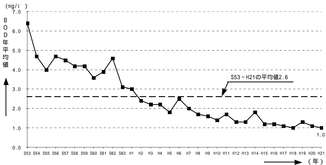
図 - 4.16 桂川の水質経年変化 (BOD年平均値)
