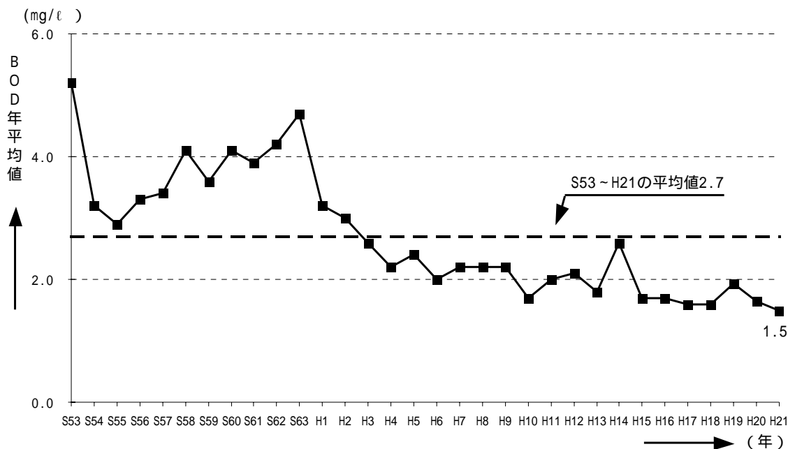
図 - 4.13 淀川本川（三川合流点下流： ひらかたおおはし 枚方大橋・ とりかいおおはし 鳥飼大橋・ くにしま 柴島・ でんぼうおおはし 伝法大橋）平均水質の経年変化
