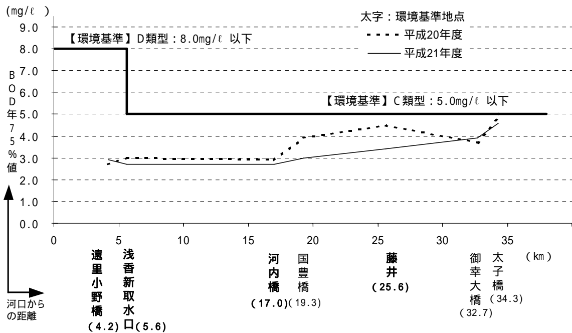
図 - 4.34 大和川の水質縦断図（BOD75%値）
