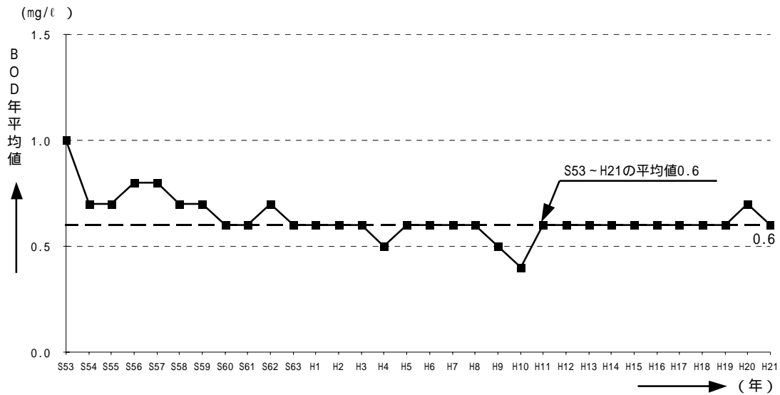
図 - 4.26 北川の水質経年変化 (BOD年平均值)
