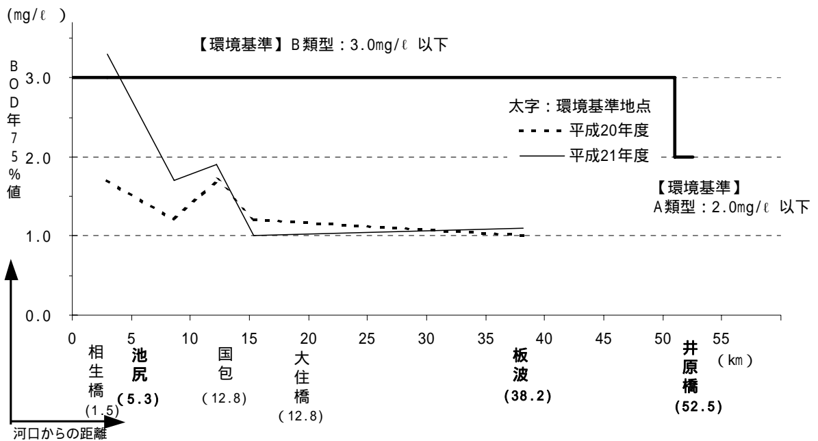
図 - 4.45 加古川の水質縦断図（BOD75%値）
