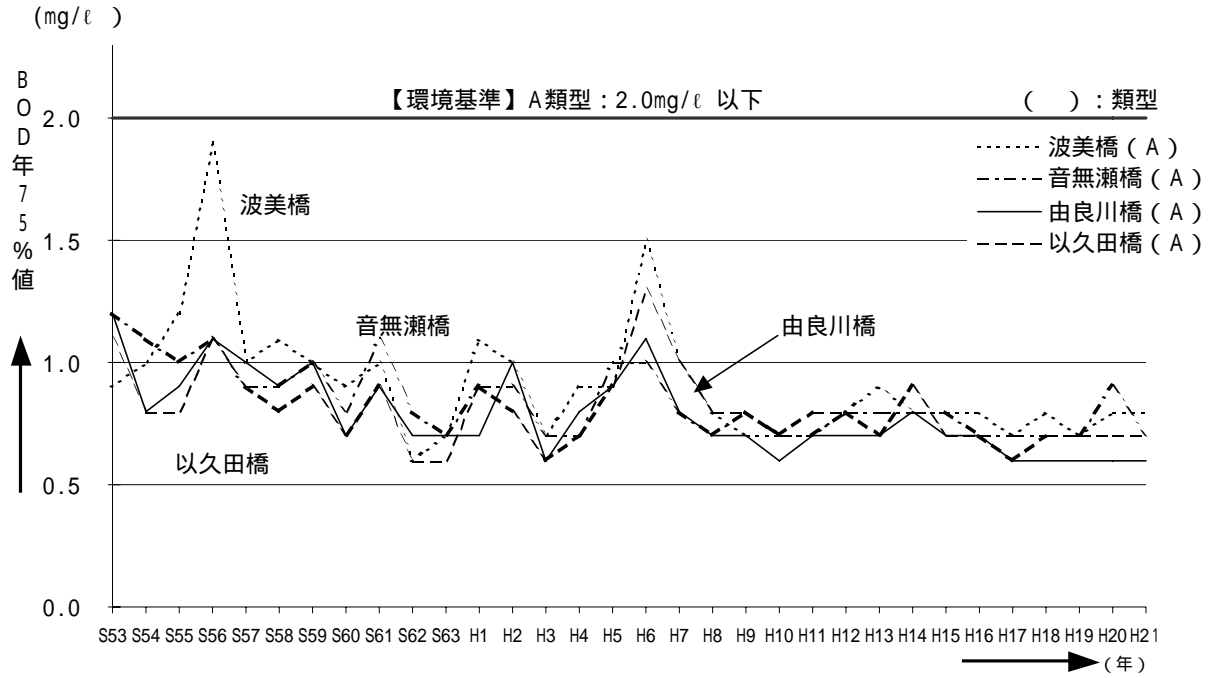
図 - 4.52 由良川水系（由良川）の環境基準地点の水質経年変化（BOD75%値）
