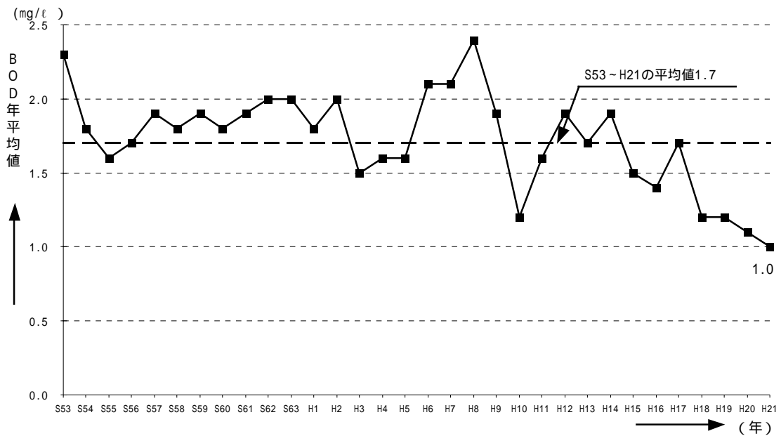
図 - 4.19 木津川の水質経年変化 (BOD年平均值)
