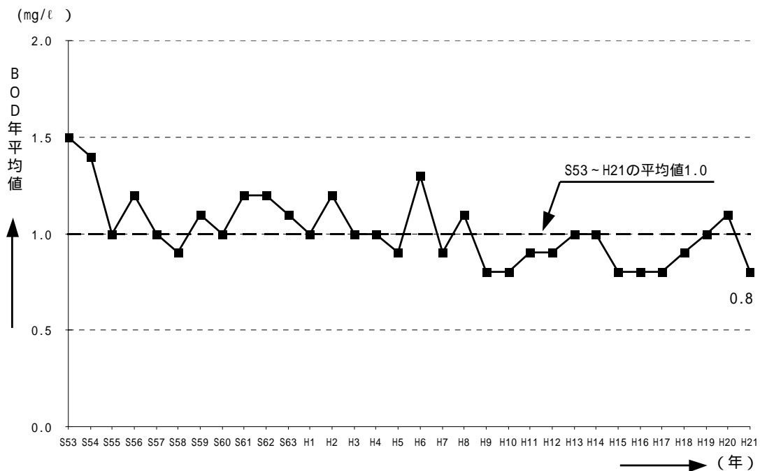
図 - 4.27 九頭竜川の水質経年変化 (BOD年平均值)
