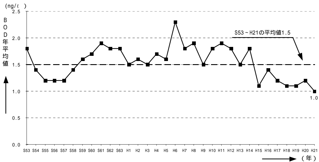
図 - 4.10 紀の川の水質経年変化 (BOD年平均值)
