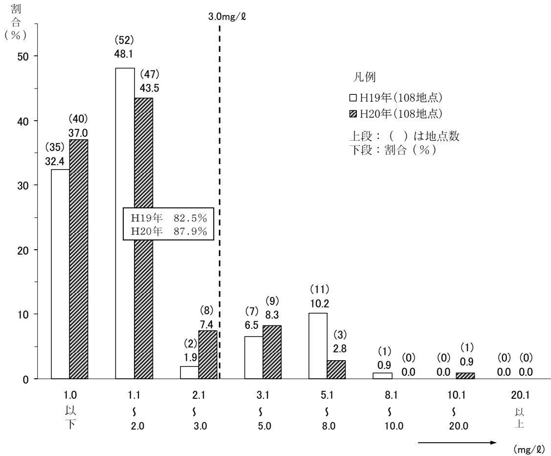
図-1.2 一級河川におけるBOD 75%値ランク別割合 (平成 19 年、平成 20 年とも河川 108 地点での評価)
