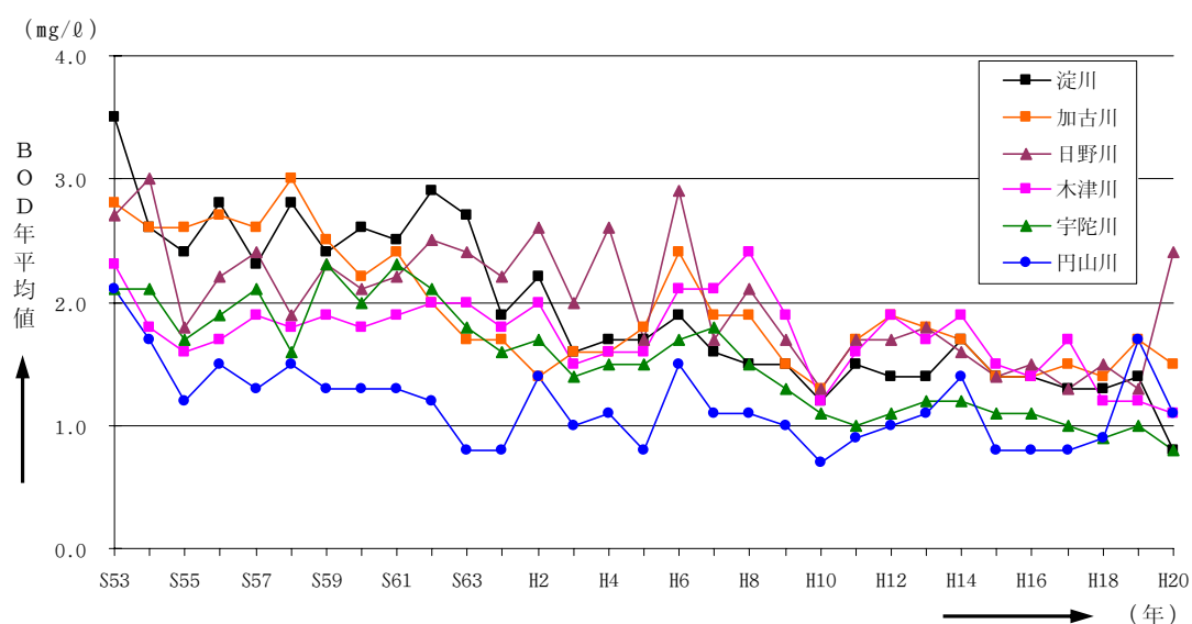
図一.4 主要河川水質の経年変化 (2) (BOD年平均値)
