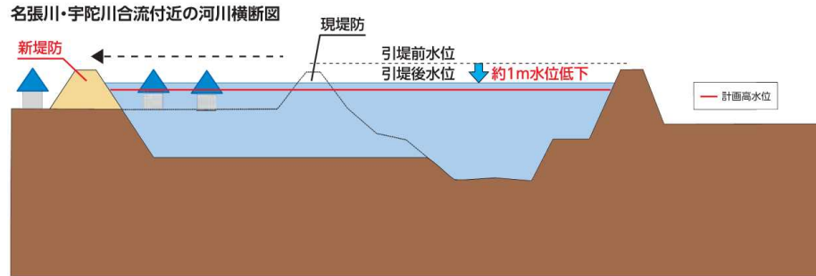
全体事業の実施効果 昭和28年台風13号洪水に対する効果
