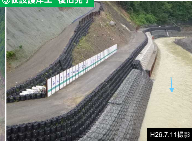
③仮設護岸工 復旧完了
