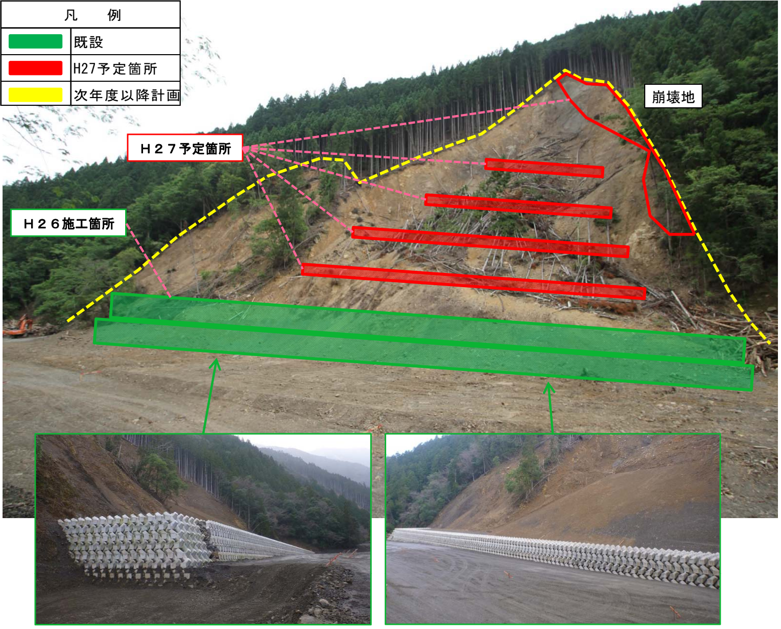
コンクリートブロック護岸工 施工状況
