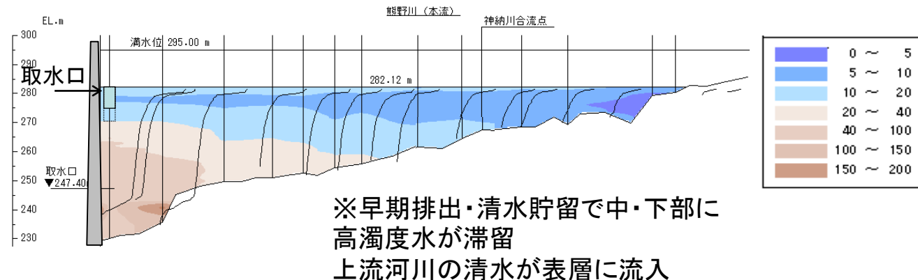
風屋貯水池縦断 濁度分布状況(8/17 9:00)
