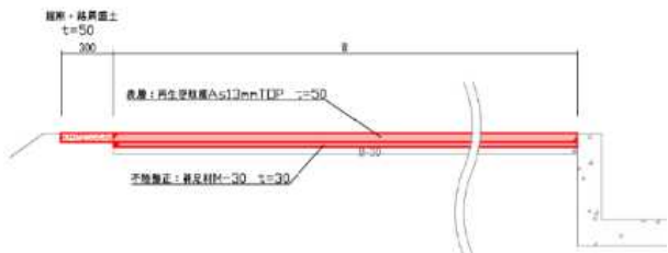
標準断面図
