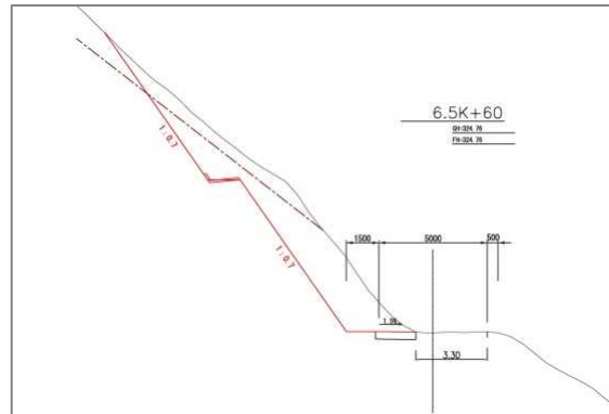
標準断面図 ②
