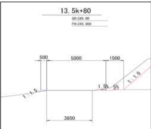
⑦ 標準断面図①-2
