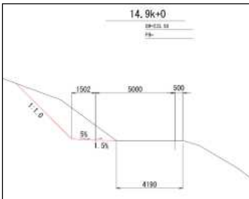
標準断面図①-6
