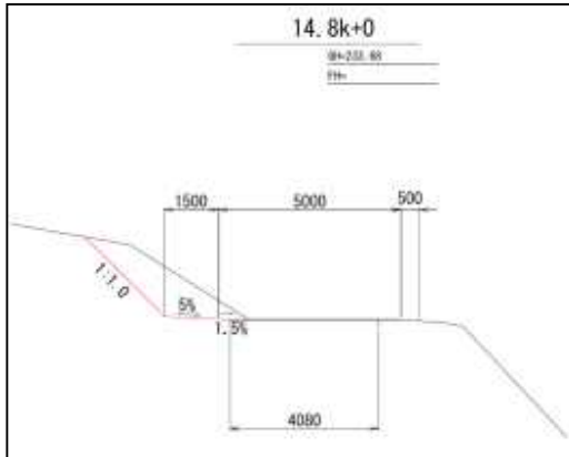
標準断面図①-5
