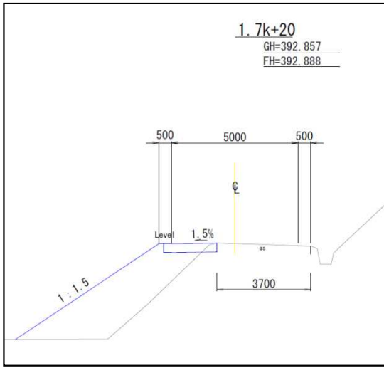
標準断面図 ①
