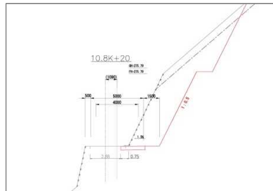
標準断面図 ⑤
