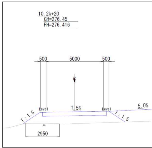
標準断面図 ④
