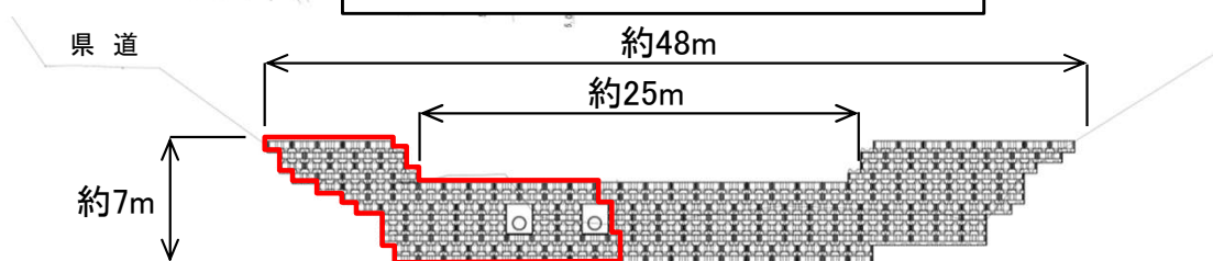
整備内容(横断図)＜上流面＞
