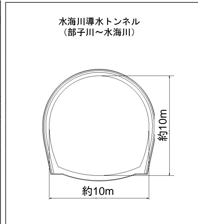
導水トンネル 断面図
