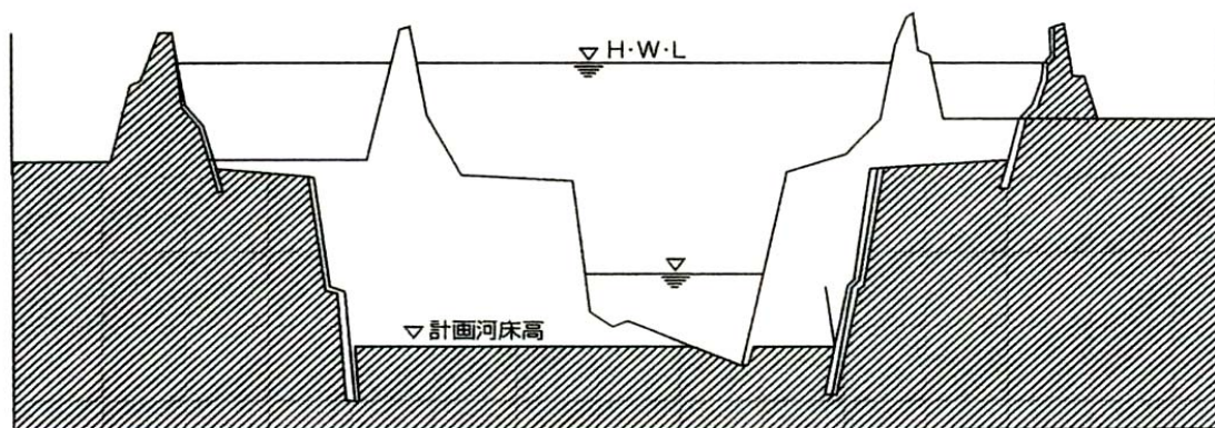
計画横断図
