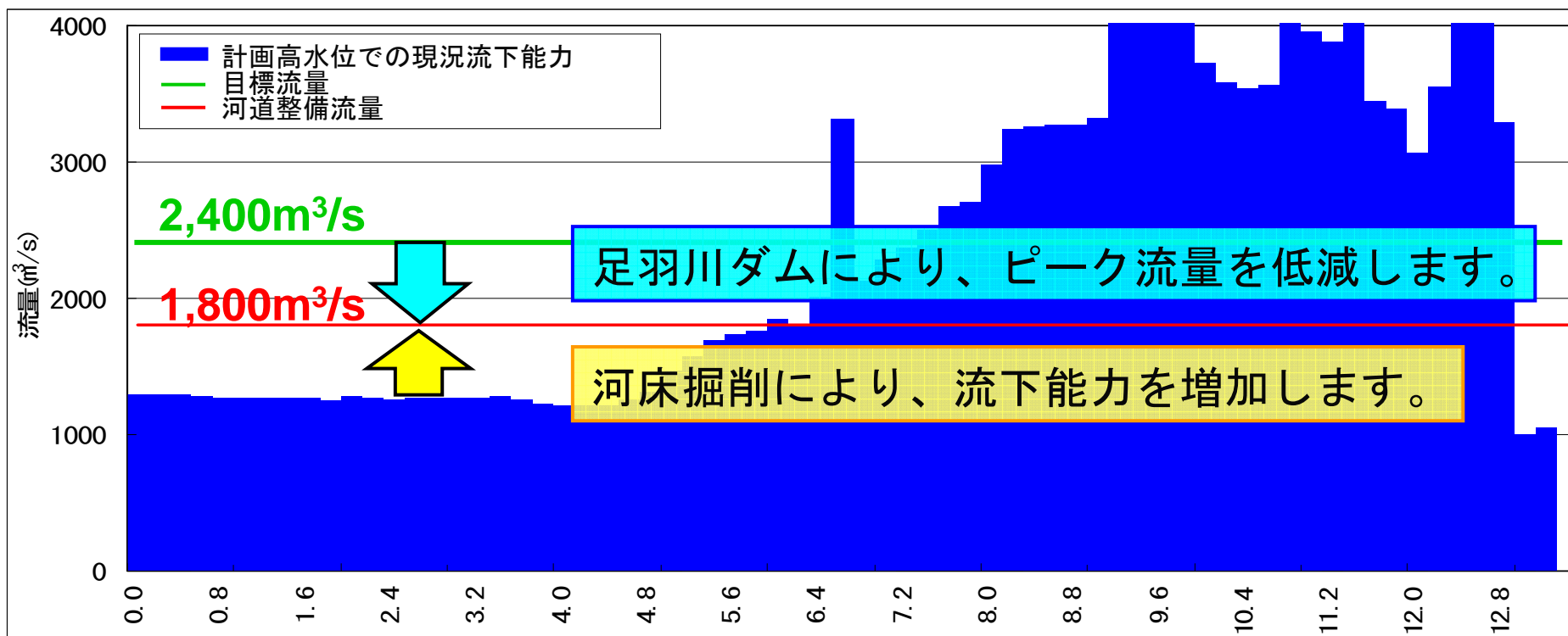
現況河道の流下能力図 (河川整備計画策定時)
