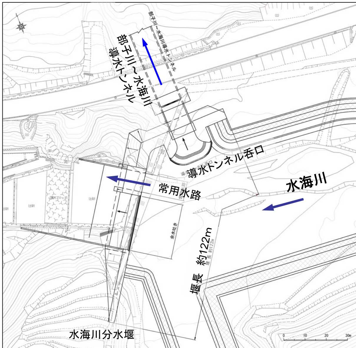
分水堰 平面図
