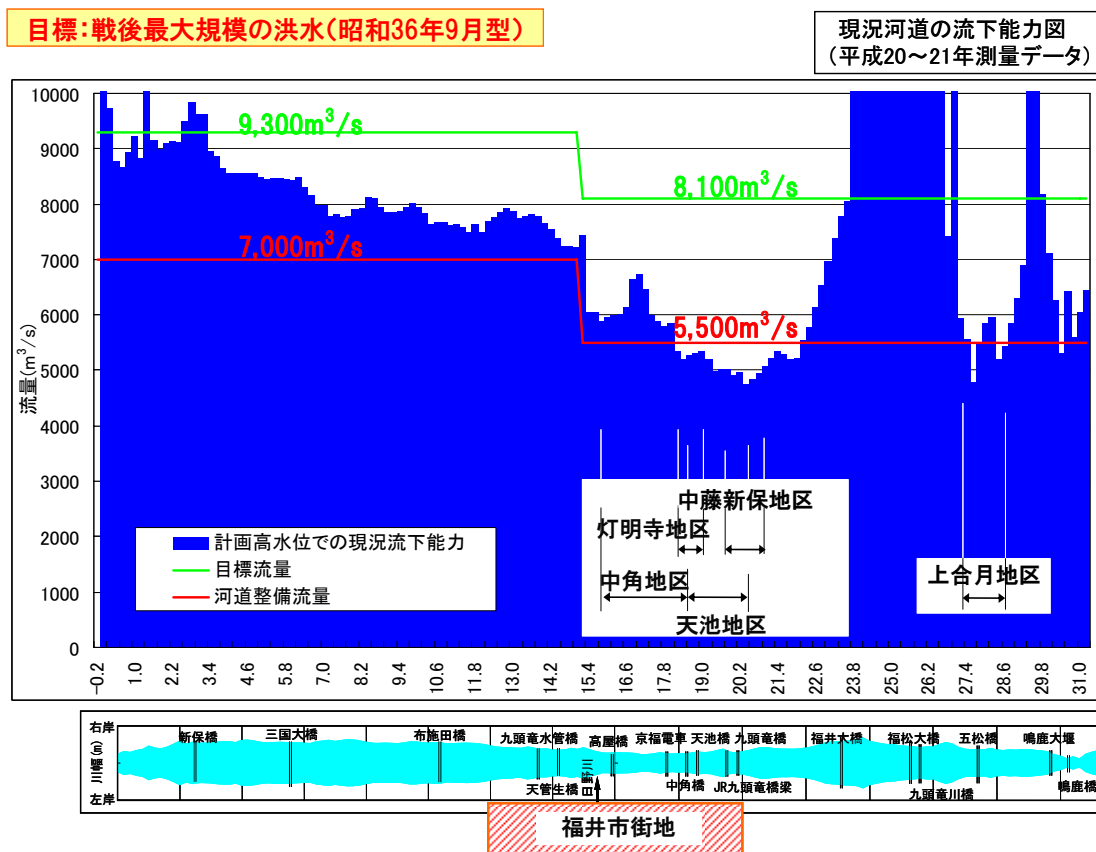
図 2-27 流下能力図（九頭竜川）
