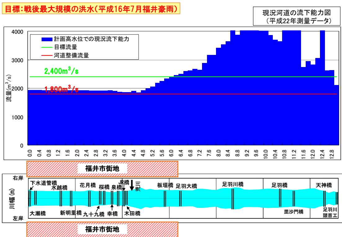
図 2-29 流下能力図（足羽川）
