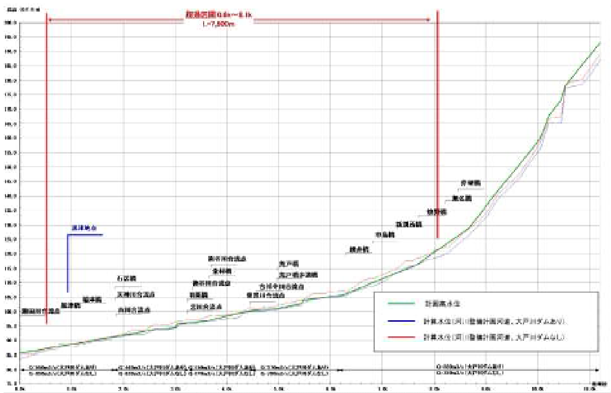
図 4.2-2 河川水位縦断面図（大戸川滋賀県管理区間）
