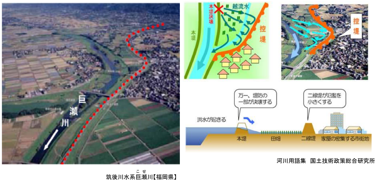
巨瀬川二線堤(控堤) (福岡県久留米市)
