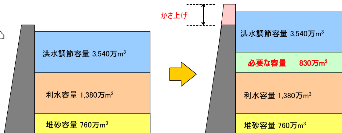
高山ダム かさ上げ イメージ図
