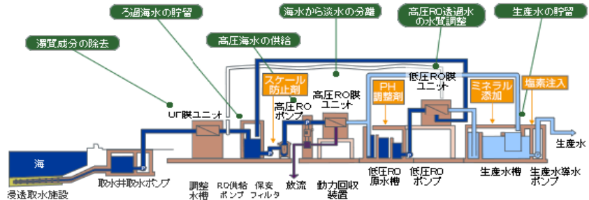
海水淡水化施設イメージ図
