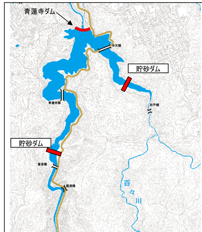
青蓮寺ダム 貯砂ダム候補地
