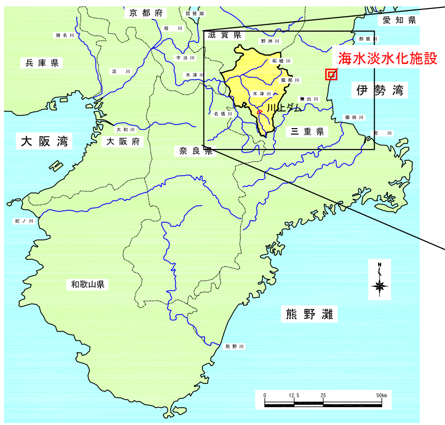
海水淡水化施設および想定導水路ルート位置図
