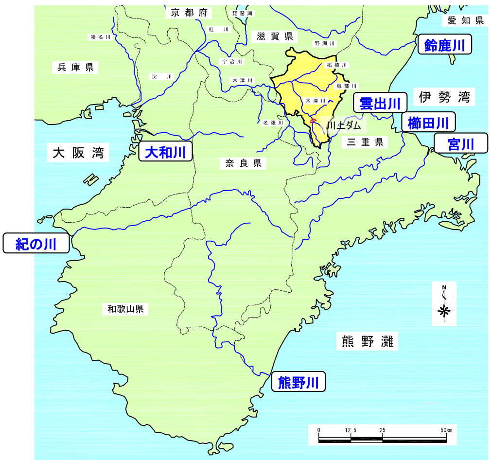
水系間導水候補水系位置図
