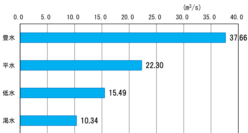
図 1.3.4-1 大河原地点における流況（至近10カ年平均）
