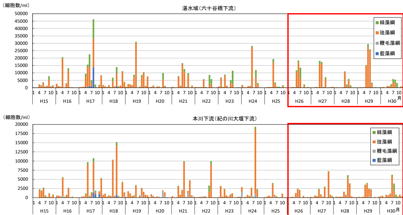
図 5.3-19 各地点における植物プランクトン細胞数の推移 (H15～H30)
