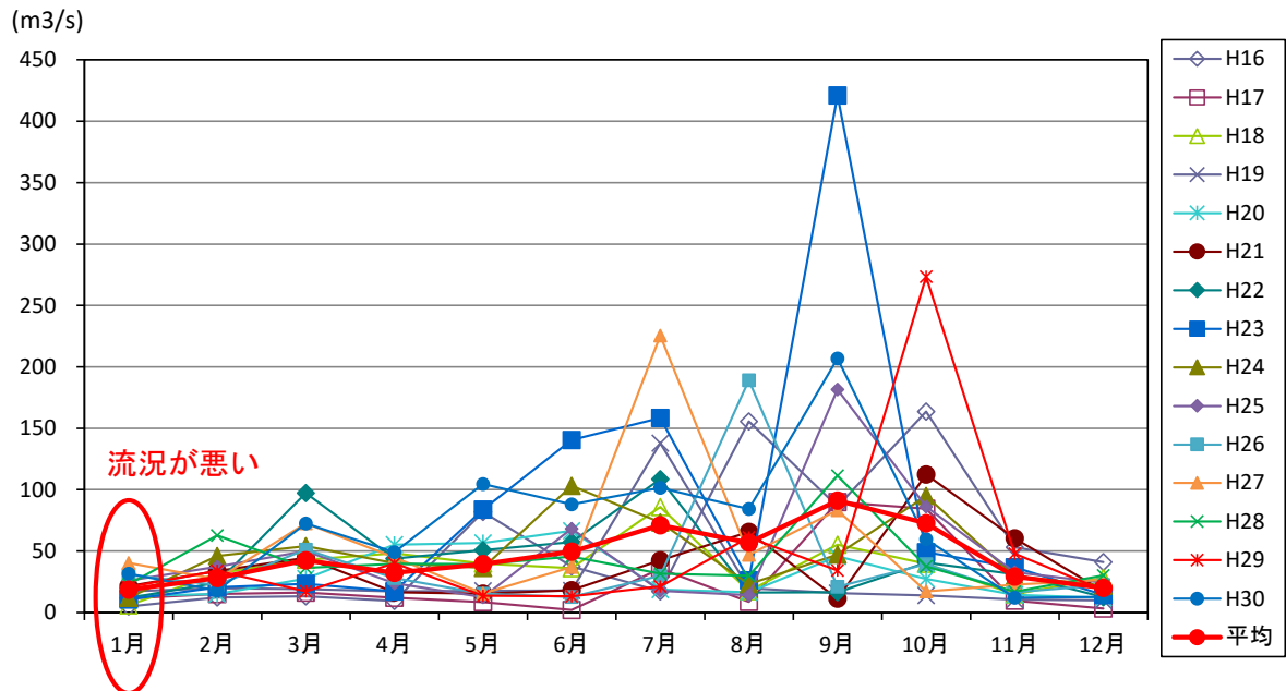
図 5.5-27 月平均放流量 (H16~H30)
