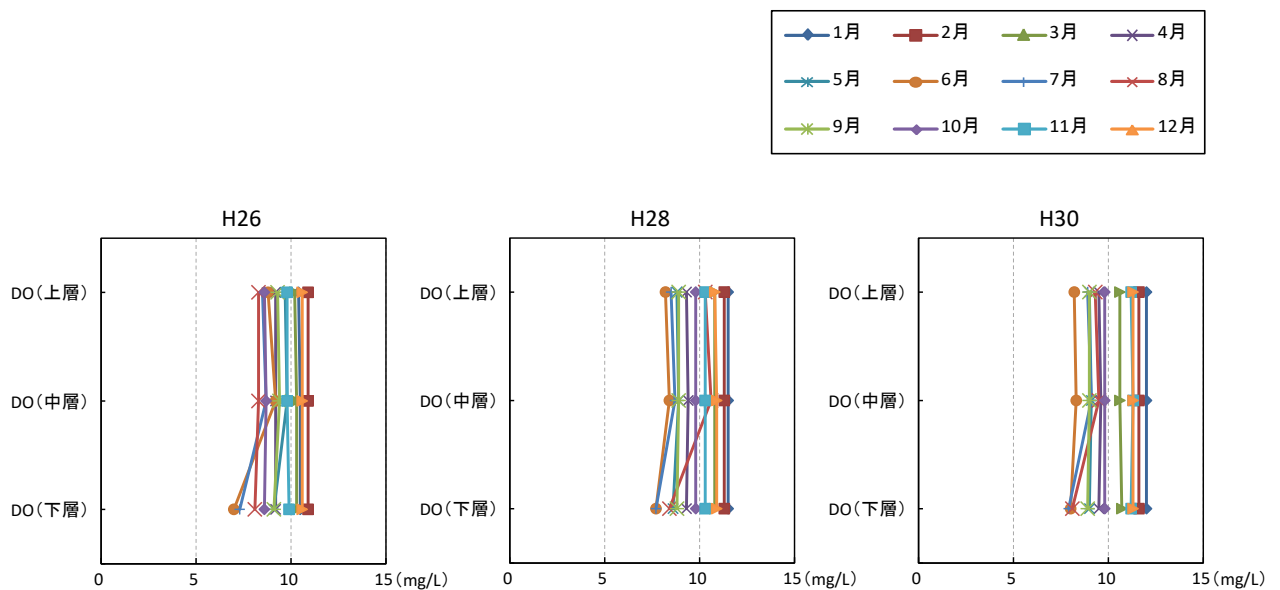
図 5.5-9 (2) 紀の川大堰直上地点の DO の鉛直分布
