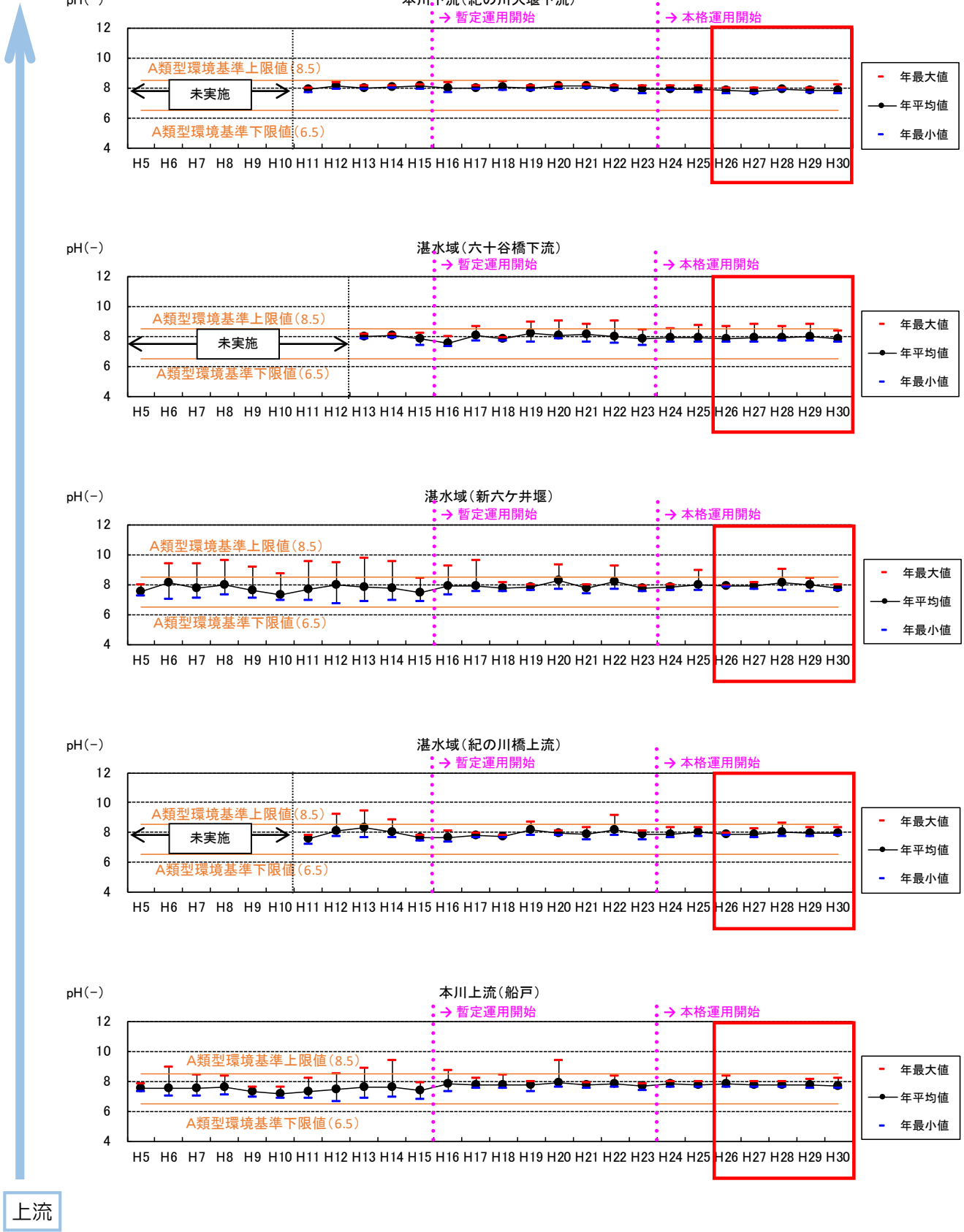
図 5.3-9 (2) 調査地点ごとの pH 年平均値の経年変化
