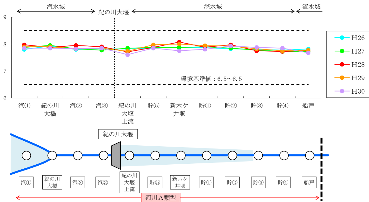
図 5.5-20 年平均pHの縦断変化
