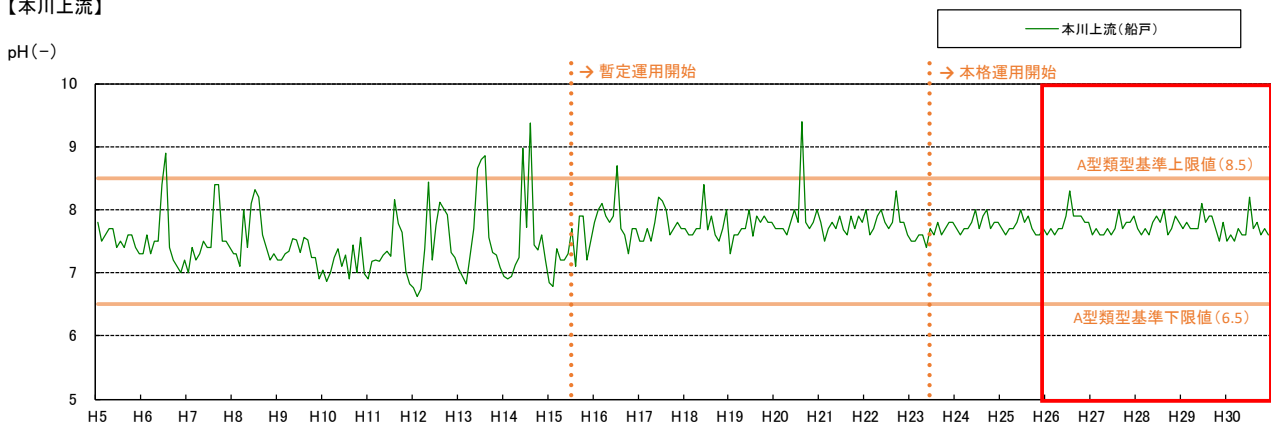
図 5.3-11 (2) 調査地点ごとの pH の経月変化 (H5~H30)
