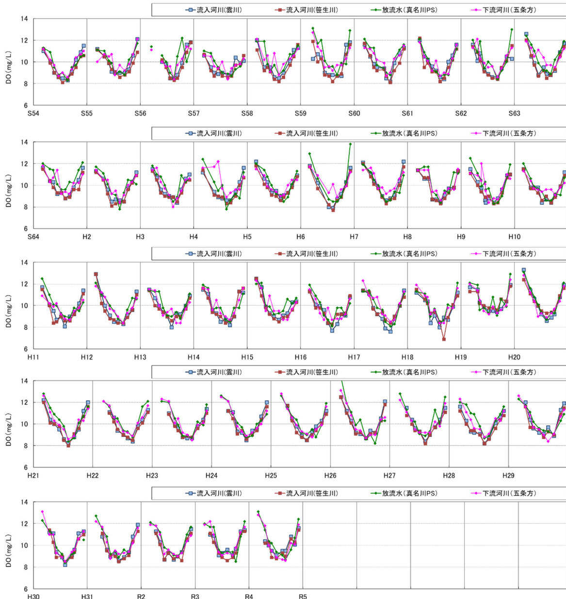
図 5.5-21 流入DO、放流DOの推移
