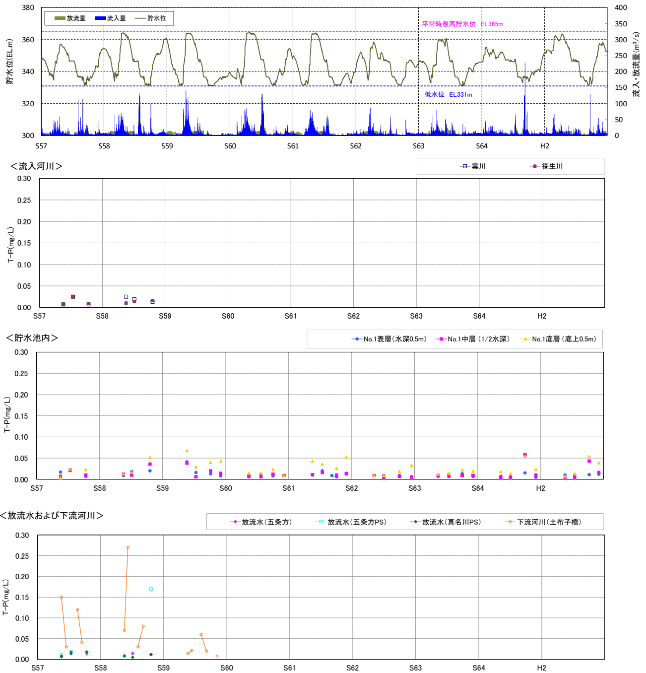
図 5.3-18(2) 流入河川、貯水池内、放流水及び下流河川の水質の経月変化 (T-P : S57~H2)
