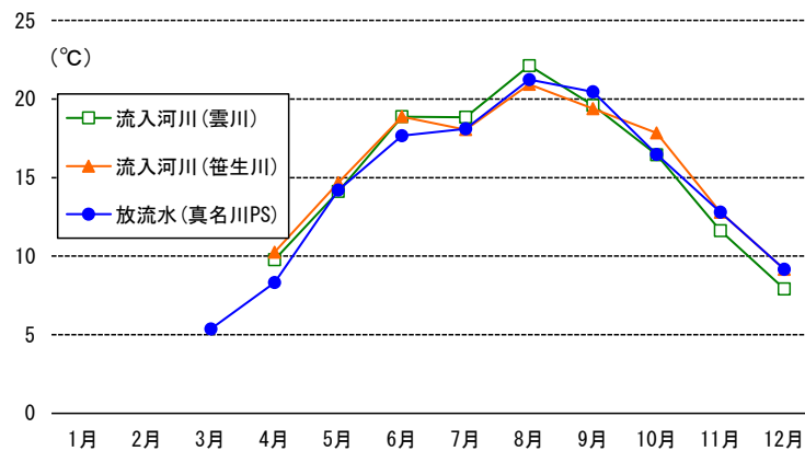
図 5.5-10 流入河川・放流水の月別平均水温 (H30~R4)
