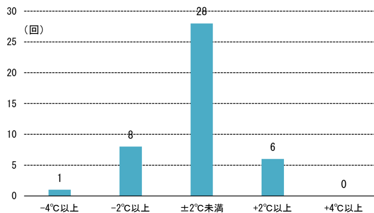
図 5.5-11 「放流水-流入河川」の水温差比較 (H30~R4)
