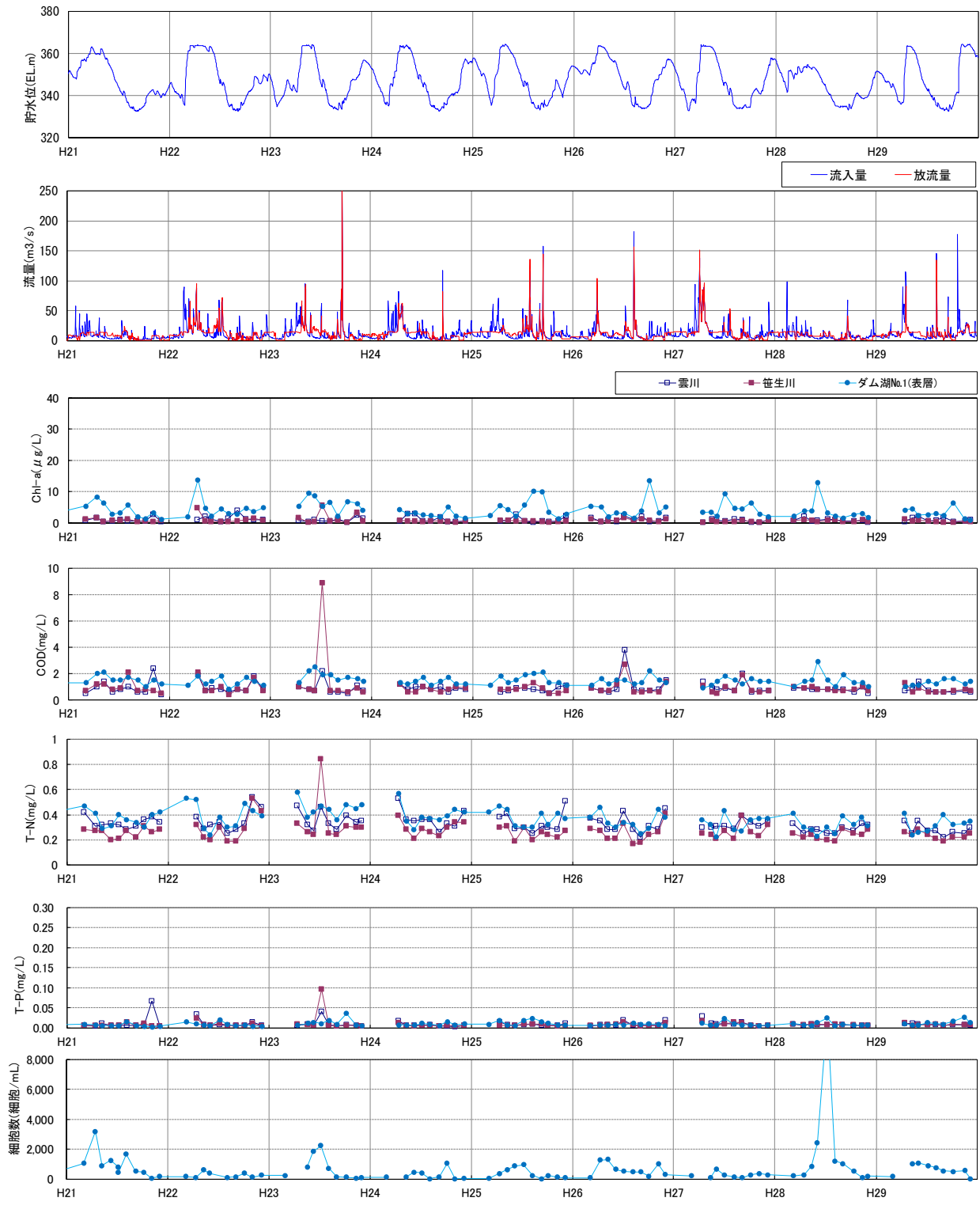
図 5.5-18 (4) 富栄養化評価関連項目の経月変化 (H21~H29) 【出典：平成30年度 真名川ダム定期報告書 平成31年3月】 【出典：水質調査業務報告書(真名川ダム)・データ 平成30年~令和4年】
