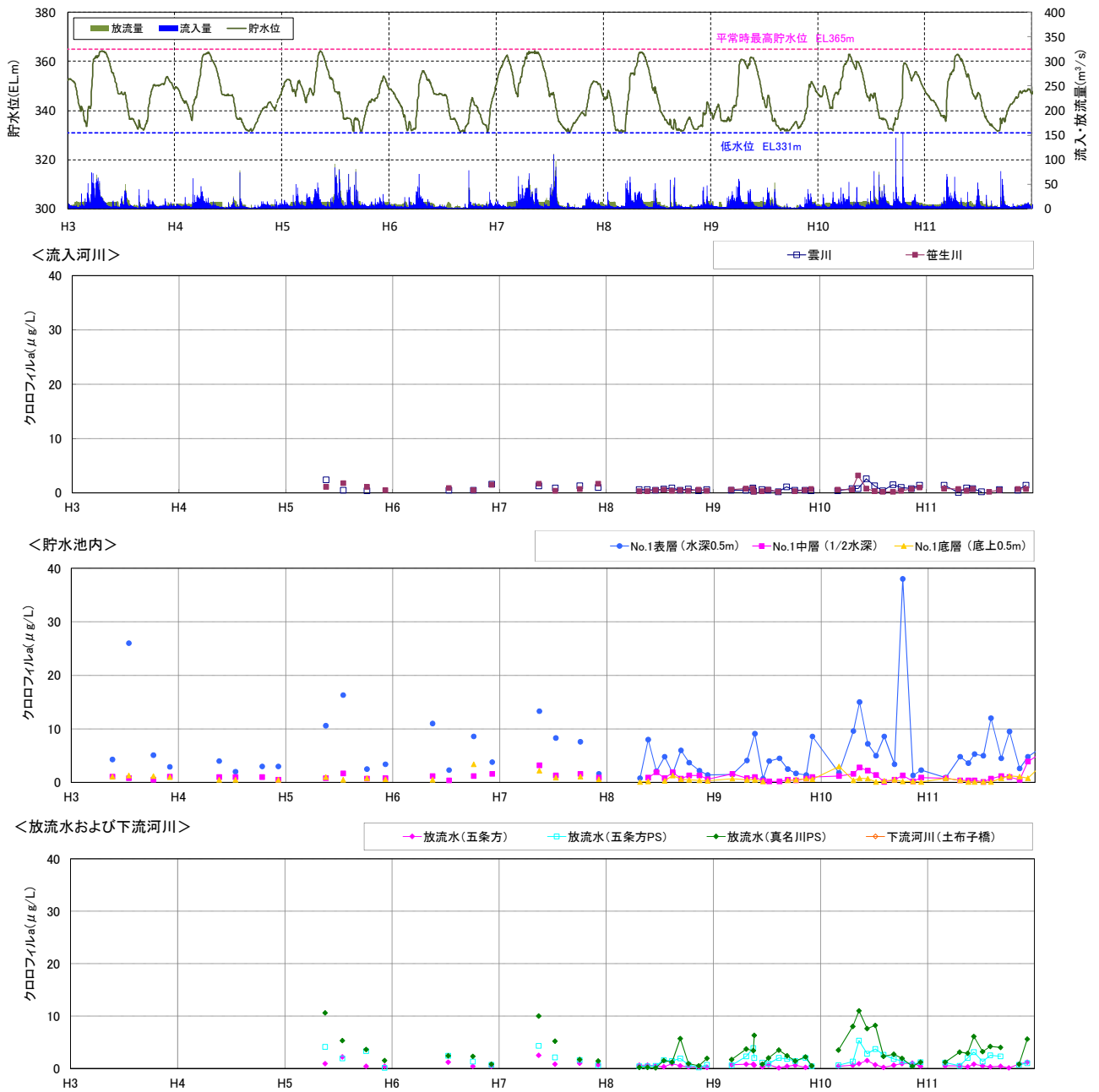
図 5.3-19(3) 流入河川、貯水池内、放流水及び下流河川の水質の経月変化 (クロロフィルa : H3~H11)
