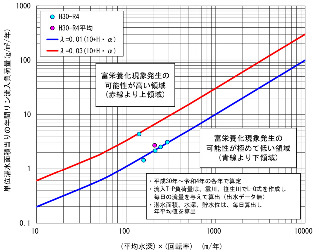
図 5.5-19 Vollenweiderモデルによる真名川ダム富栄養化評価
