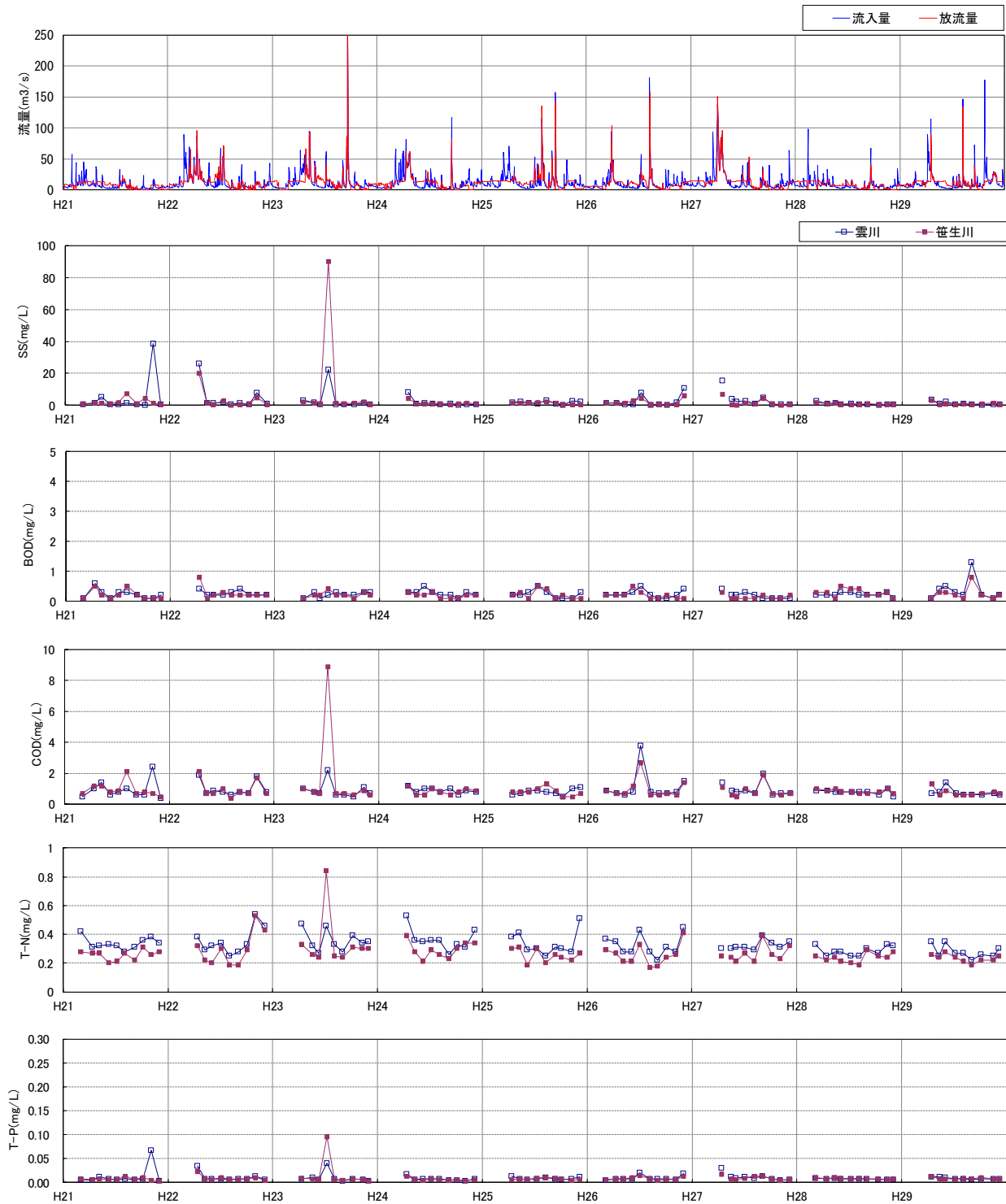
図 5.4-6(4) 真名川ダム流入水質の状況(H21~H29)
