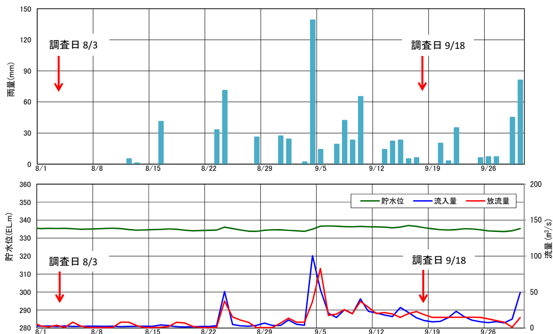
図 5.3-22 平成30年8月、9月調査日周辺の雨量及び貯水池運用図
