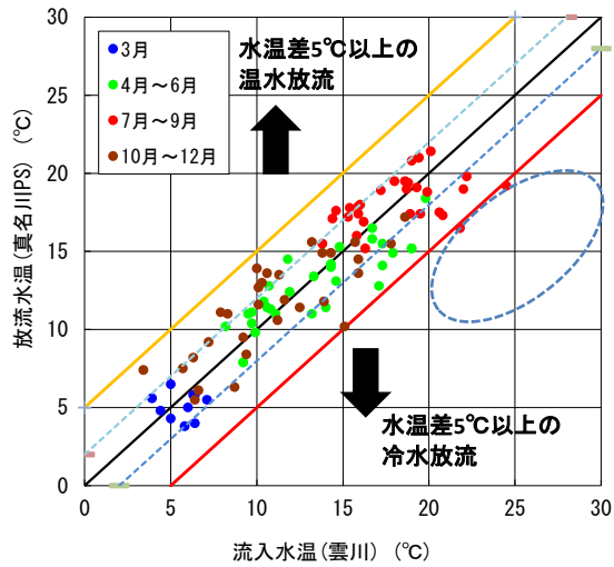
図 5.5-9(3) 流入・放流水温の比較(S63~H9)
