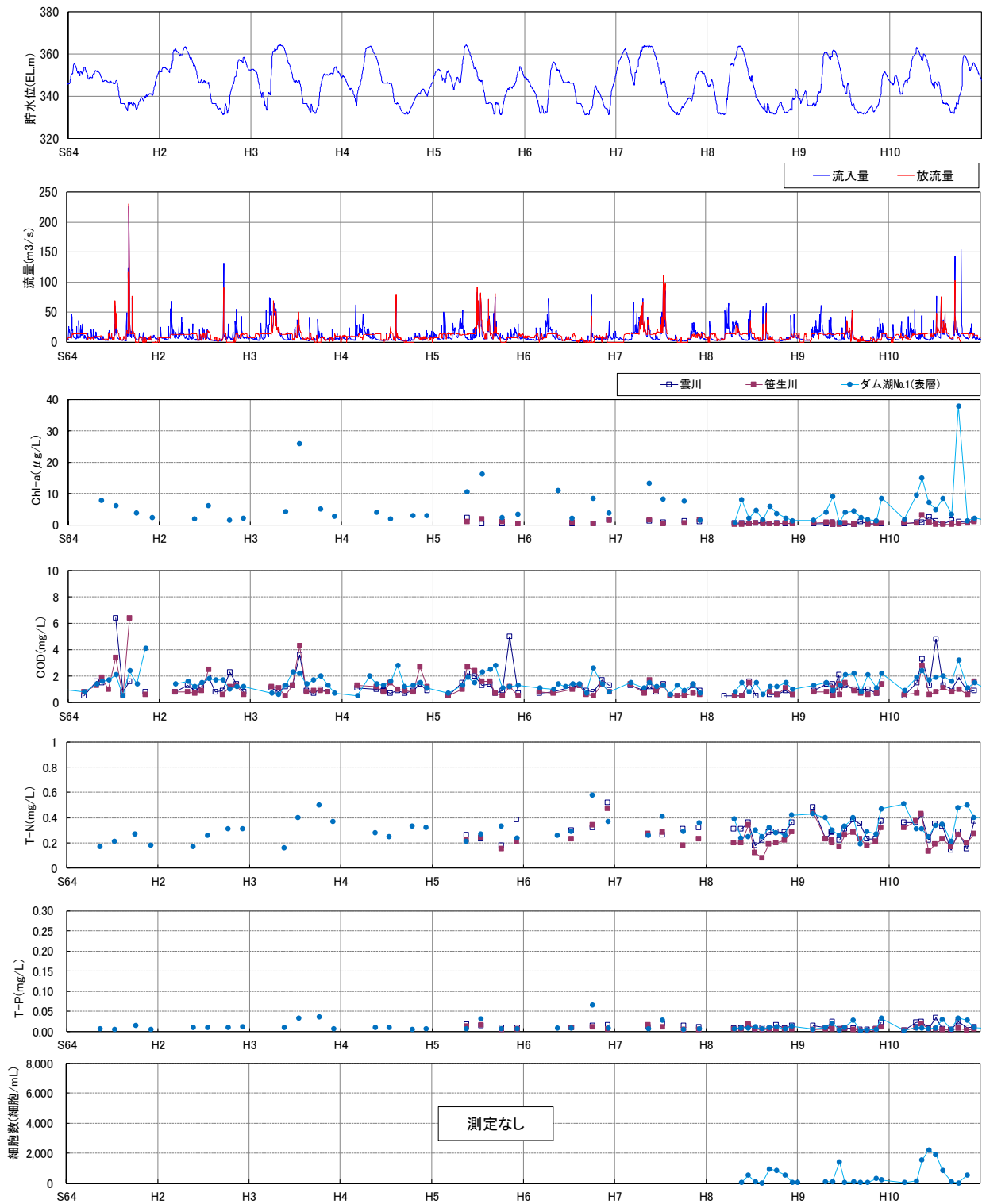
図 5.5-18 (2) 富栄養化評価関連項目の経月変化 (S64~H10) 【出典 : 平成 30 年度 真名川ダム定期報告書 平成 31 年 3 月】 【出典 : 水質調査業務報告書(真名川ダム)・データ 平成 30 年~令和 4 年】
