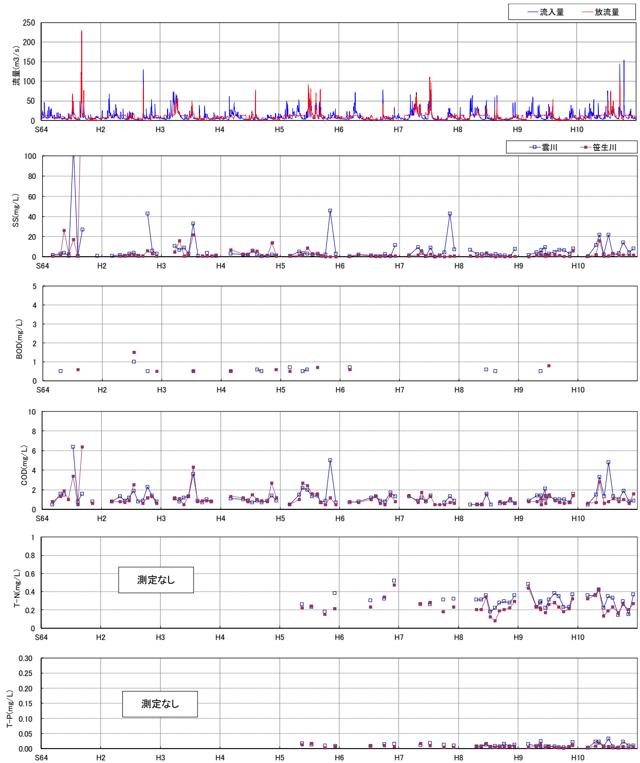
図 5.4-6 (2) 真名川ダム流入水質の状況 (S64~H10)
