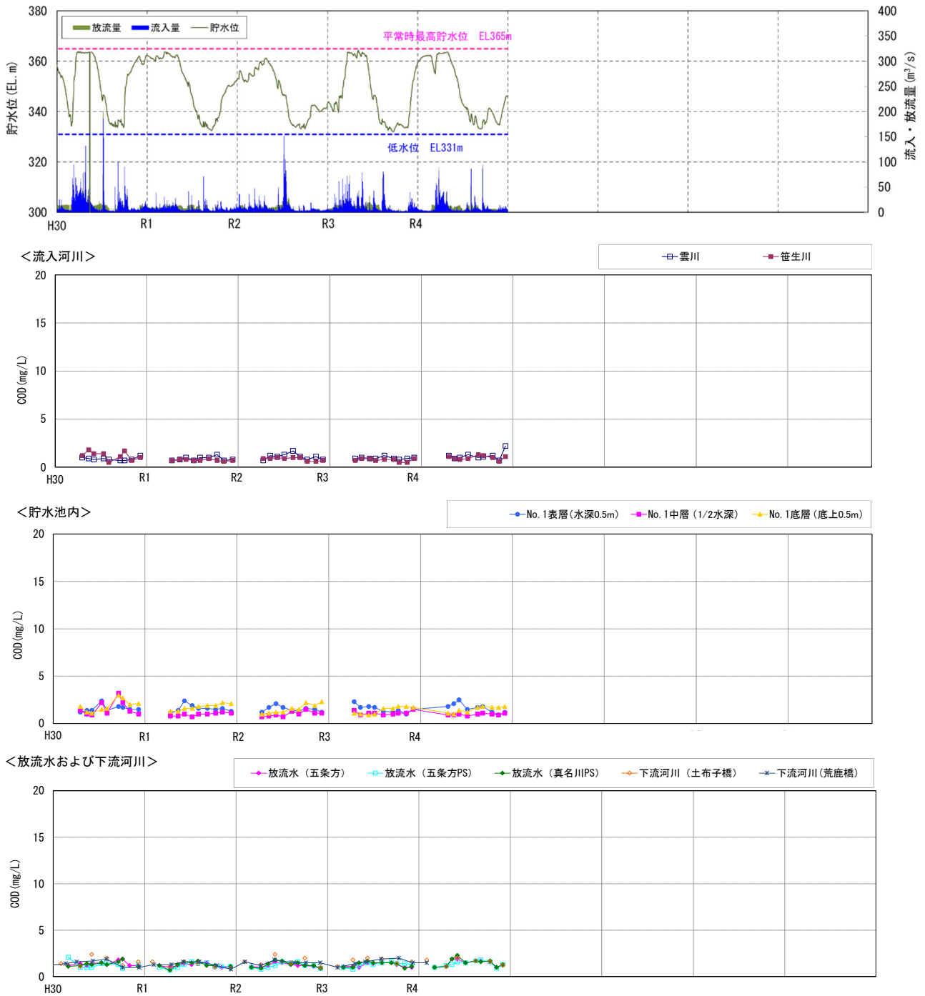
図 5.3-16(6) 流入河川、貯水池内、放流水及び下流河川の水質の経月変化 (COD : H30~R4)
