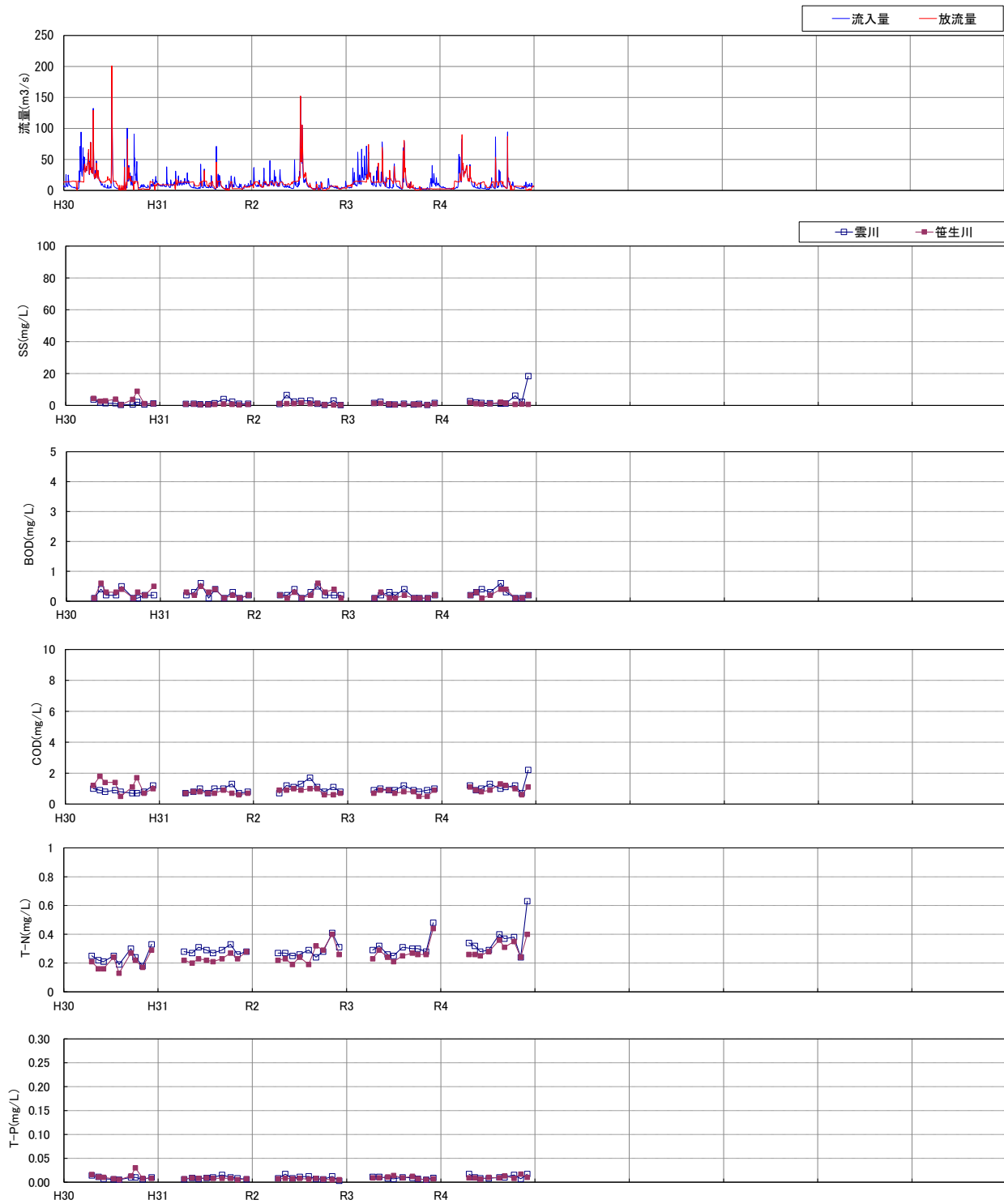
図 5.4-6(5) 真名川ダム流入水質の状況 (H30~R4)
