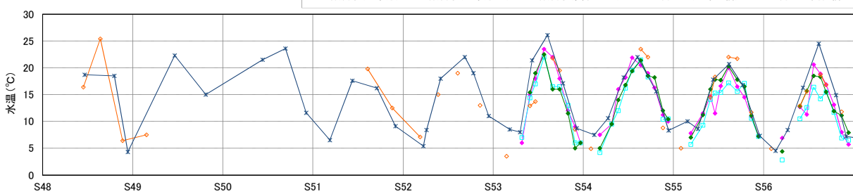
図 5.3-11(1) 流入河川、貯水池内、放流水及び下流河川の水質の経月変化 (水温：S48～S56)
