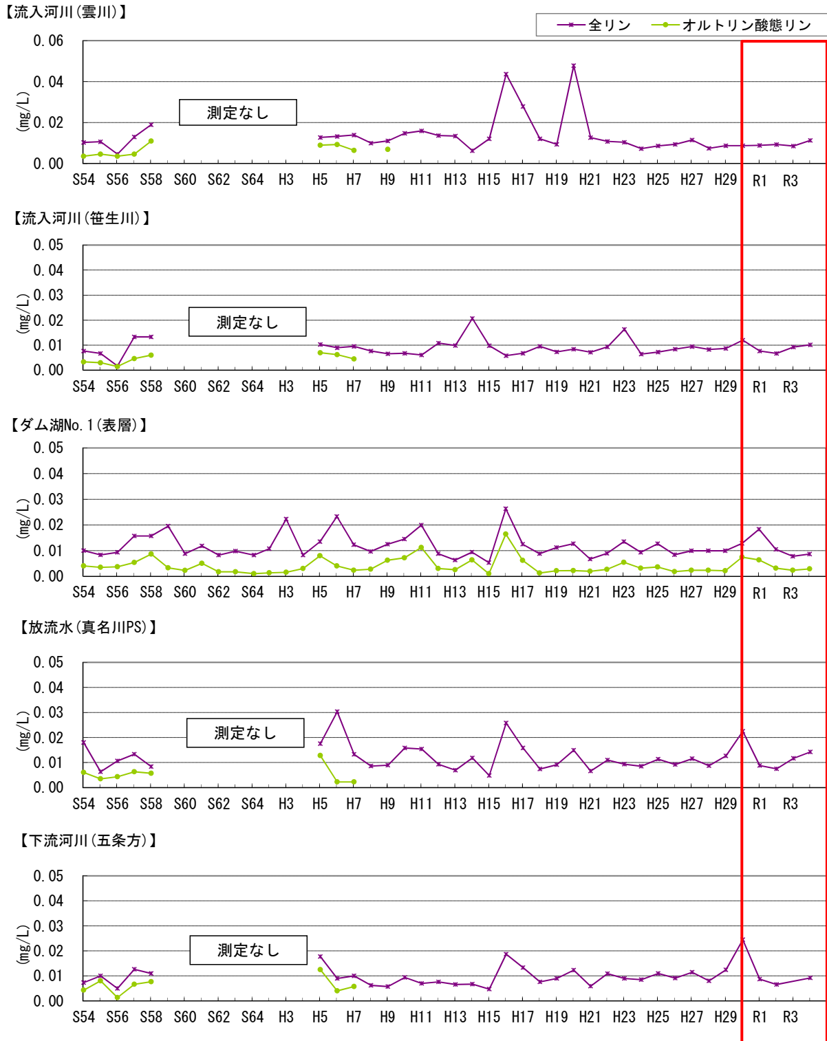
図 5.3-24(2) リンの構成形態別変化
