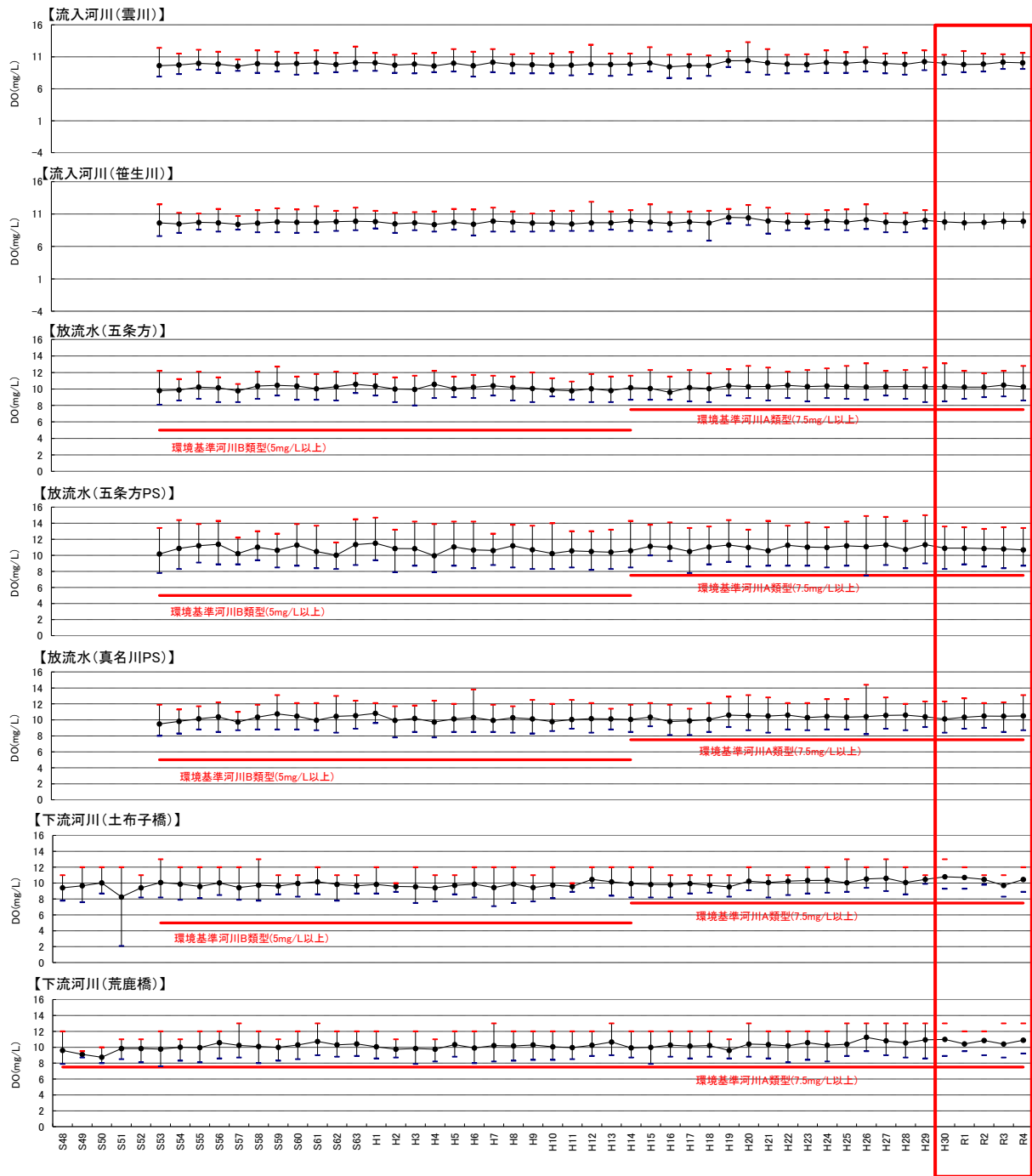
図 5.3-9(3) 各地点における流入河川、放流水及び下流河川の水質の経年変化(DO)
