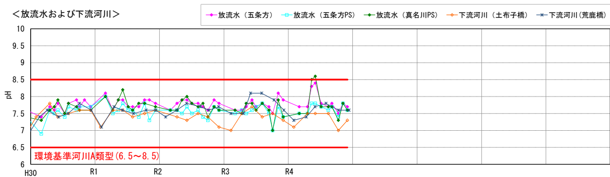
図 5.3-12(6) 流入河川、貯水池内、放流水及び下流河川の水質の経月変化 (pH: H30~R4)
