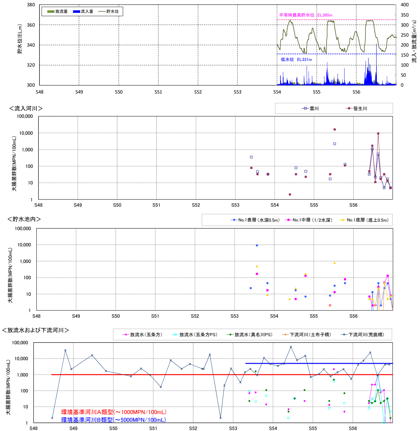
図 5.3-21(1) 流入河川、貯水池内、放流水及び下流河川の水質の経月変化 (大腸菌群数：S48～S56)
