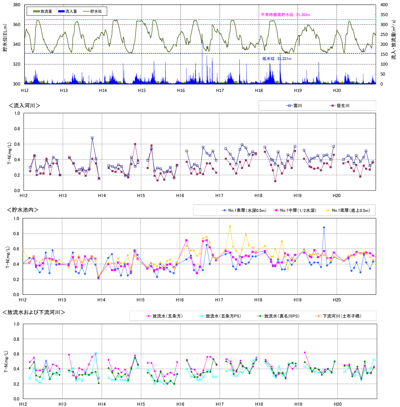
図 5.3-17(4) 流入河川、貯水池内、放流水及び下流河川の水質の経月変化 (T-N : H12~H20)
