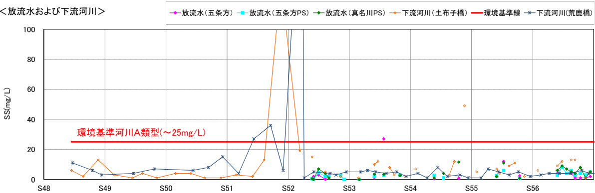
図 5.3-13(1) 流入河川、貯水池内、放流水及び下流河川の水質の経月変化 (SS : S48～S56)
