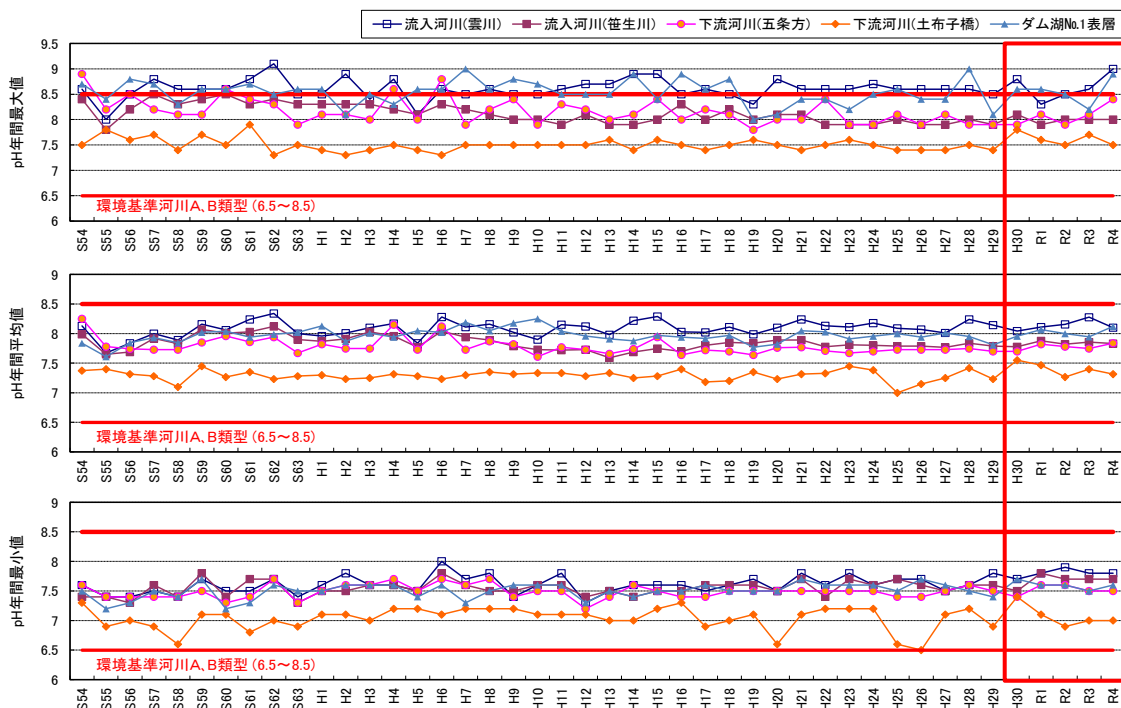
図 5.5-1 流入河川及び下流河川のpHの経年変化(最大値、平均値、最小値)
