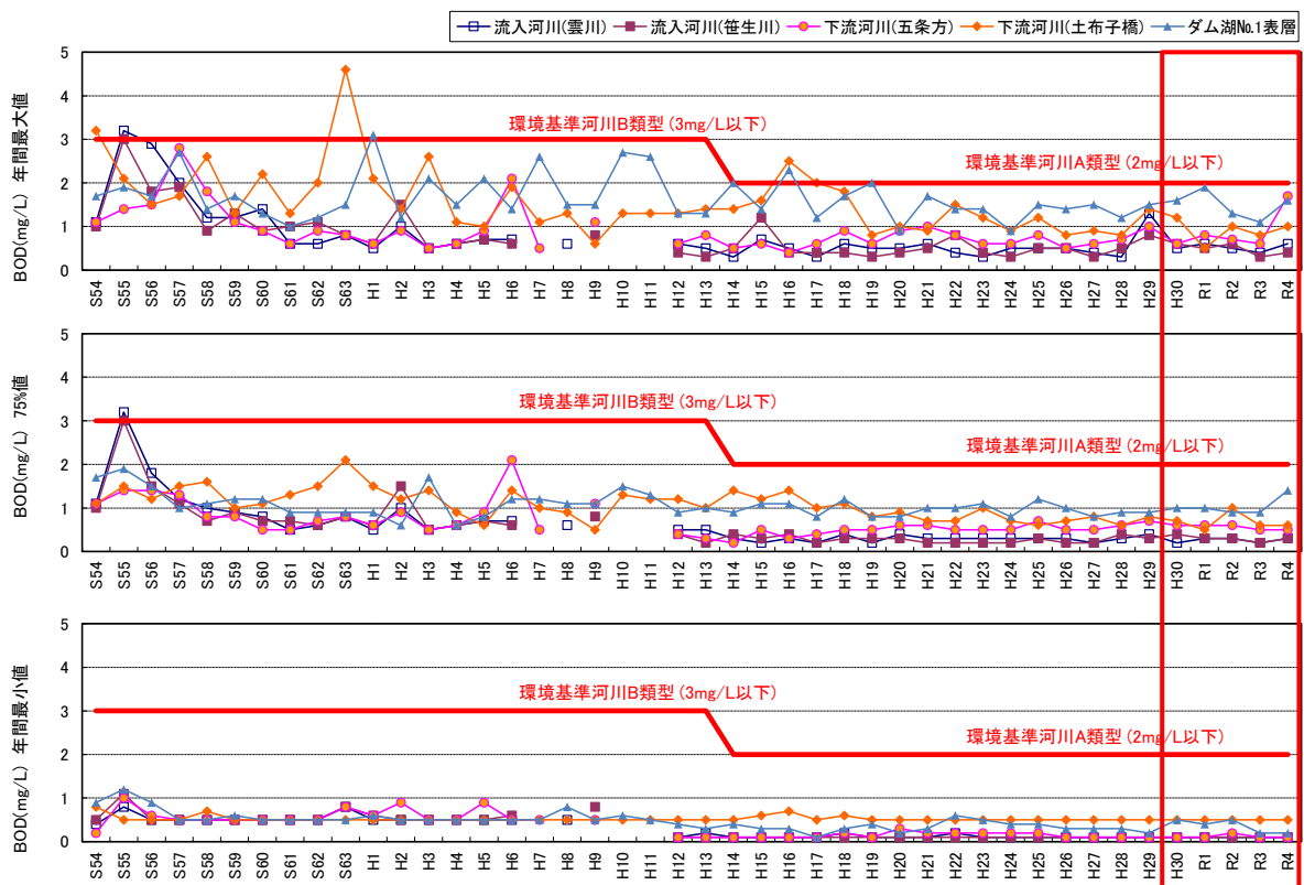
図 5.5-2 流入河川及び下流河川のBODの経年変化(最大値、75%値、最小値)
