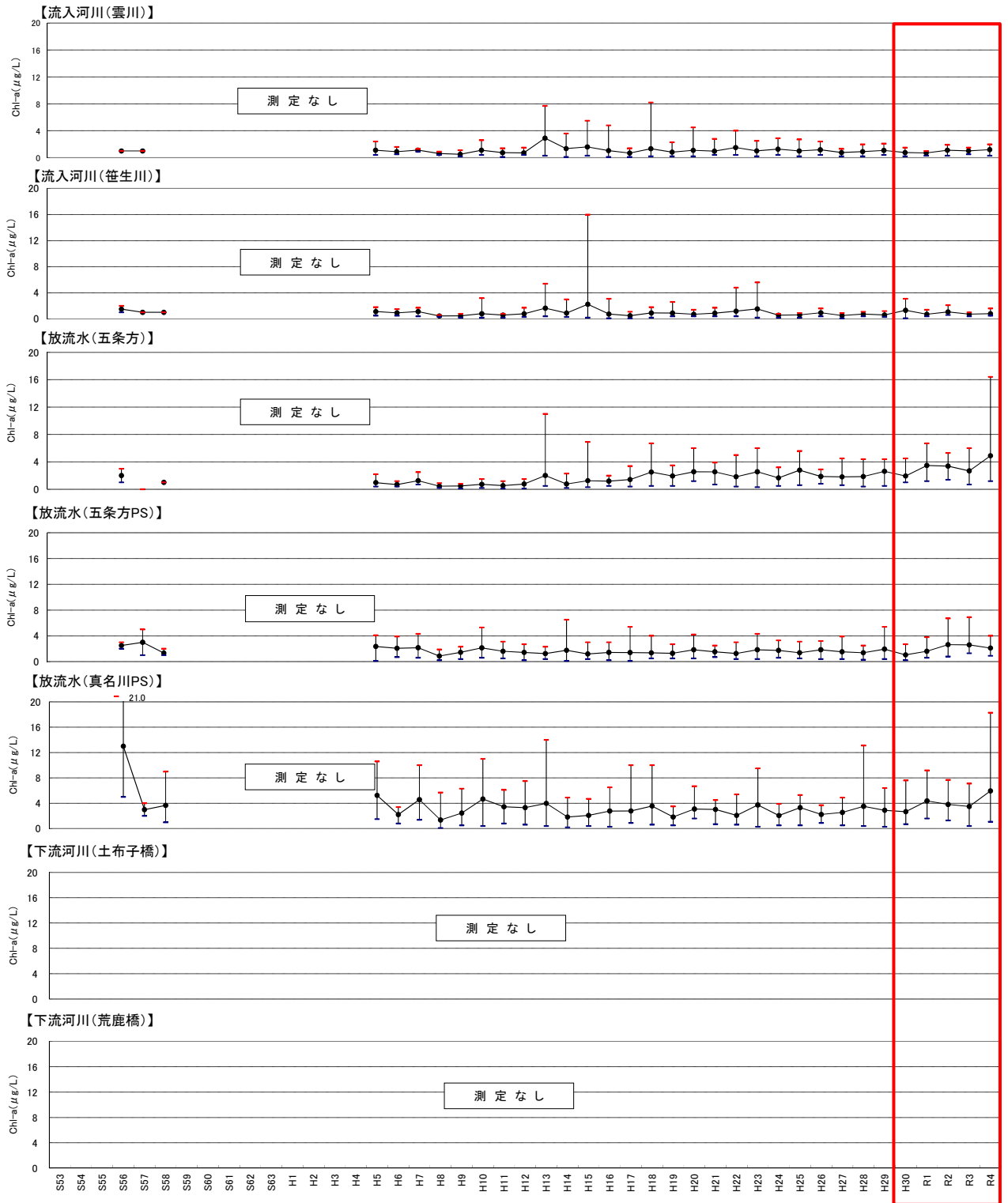
図 5.3-9(8) 各地点における流入河川、放流水及び下流河川の水質の経年変化 (クロロフィルa)
