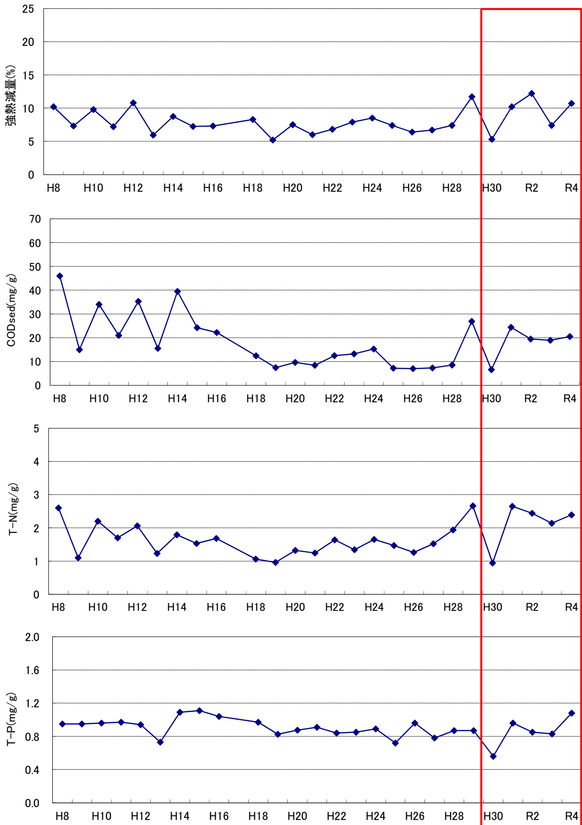
図 5.3-27(1) 底質濃度の推移(ダム湖No.1)
