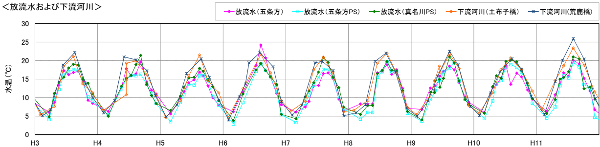
図 5.3-11(3) 流入河川、貯水池内、放流水及び下流河川の水質の経月変化 (水温: H3~H11)
