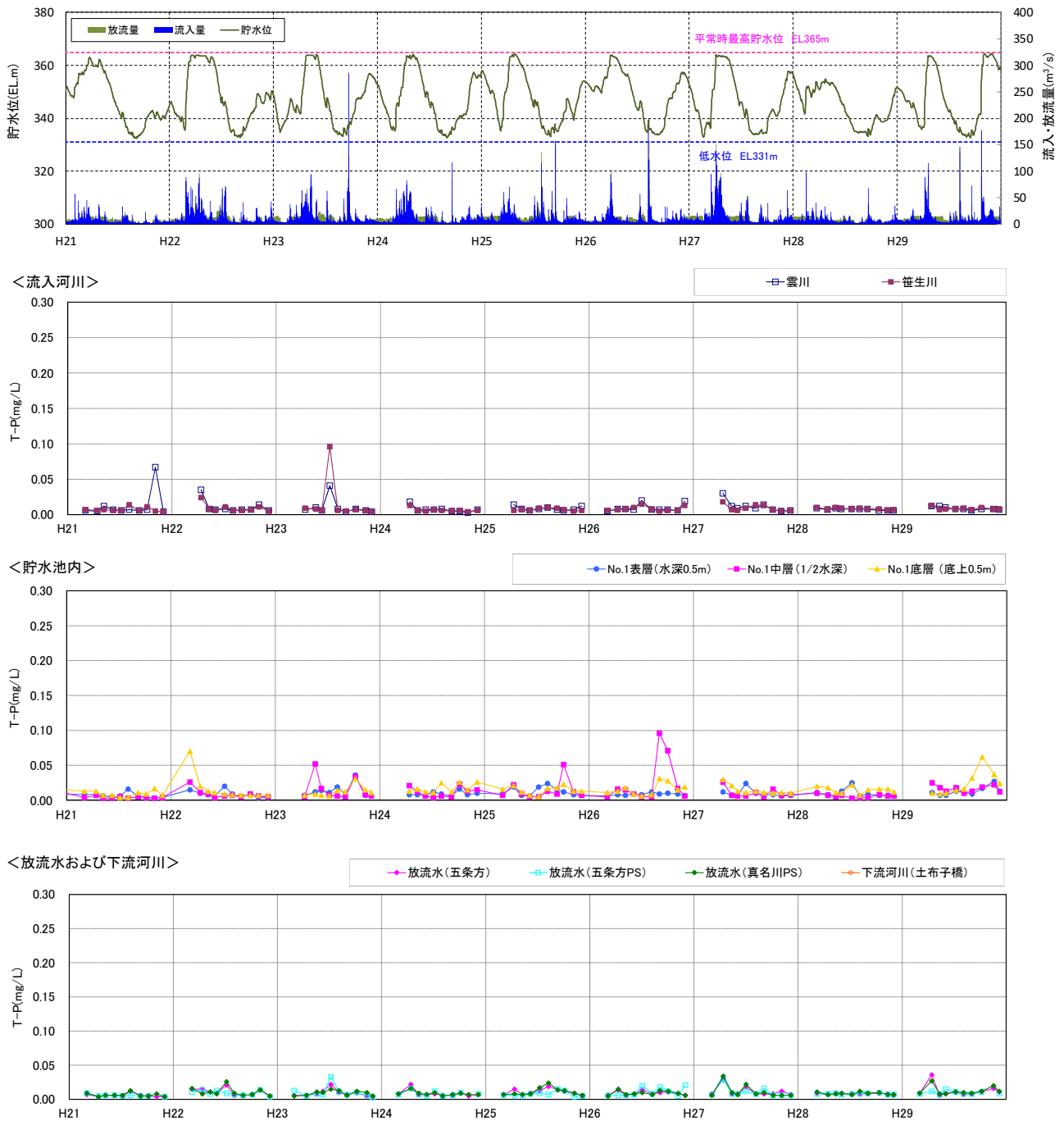
図 5.3-18(5) 流入河川、貯水池内、放流水及び下流河川の水質の経月変化 (T-P : H21~H29)
