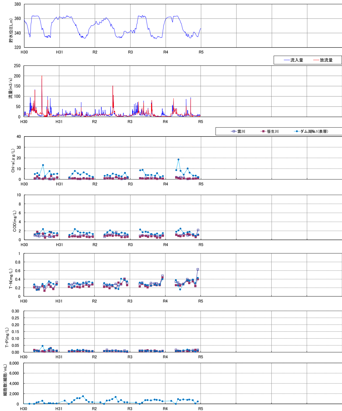
図 5.5-18(5) 富栄養化評価関連項目の経月変化(H30~R4)
