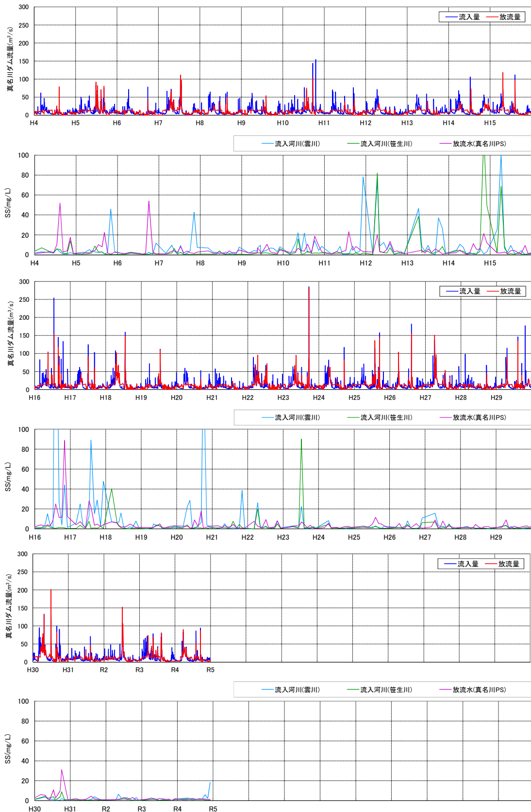
図 5.5-12(2) 流入SSと放流SSの経月変化 (H4~R4)
