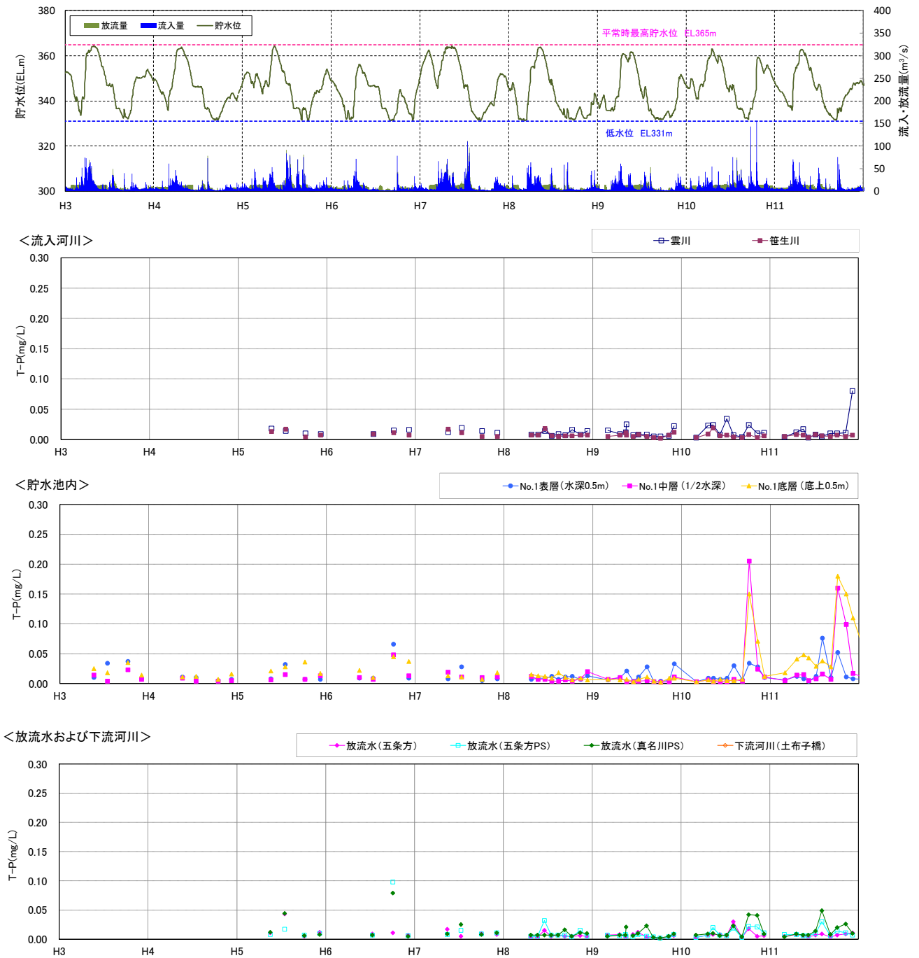
図 5.3-18(3) 流入河川、貯水池内、放流水及び下流河川の水質の経月変化 (T-P : H3~H11)
