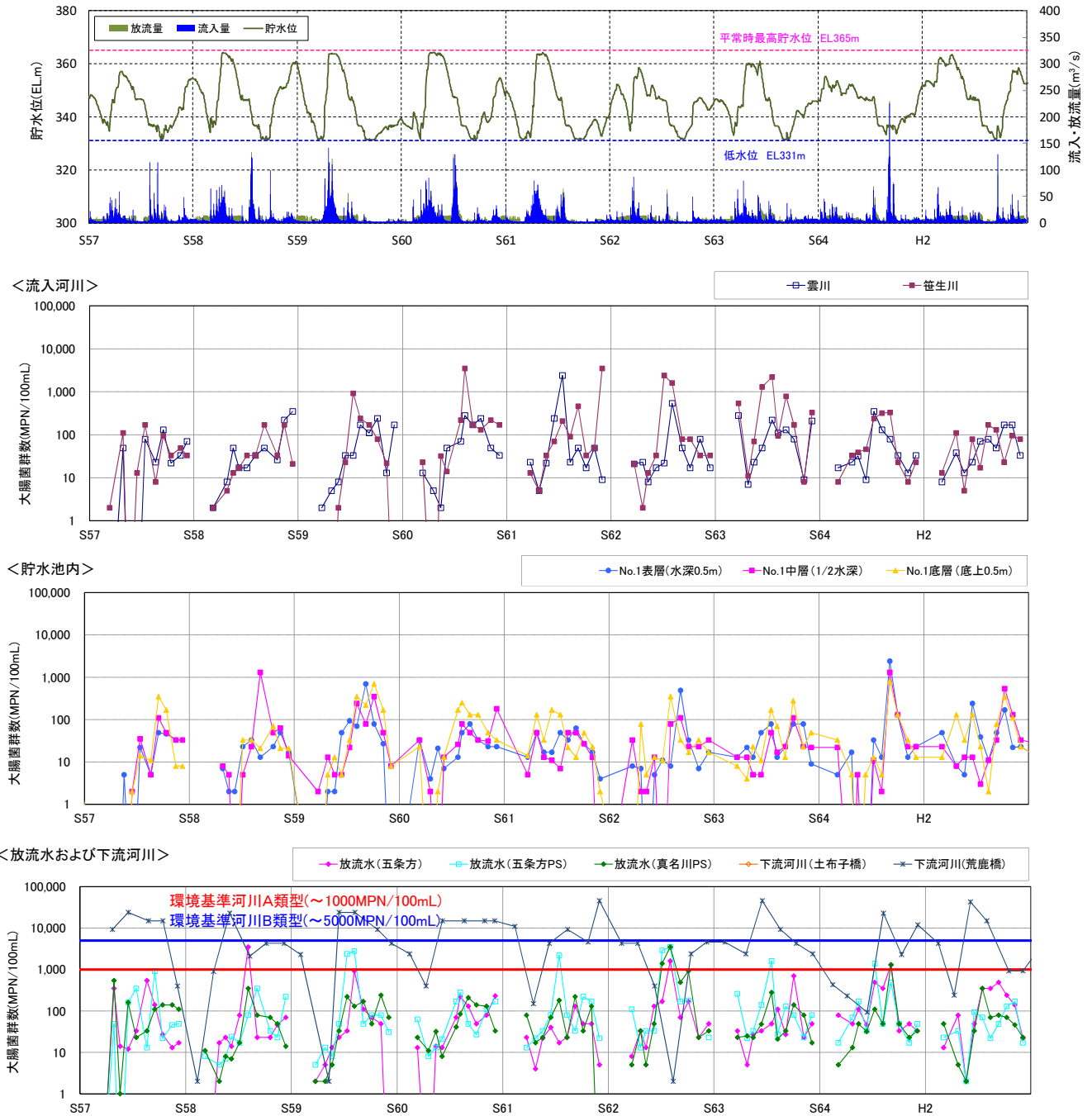
図 5.3-21(2) 流入河川、貯水池内、放流水及び下流河川の水質の経月変化 (大腸菌群数: S57~H2)
