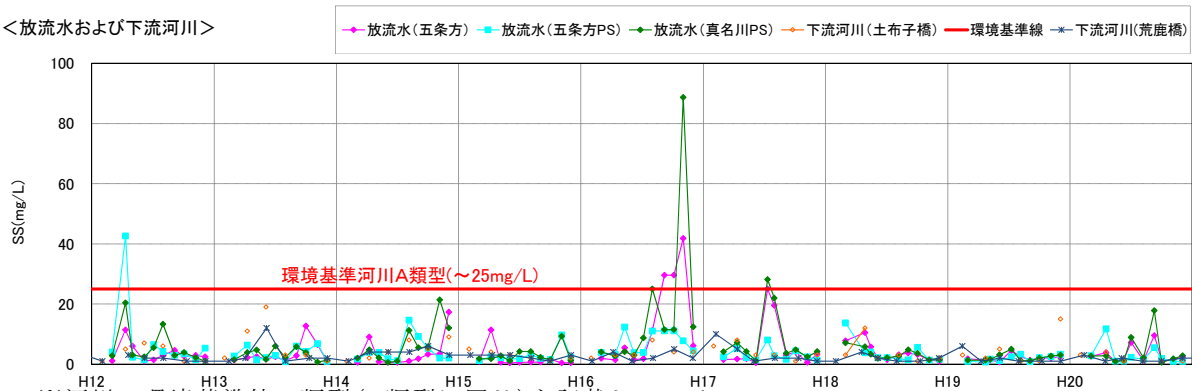
図 5.3-13(4) 流入河川、貯水池内、放流水及び下流河川の水質の経月変化 (SS : H12~H20)
