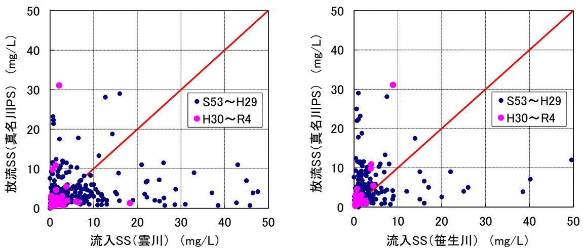
図 5.5-13(1) 流入・放流SSの比較(S54～R4)
