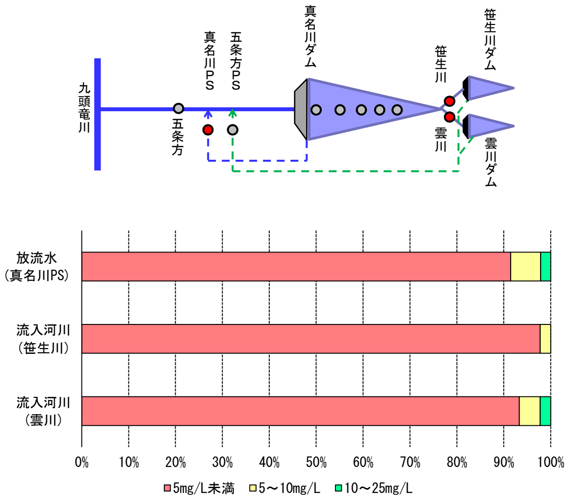
図 5.5-14 流入・放流SSの調査結果の比較 (H30~R4)
