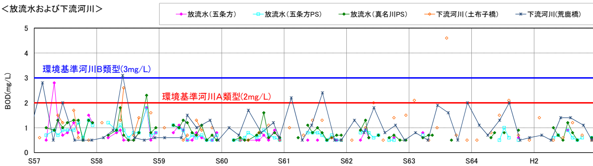
図 5.3-15(2) 流入河川、貯水池内、放流水及び下流河川の水質の経月変化 (BOD : S57~H2)
