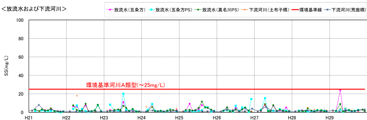
図 5.3-13(5) 流入河川、貯水池内、放流水及び下流河川の水質の経月変化 (SS : H21~H29)
