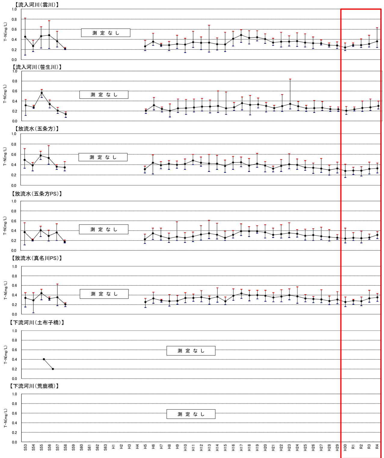
図 5.3-9(6) 各地点における流入河川、放流水及び下流河川の水質の経年変化(T-N) 【出典：平成30年度 真名川ダム定期報告書 平成31年3月】 【出典：水質調査業務報告書(真名川ダム)・データ 平成30年～令和4年】 【出典：福井県公共用水域水質測定結果 平成30年～令和4年】
