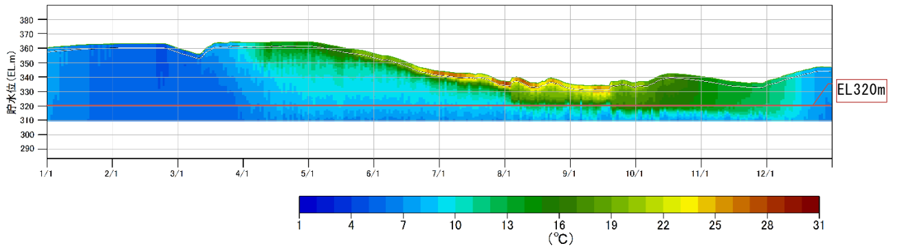
図 5.5-15(3) 真名川ダム連続観測結果(ダムサイト、水温・濁度)
