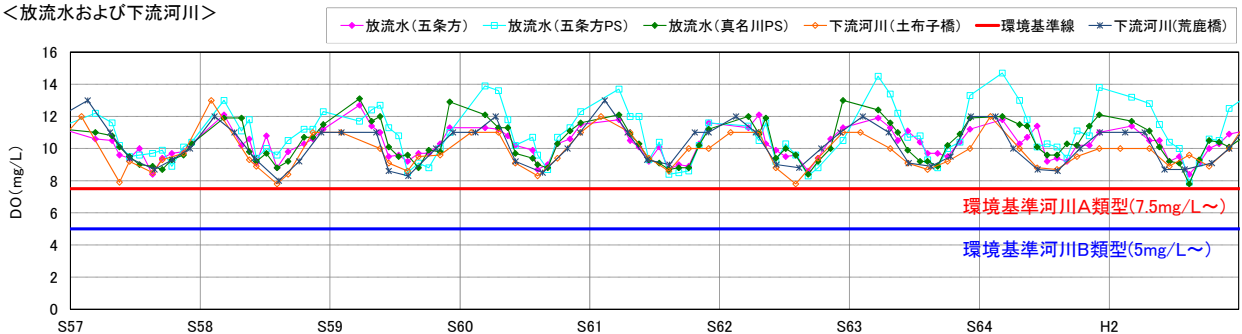
図 5.3-14(2) 流入河川、貯水池内、放流水及び下流河川の水質の経月変化 (DO : S57~H2)
