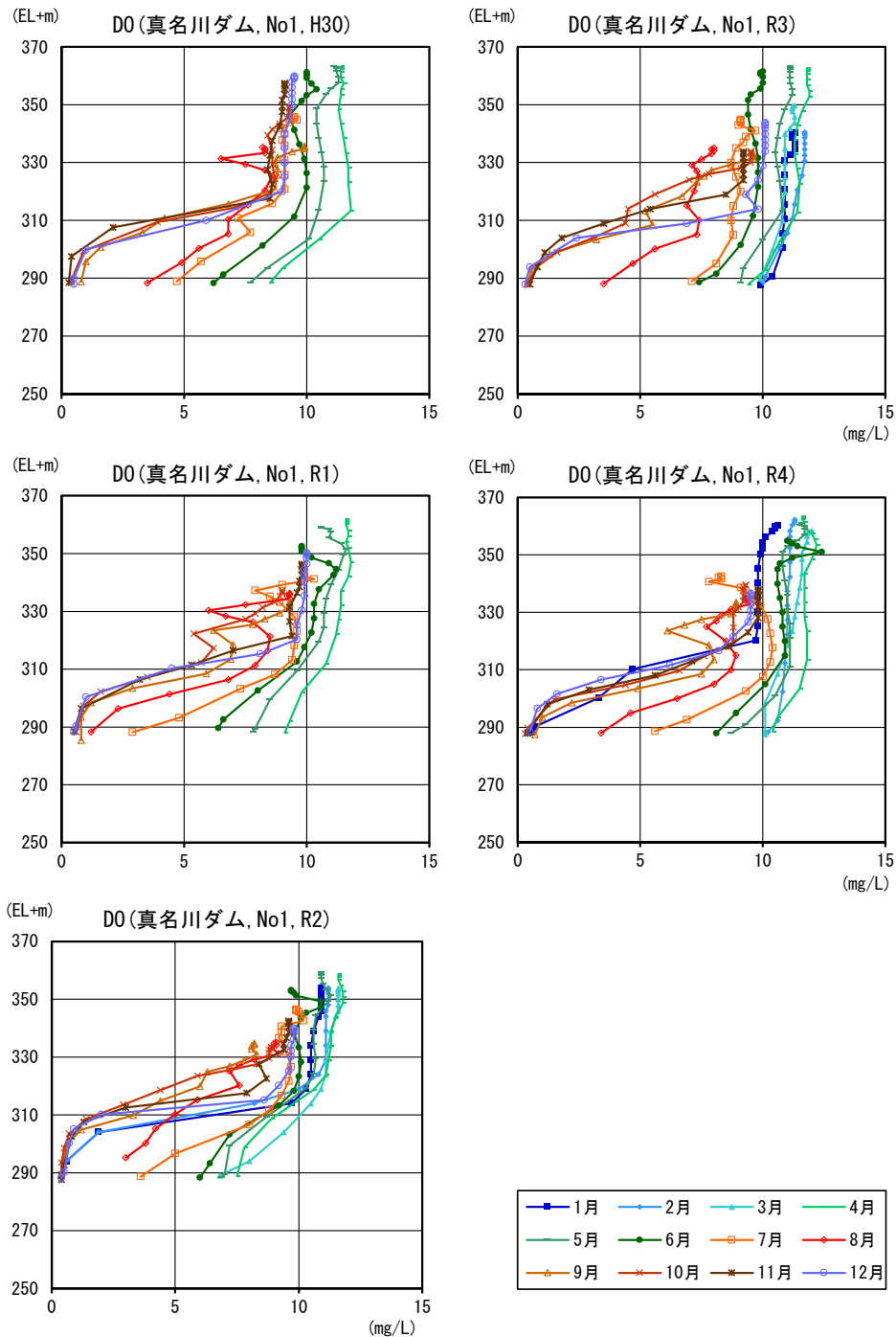
図 5.5-20 D0鉛直分布図(ダム湖No.1)
