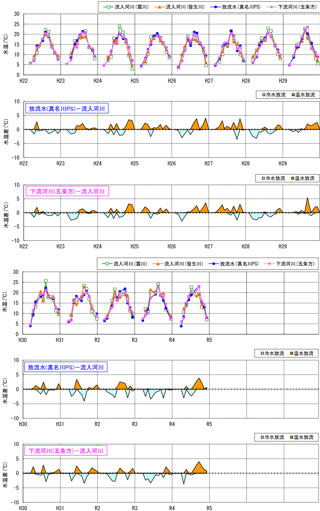
図 5.5-8(3) 流入河川・放流水・下流河川の水温の経月変化(H22~R4)
