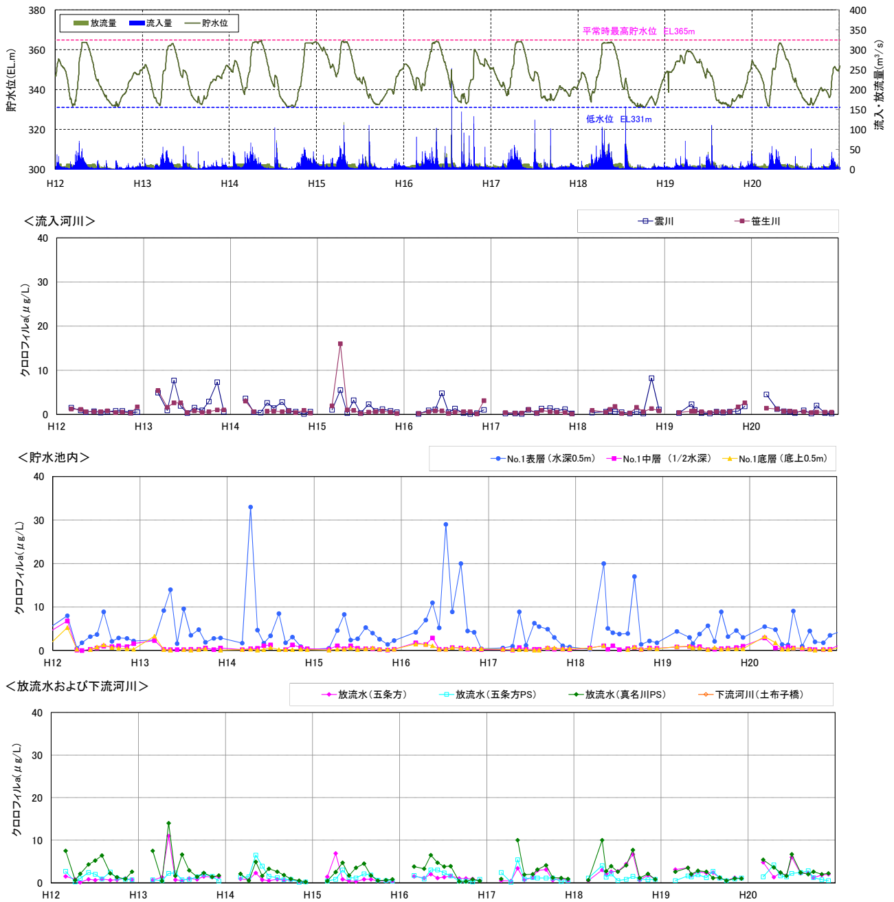
図 5.3-19(4) 流入河川、貯水池内、放流水及び下流河川の水質の経月変化 (クロロフィルa : H12~H20)
