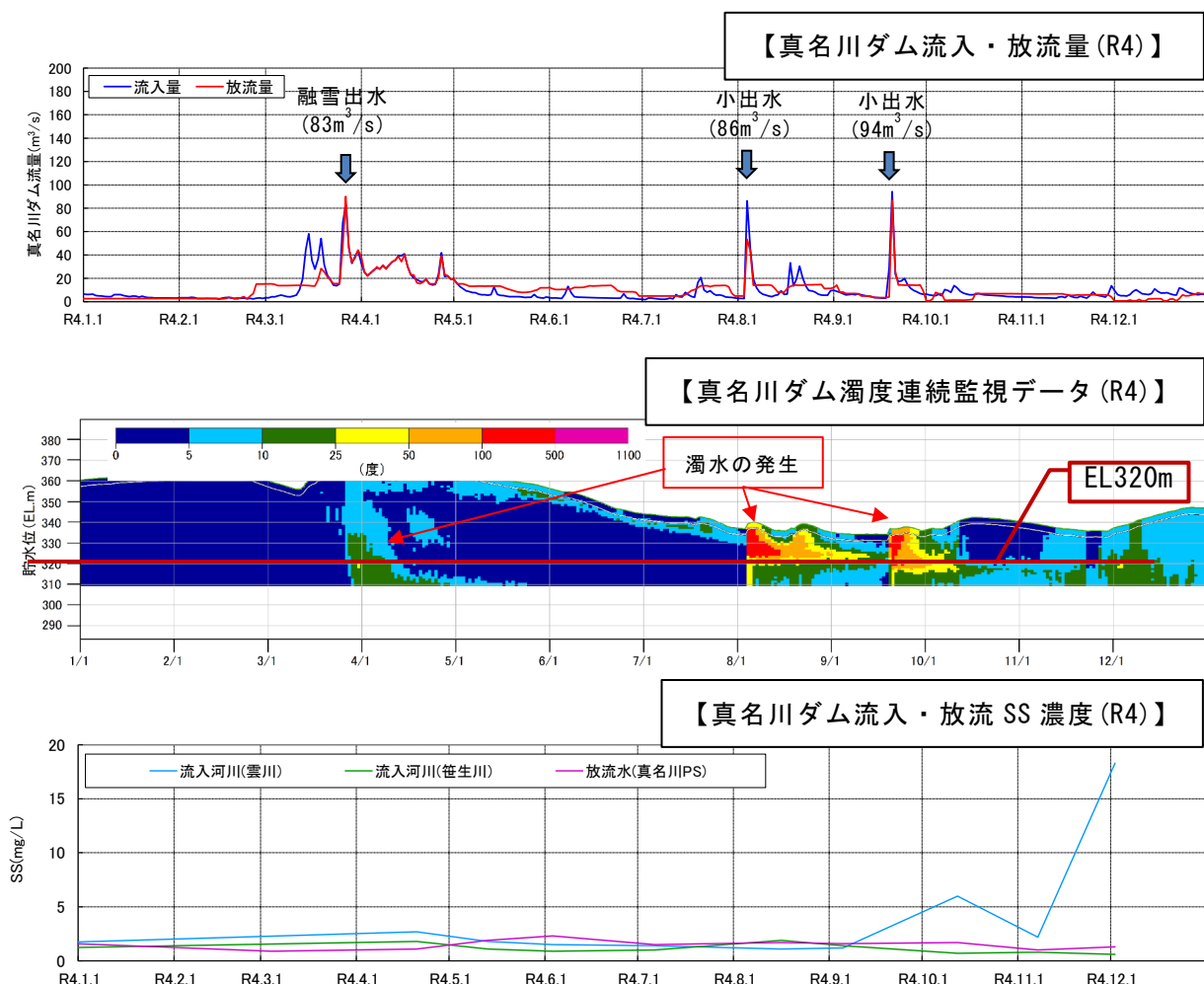
図 5.5-16 令和4年の真名川ダム濁水発生状況と流入・放流水の濁度変化
