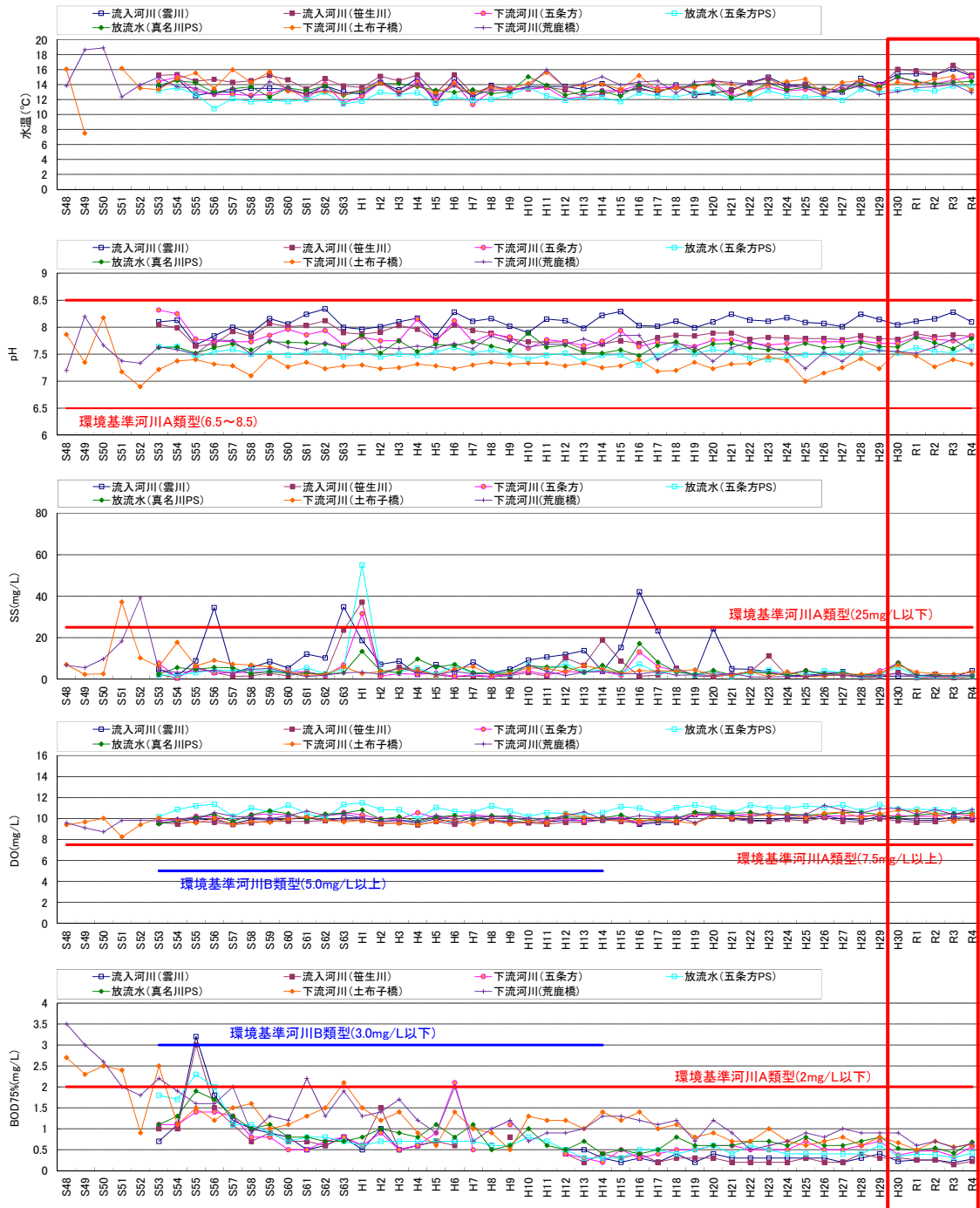
図 5.3-8(1) 流入河川、放流水及び下流河川の水質の経年変化
