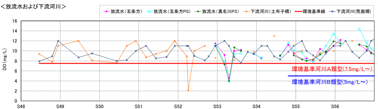
図 5.3-14(1) 流入河川、貯水池内、放流水及び下流河川の水質の経月変化 (DO : S48～S56)
