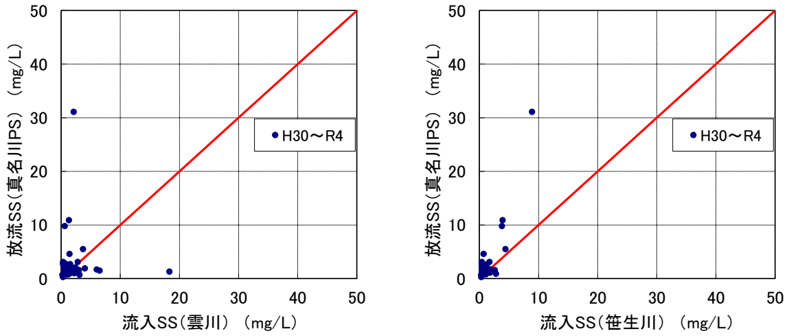
図 5.5-13(6) 流入・放流SSの比較(H30~R4)
