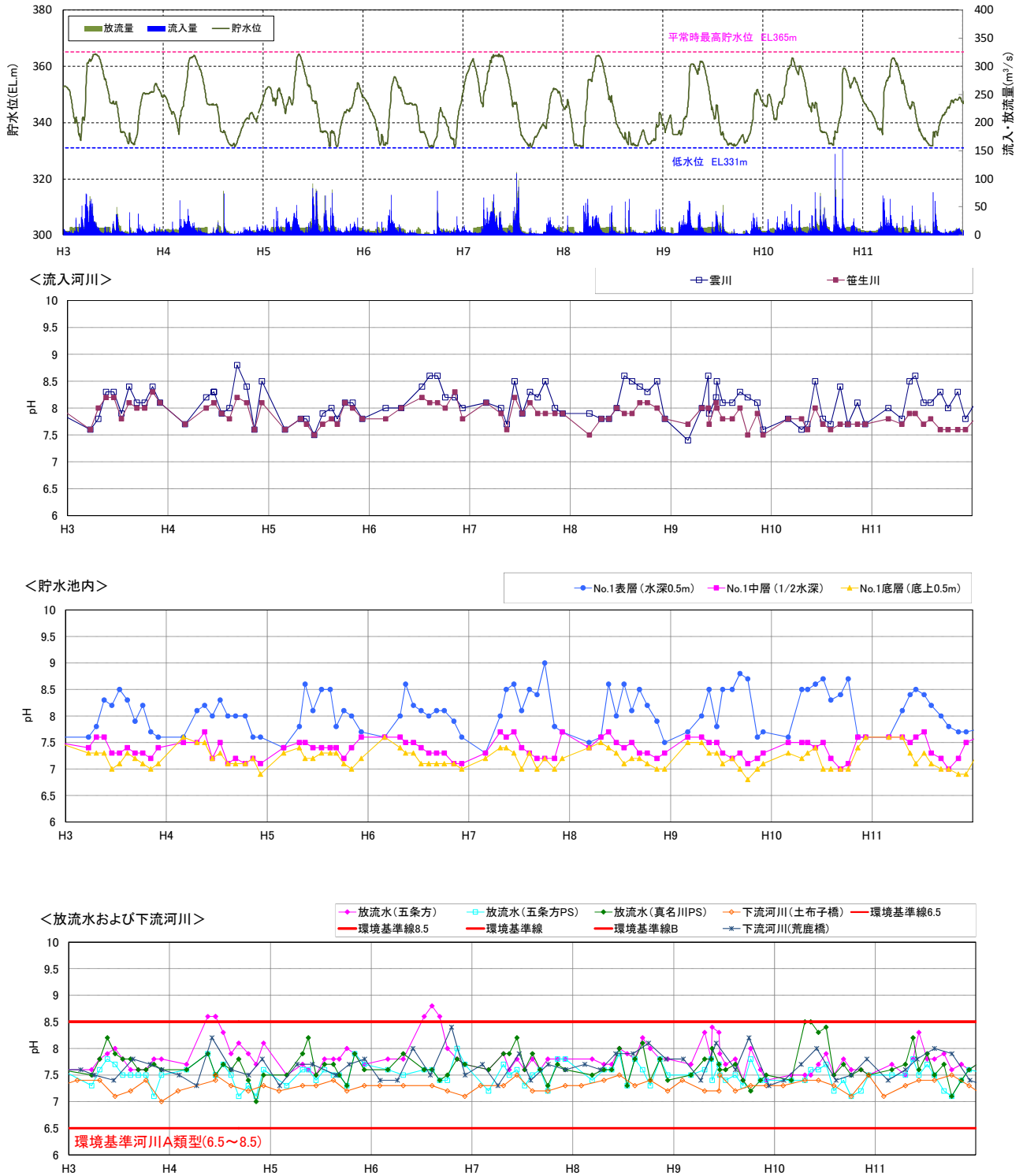
図 5.3-12(3) 流入河川、貯水池内、放流水及び下流河川の水質の経月変化 (pH : H3~H11)
