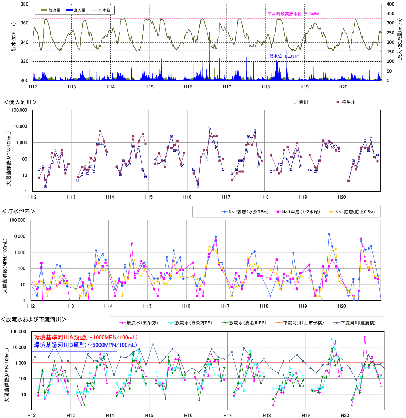
図 5.3-21(4) 流入河川、貯水池内、放流水及び下流河川の水質の経月変化 (大腸菌群数 : H12~H20)
