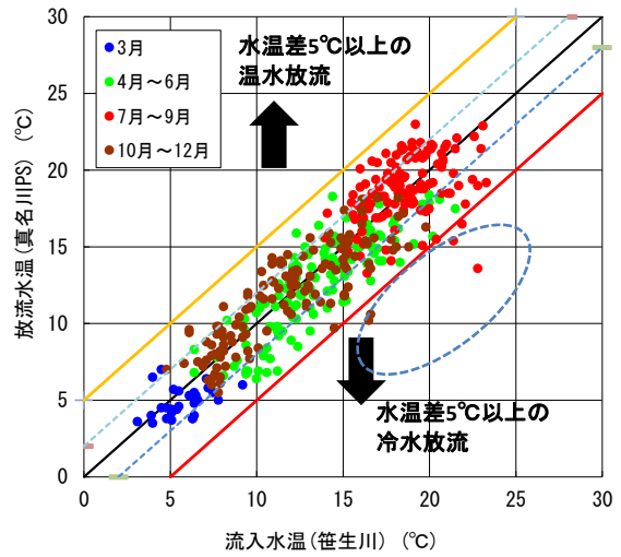
図 5.5-9(1) 流入・放流水温の比較 (S54~R4)
