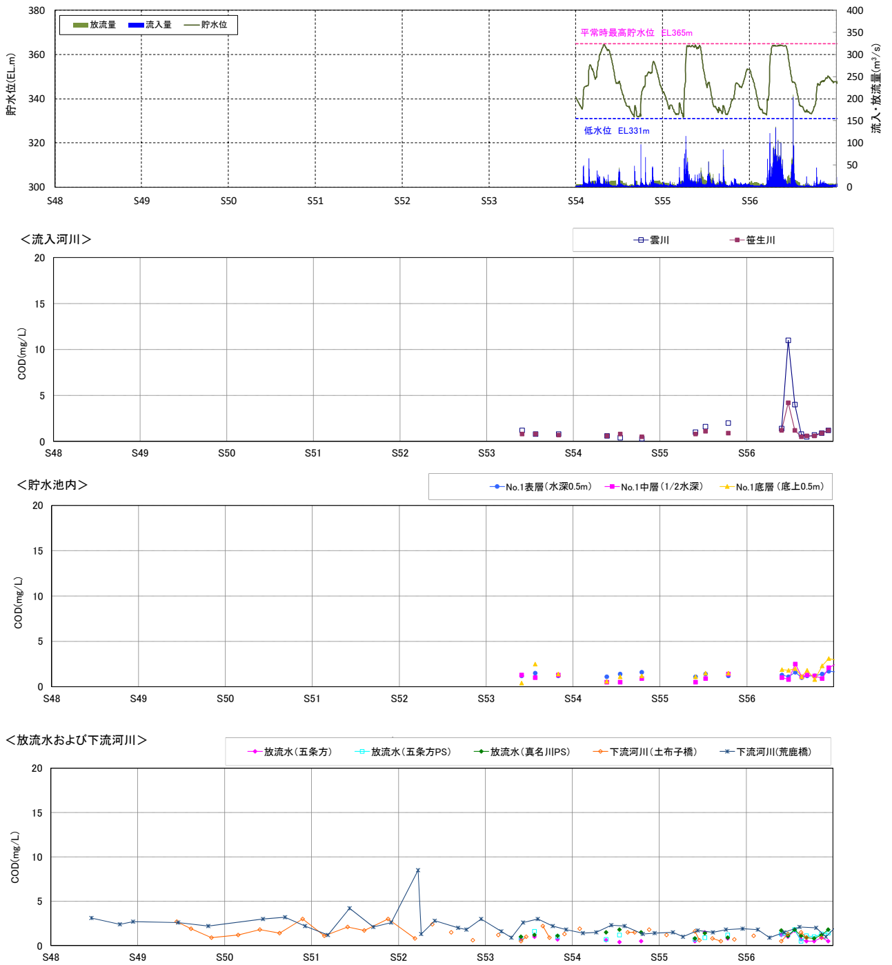
図 5.3-16(1) 流入河川、貯水池内、放流水及び下流河川の水質の経月変化 (COD : S48~S56)
