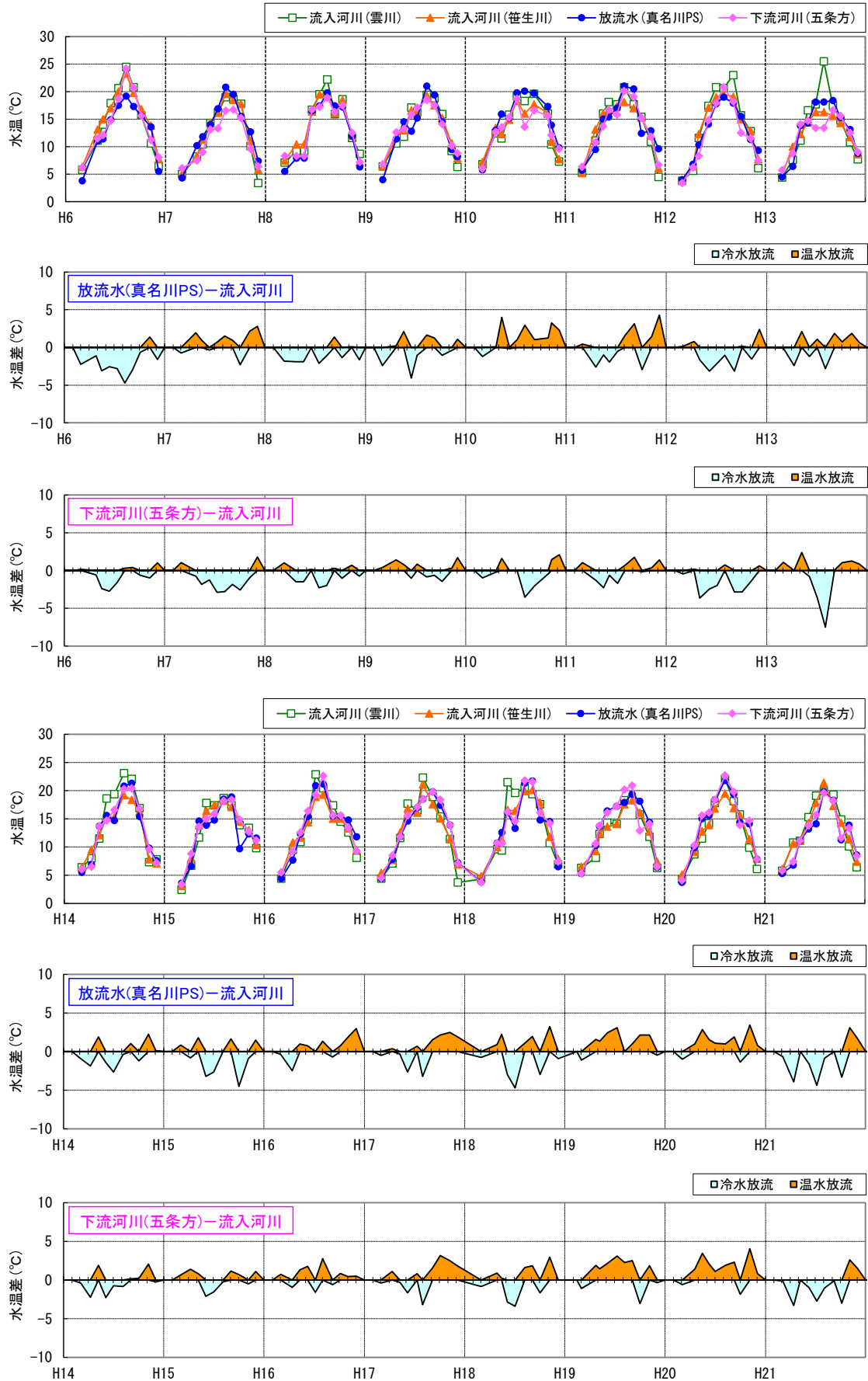
図 5.5-8(2) 流入河川・放流水・下流河川の水温の経月変化(H6~H21)
