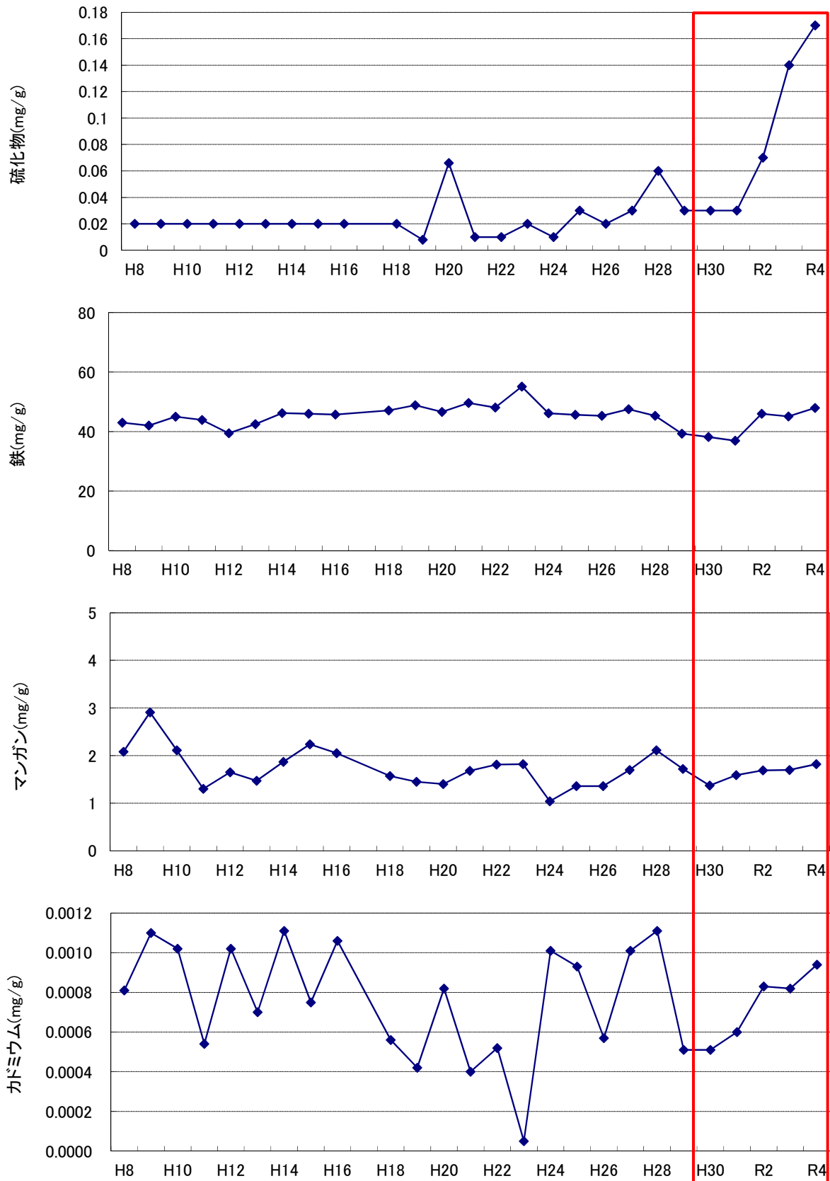
図 5.3-27(2) 底質濃度の推移(ダム湖No.1)
