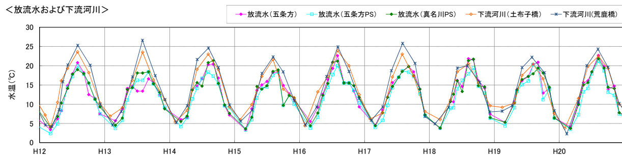
図 5.3-11(4) 流入河川、貯水池内、放流水及び下流河川の水質の経月変化 (水温: H12~H20)
