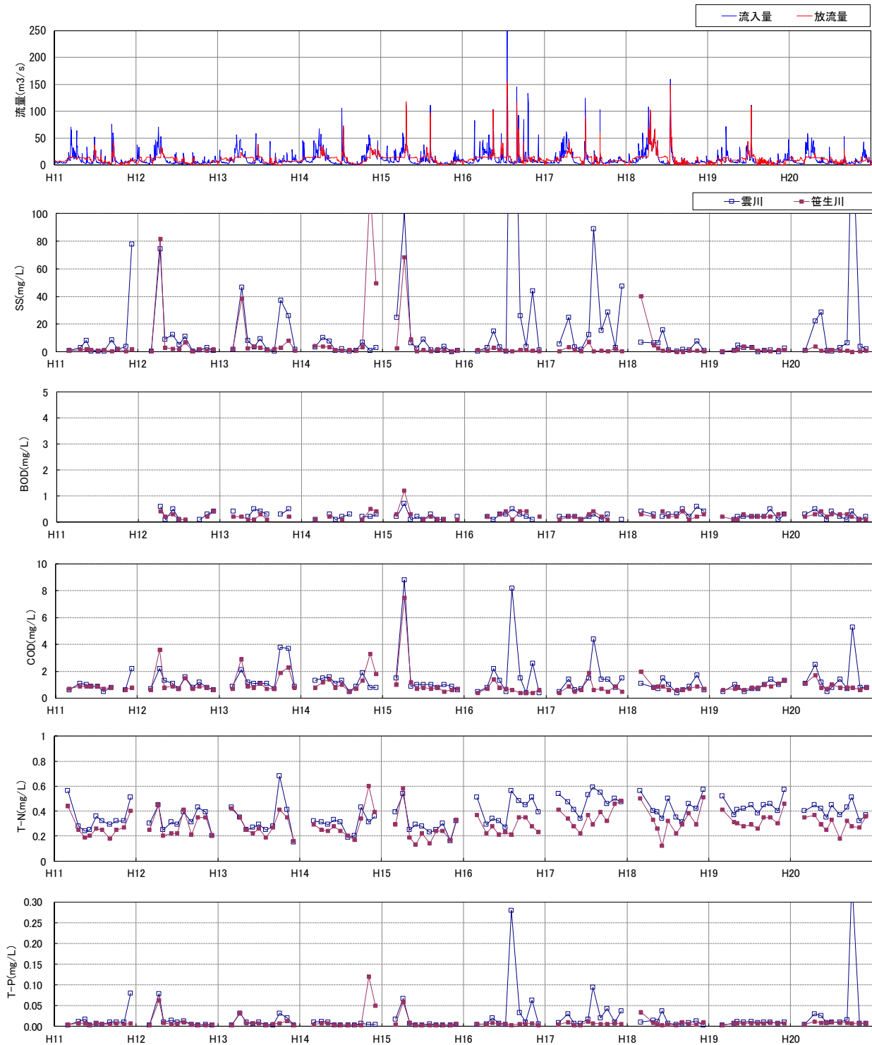
図 5.4-6 (3) 真名川ダム流入水質の状況 (H11~H20)
