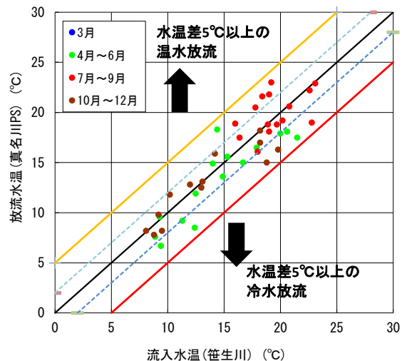
図 5.5-9(6) 流入・放流水温の比較 (H30~R4)
