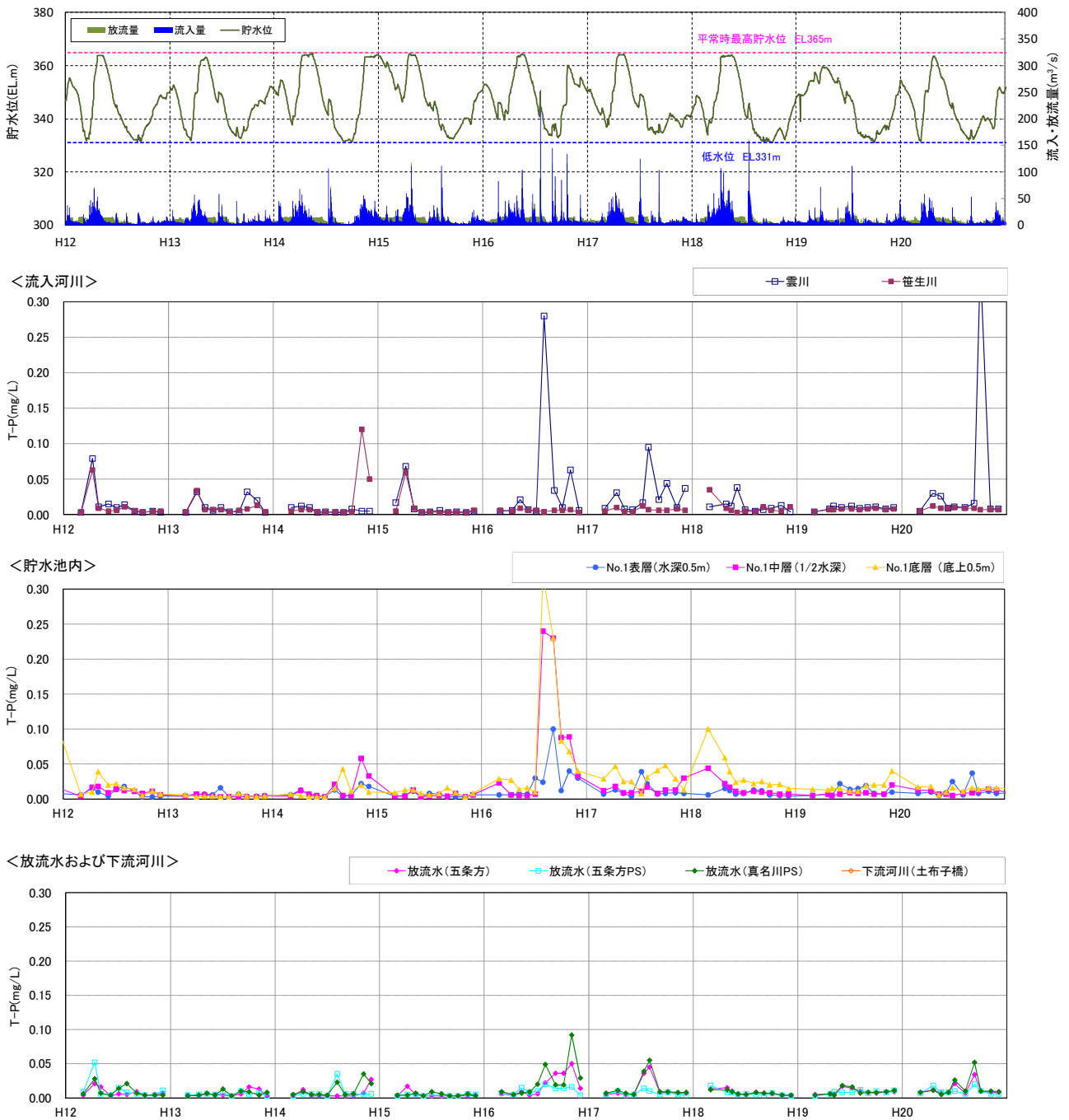
図 5.3-18(4) 流入河川、貯水池内、放流水及び下流河川の水質の経月変化 (T-P : H12~H20)
