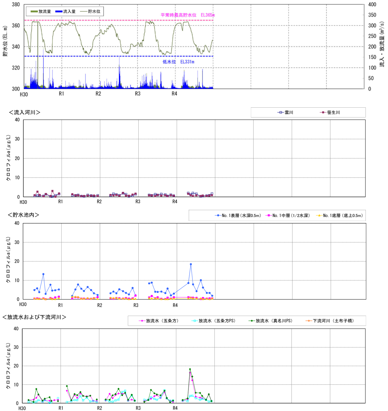
図 5.3-19(6) 流入河川、貯水池内、放流水及び下流河川の水質の経月変化 (クロロフィルa : H30~R4)
