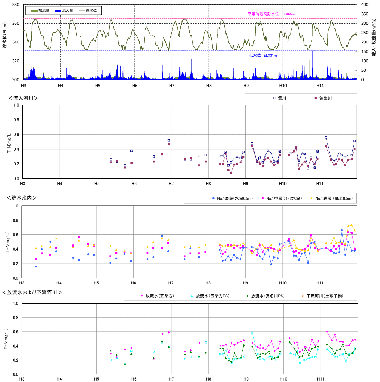
図 5.3-17(3) 流入河川、貯水池内、放流水及び下流河川の水質の経月変化 (T-N : H3~H11)
