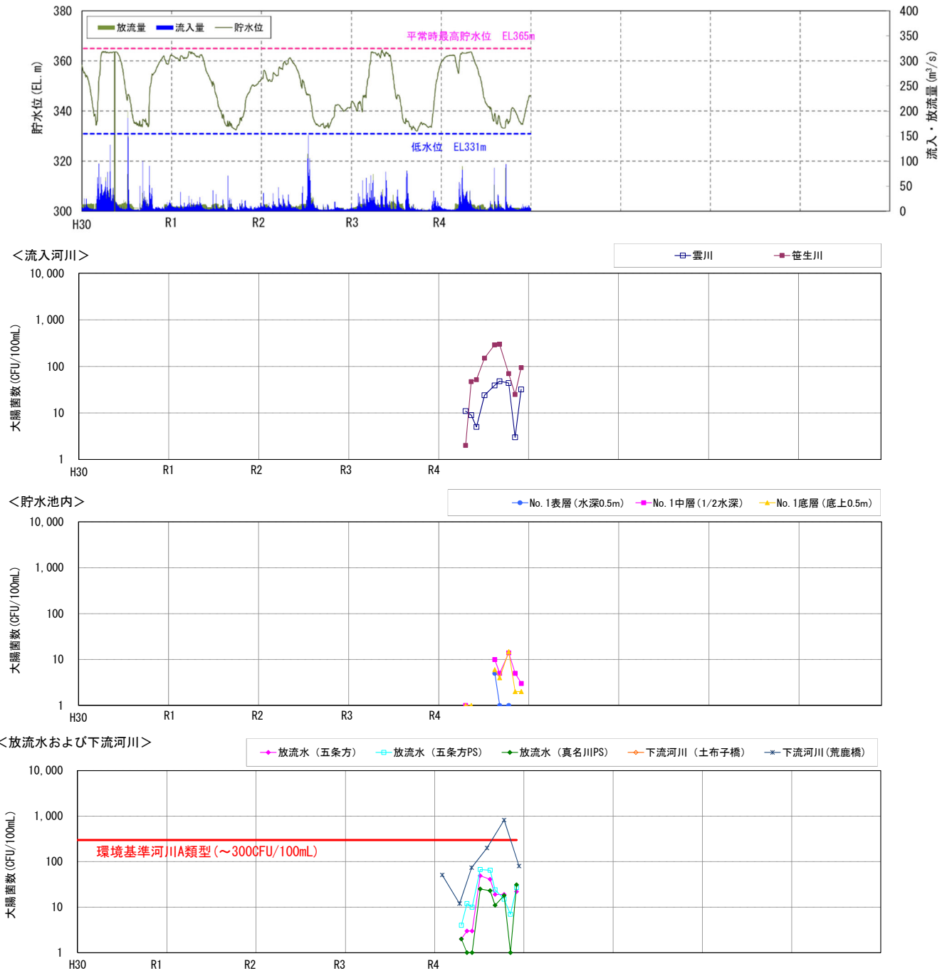
図 5.3-20(1) 流入河川、貯水池内、放流水及び下流河川の水質の経月変化 (大腸菌数：H30～R4)
