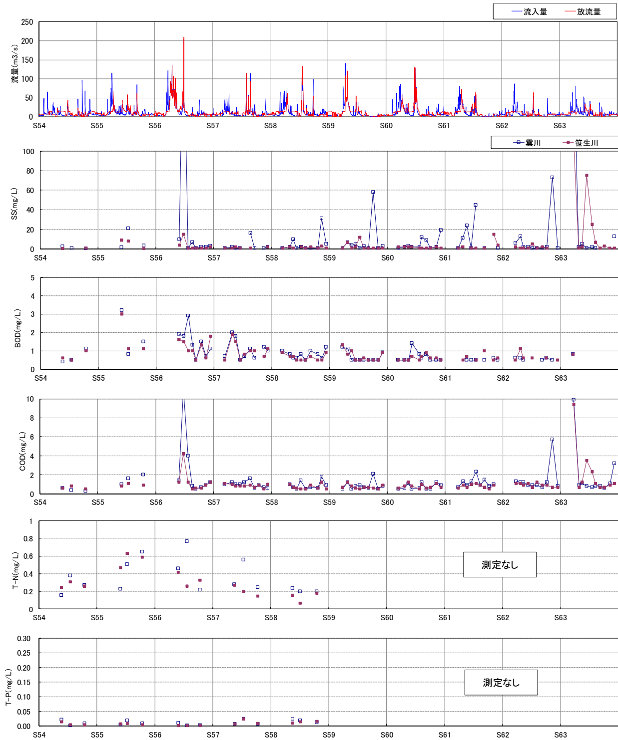
図 5.4-6(1) 真名川ダム流入水質の状況(S54~S63)
