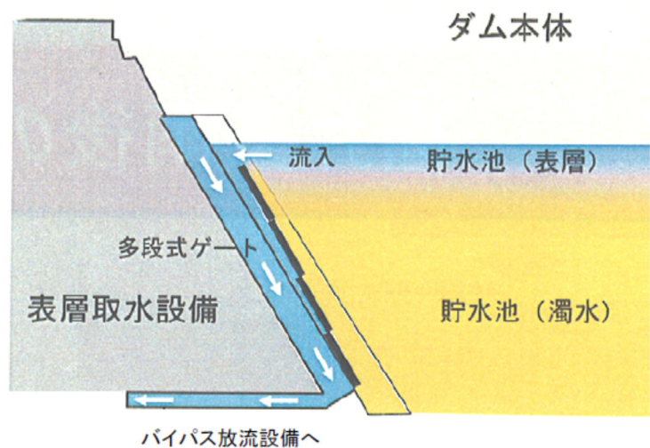
図 5.1-5 発電取水設備
