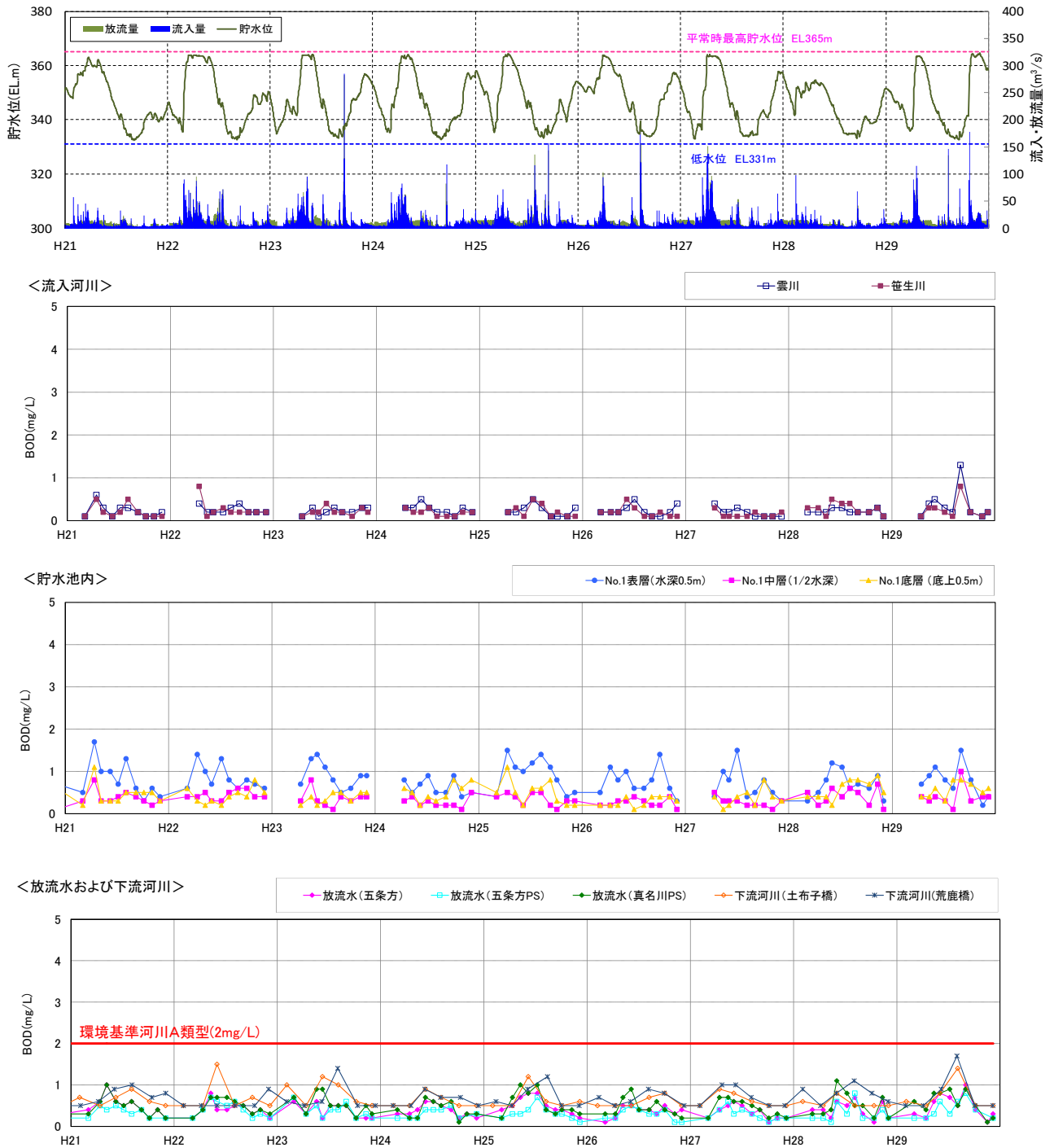
図 5.3-15(5) 流入河川、貯水池内、放流水及び下流河川の水質の経月変化 (BOD: H21~H29)
