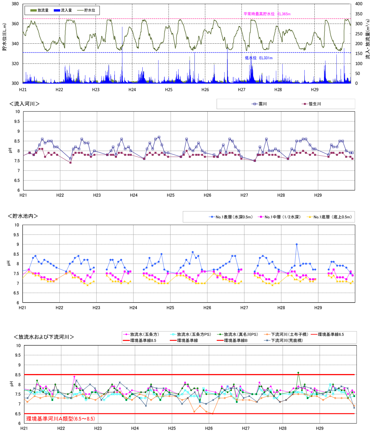
図 5.3-12(5) 流入河川、貯水池内、放流水及び下流河川の水質の経月変化 (pH : H21~H29)
