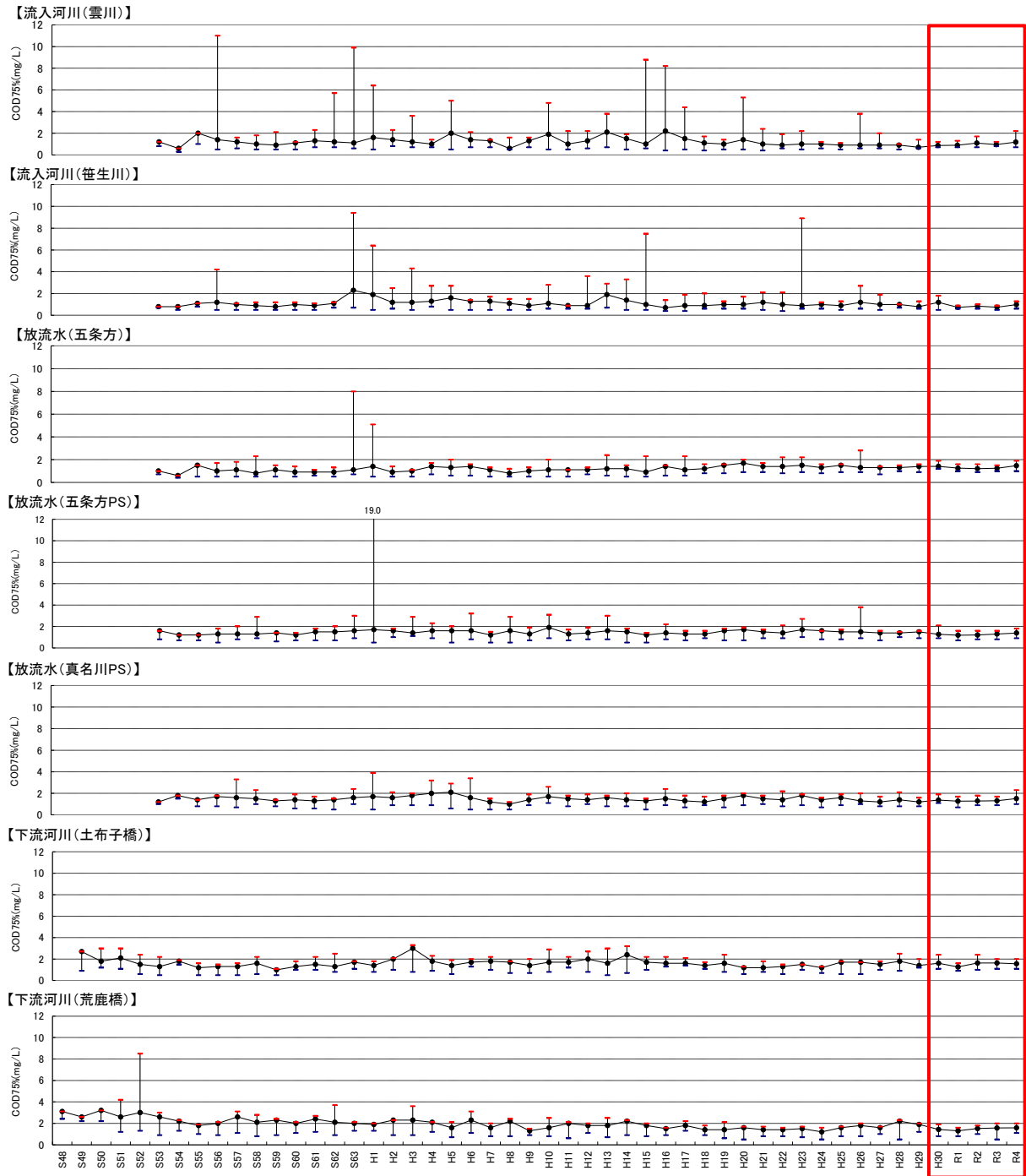
図 5.3-9(5) 各地点における流入河川、放流水及び下流河川の水質の経年変化(COD) 【出典：平成30年度 真名川ダム定期報告書 平成31年3月】 【出典：水質調査業務報告書(真名川ダム)・データ 平成30年～令和4年】 【出典：福井県公共用水域水質測定結果 平成30年～令和4年】
