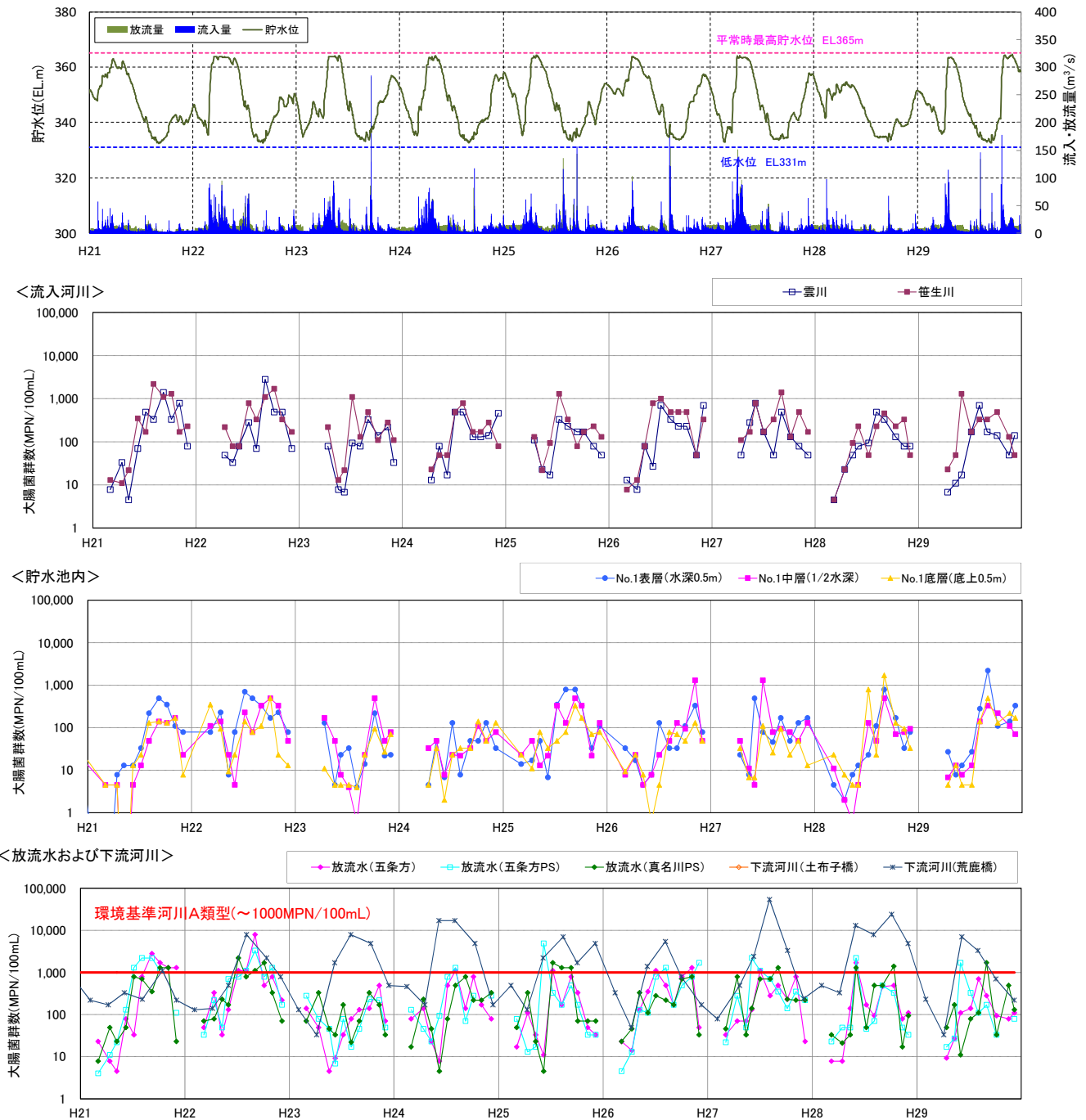
図 5.3-21(5) 流入河川、貯水池内、放流水及び下流河川の水質の経月変化 (大腸菌群数: H21~H29)
