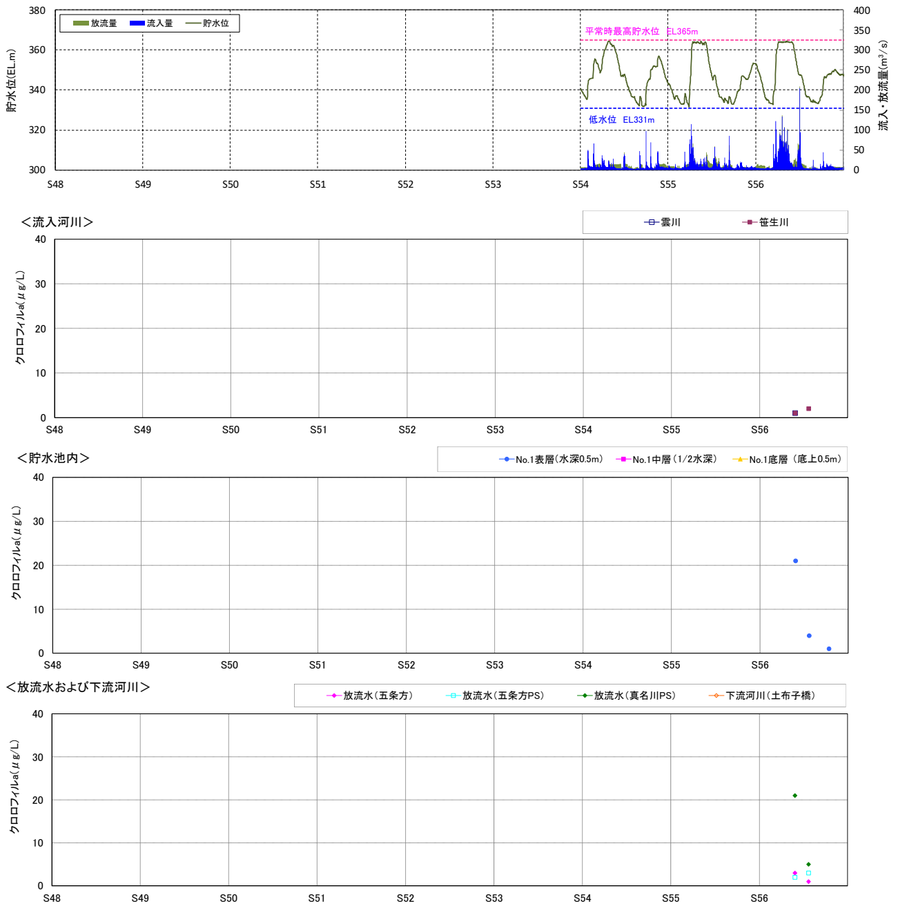
図 5.3-19(1) 流入河川、貯水池内、放流水及び下流河川の水質の経月変化 (クロロフィルa : S48~S56)
