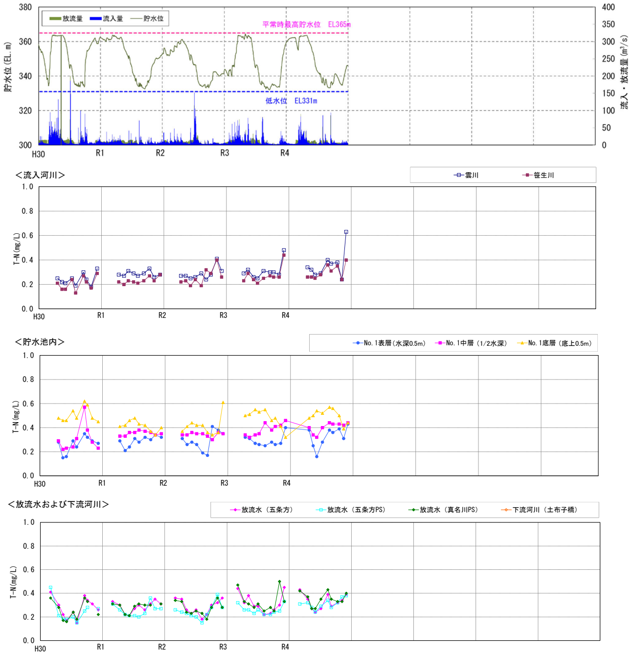
図 5.3-17(6) 流入河川、貯水池内、放流水及び下流河川の水質の経月変化 (T-N : H30~R4)
