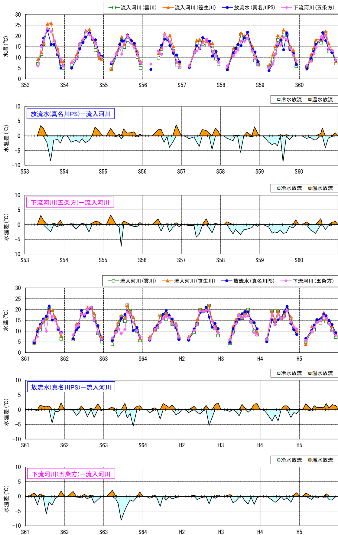
図 5.5-8(1) 流入河川・放流水・下流河川の水温の経月変化(S53~H5)
