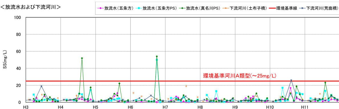
図 5.3-13(3) 流入河川、貯水池内、放流水及び下流河川の水質の経月変化 (SS: H3～H11)
