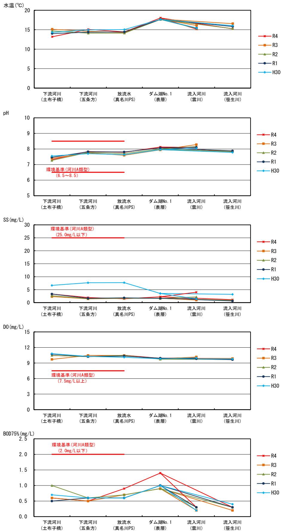
図 5.5-22(1) 水質縦断変化
