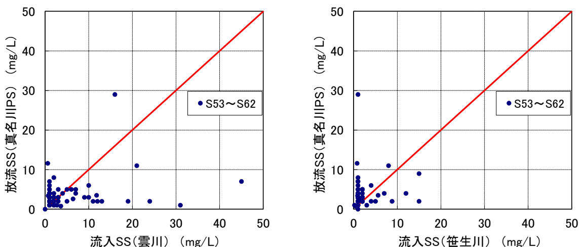
図 5.5-13(2) 流入・放流SSの比較(S53～S62)
