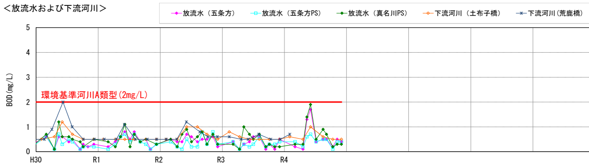
図 5.3-15(6) 流入河川、貯水池内、放流水及び下流河川の水質の経月変化 (BOD : H30~R4)
