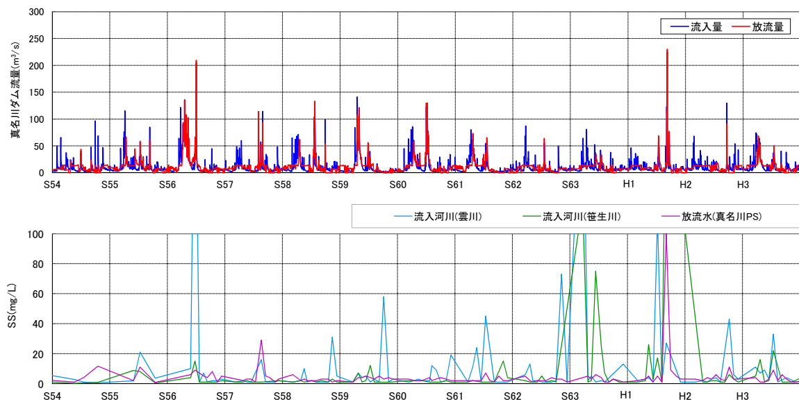
図 5.5-12(1) 流入SSと放流SSの経月変化(S54～H3)
