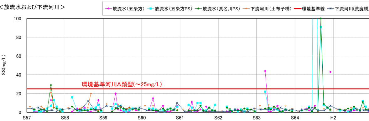
図 5.3-13(2) 流入河川、貯水池内、放流水及び下流河川の水質の経月変化 (SS: S57~H2)
