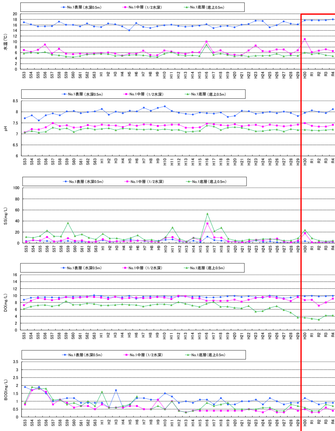
図 5.3-10(1) 貯水池内の水質の経年変化(ダム湖No.1)
