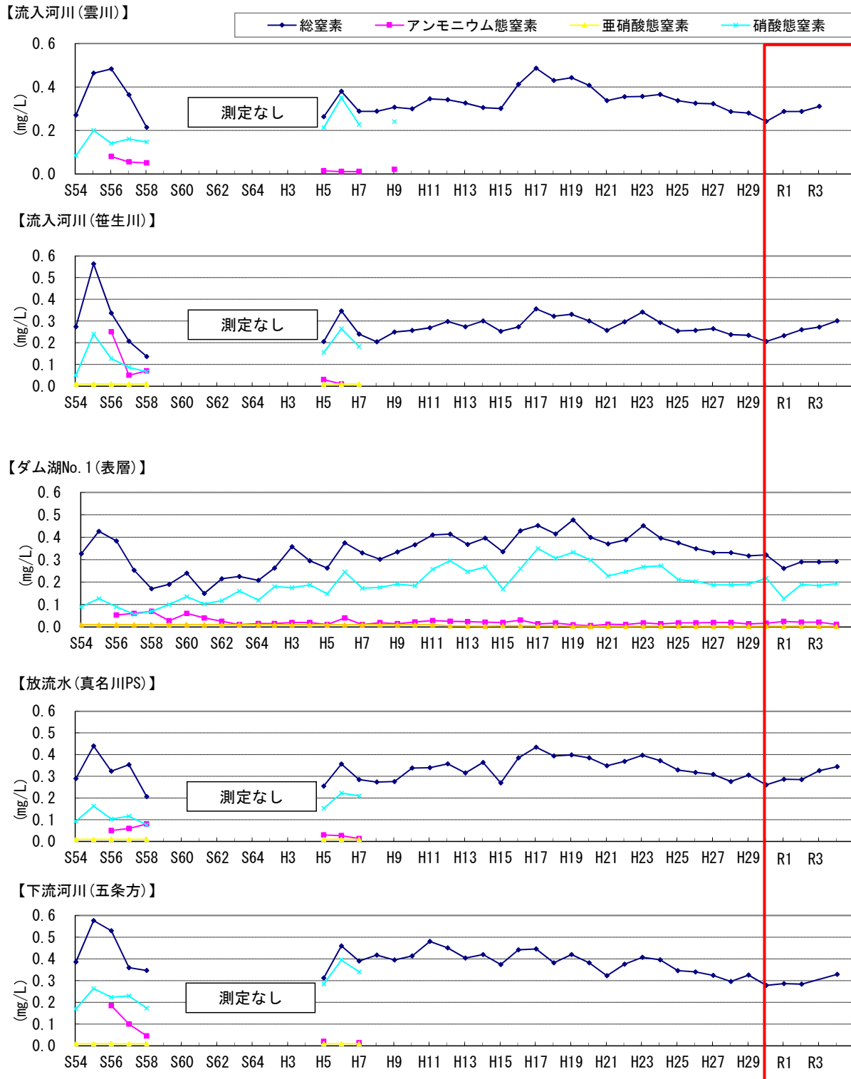
図 5.3-24(1) 窒素の構成形態別変化
