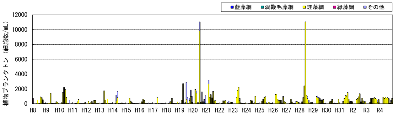
図 5.3-25 植物プランクトンの細胞数の経年変化(ダム湖No. 1)
