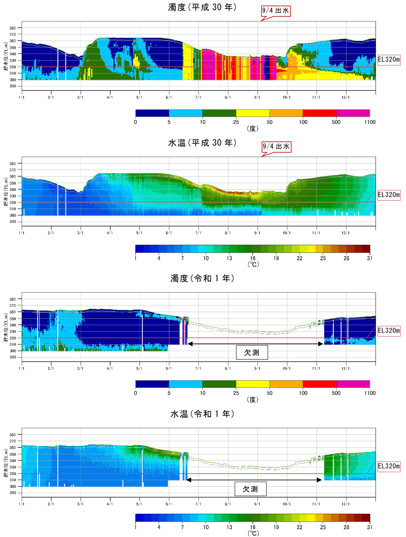
図 5.5-15(1) 真名川ダム連続観測結果(ダムサイト、水温・濁度) 【出典：真名川ダムダムサイト連続観測データ 平成30年～令和元年】
