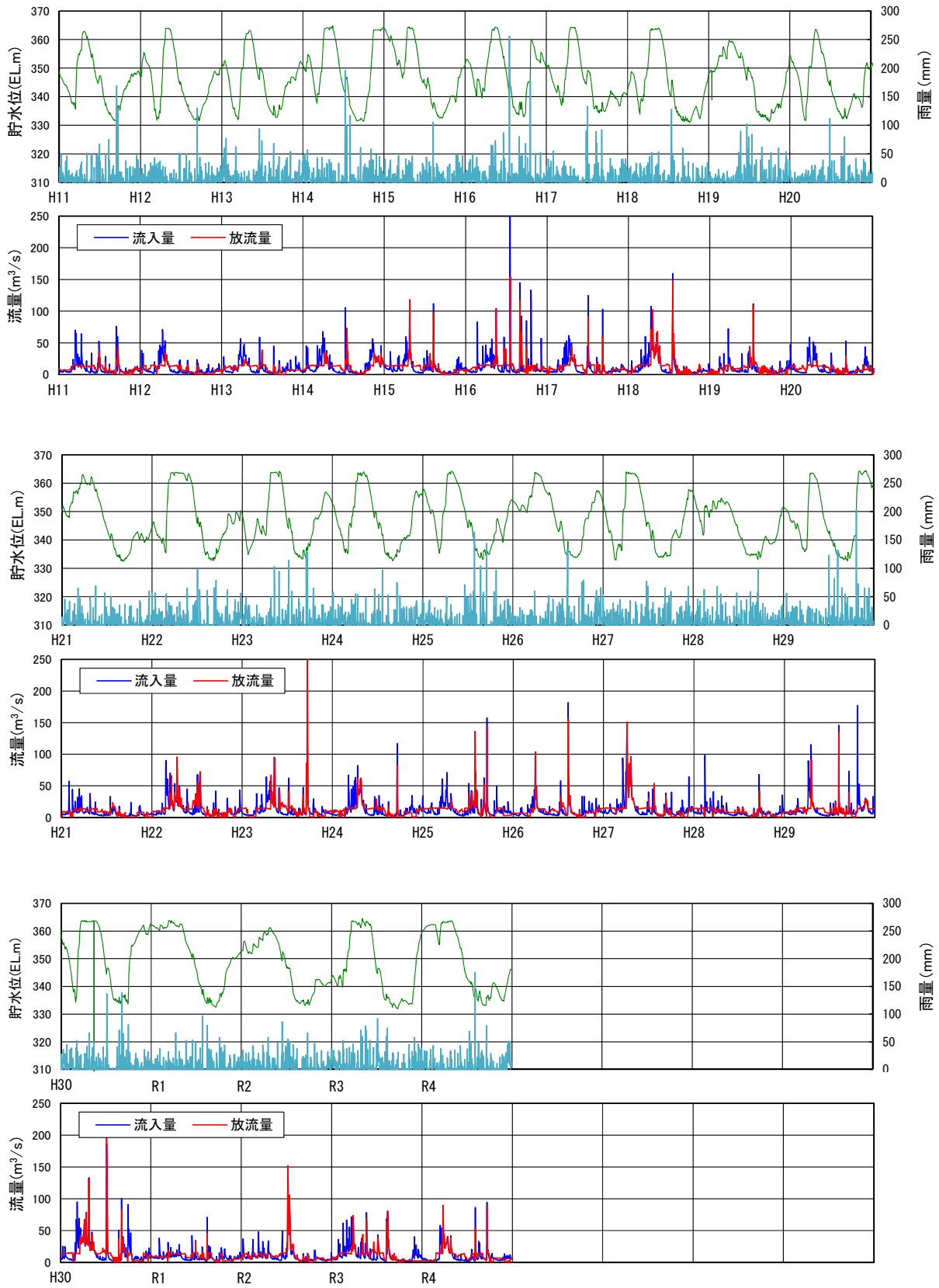
図 5.3-2(2) 真名川ダムにおけるダム諸量と日降水量 【出典:平成30年度 真名川ダム定期報告書 平成31年3月】 【出典:真名川ダム管理年報 平成30年～令和4年】
