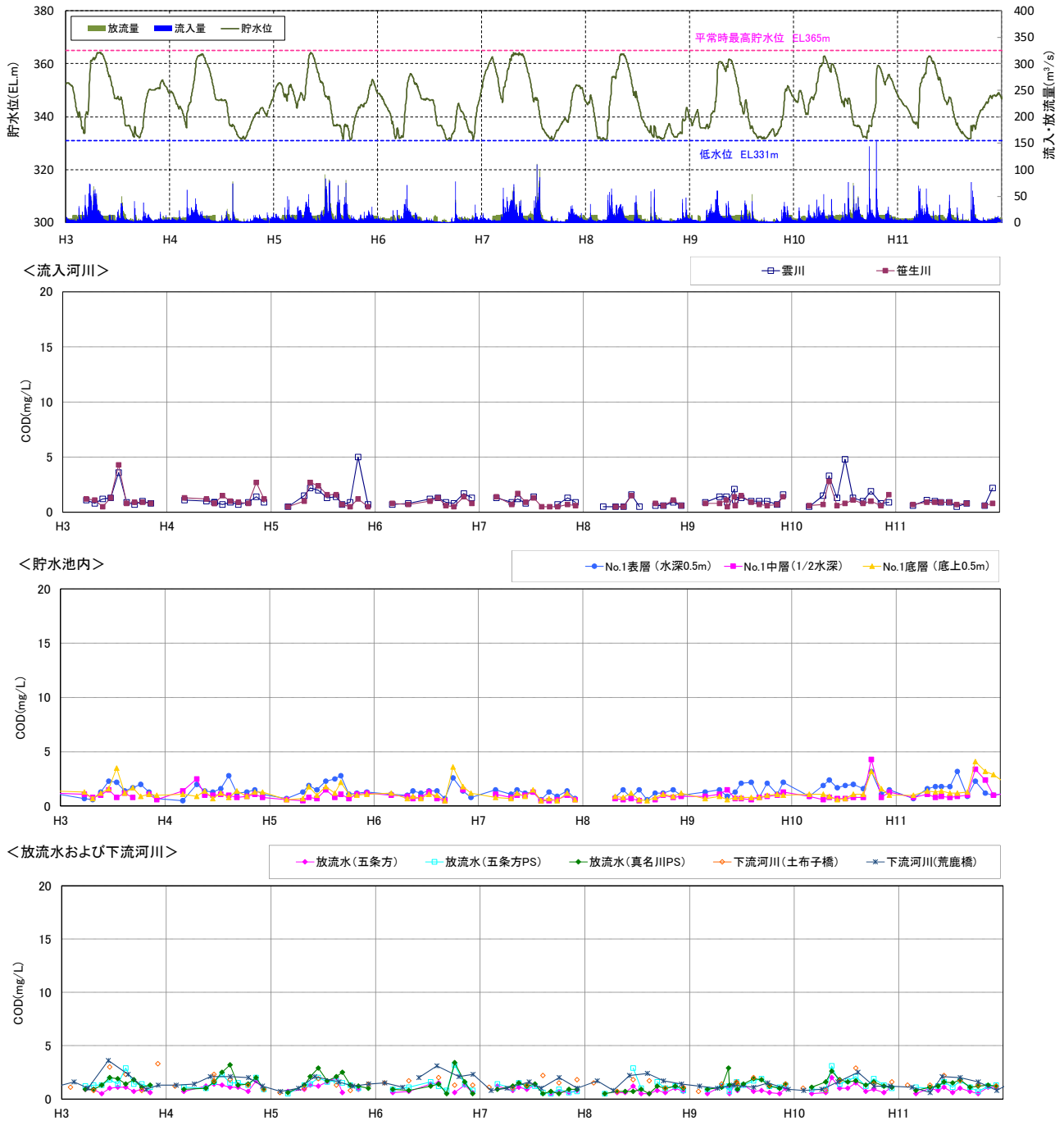
図 5.3-16(3) 流入河川、貯水池内、放流水及び下流河川の水質の経月変化 (COD : H3~H11)
