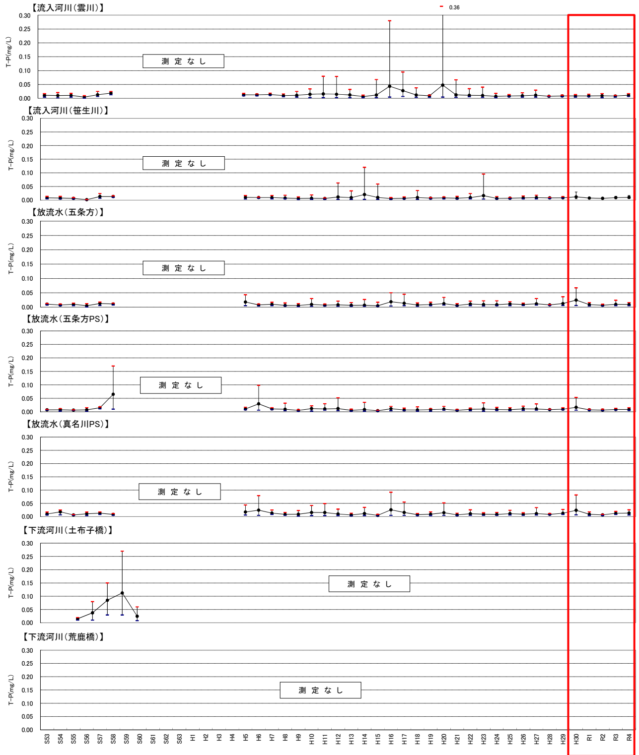
図 5.3-9(7) 各地点における流入河川、放流水及び下流河川の水質の経年変化(T-P) 【出典：平成30年度 真名川ダム定期報告書 平成31年3月】 【出典：水質調査業務報告書(真名川ダム)・データ 平成30年～令和4年】 【出典：福井県公共用水域水質測定結果 平成30年～令和4年】
