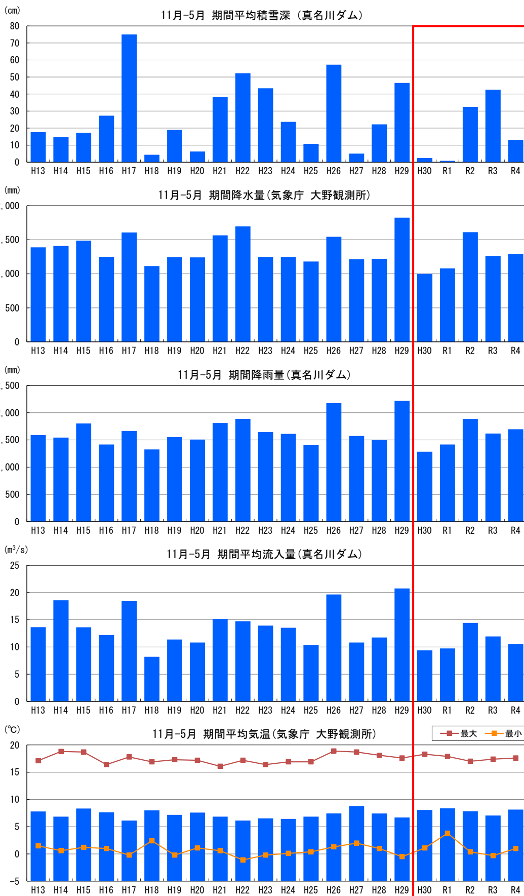
図 3.4-7 11月-5月の経年変化 (真名川ダム) 【出典：平成 13～令和 4 年度 真名川ダム諸量気象月報、真名川ダム管理年報、大野観測所データ (気象庁)】
