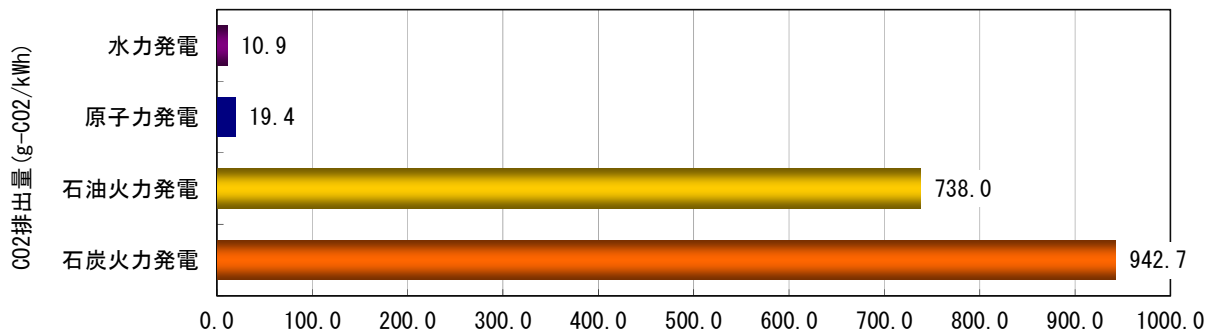
図 3.4-5 1kWを1時間発電する時のCO 2 排出量の比較
