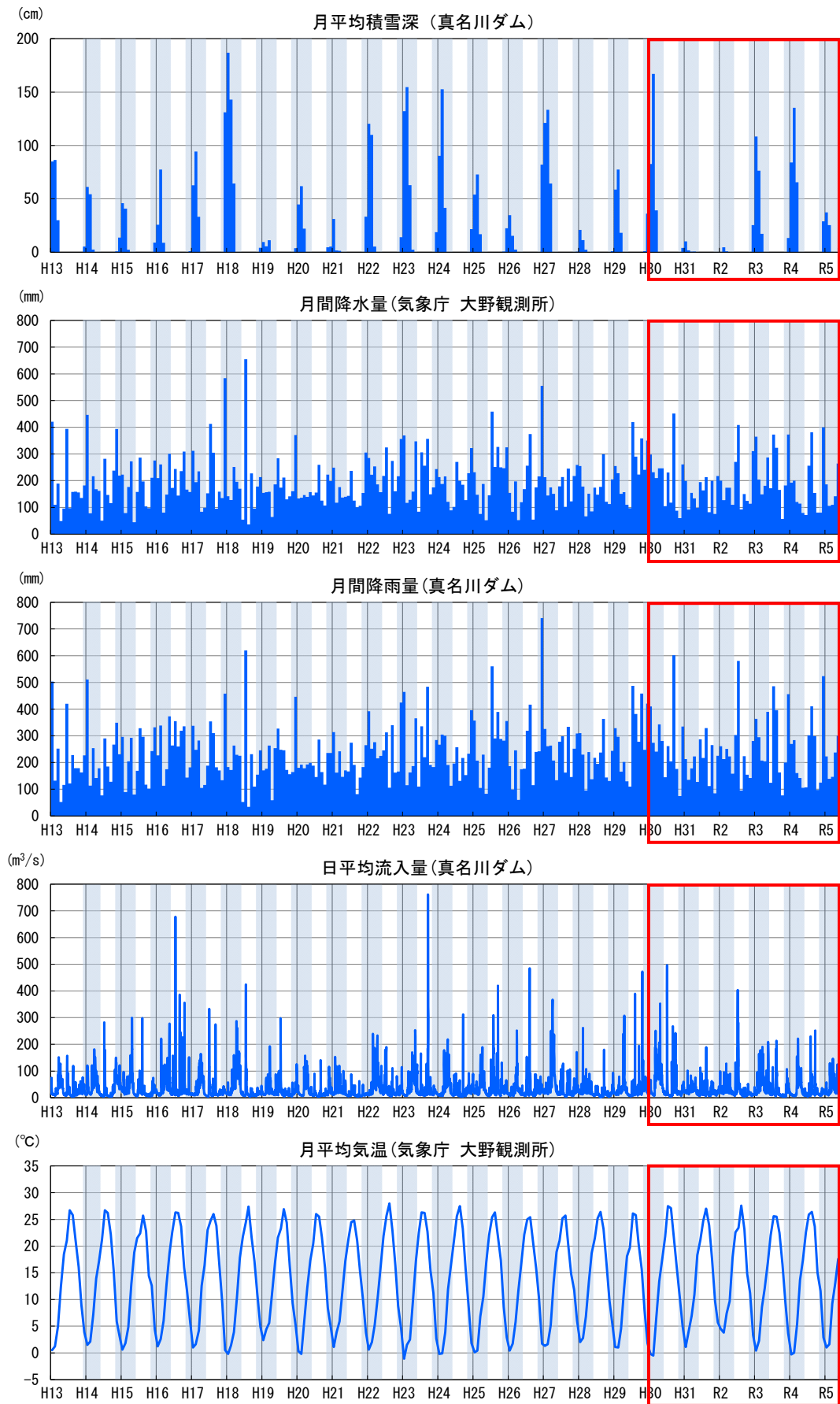
図 3.4-10 時系列変化 (真名川ダム)
