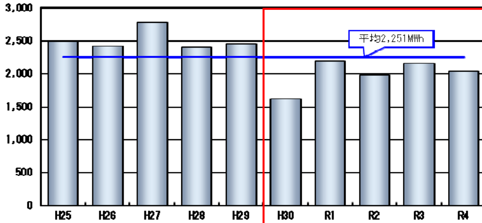
図 3.3-8 発電電力量実績 (管理用発電)
