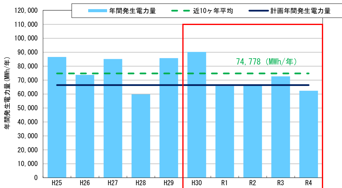
図 3.3-5 発電電力量実績
