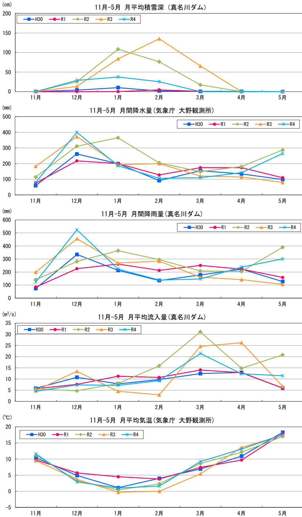
図 3.4-8 経月変化 (真名川ダム)
