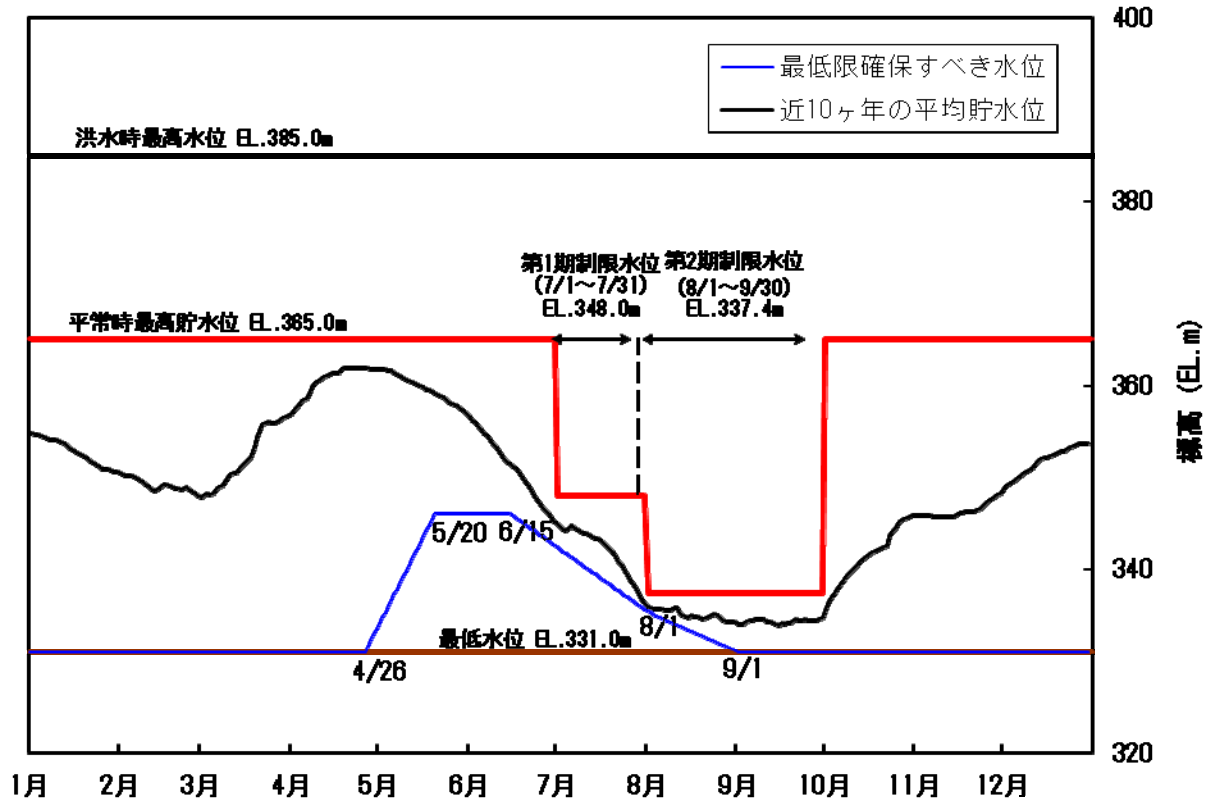
図 3.2-2 貯水池運用計画図
