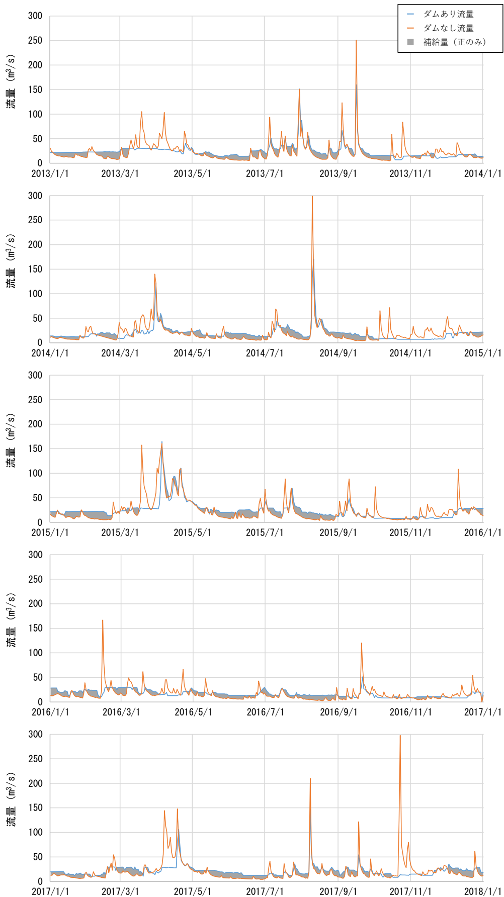
図 3.4-1 五条方下流におけるダムありなしの流量比較（平成25年～平成29年）
