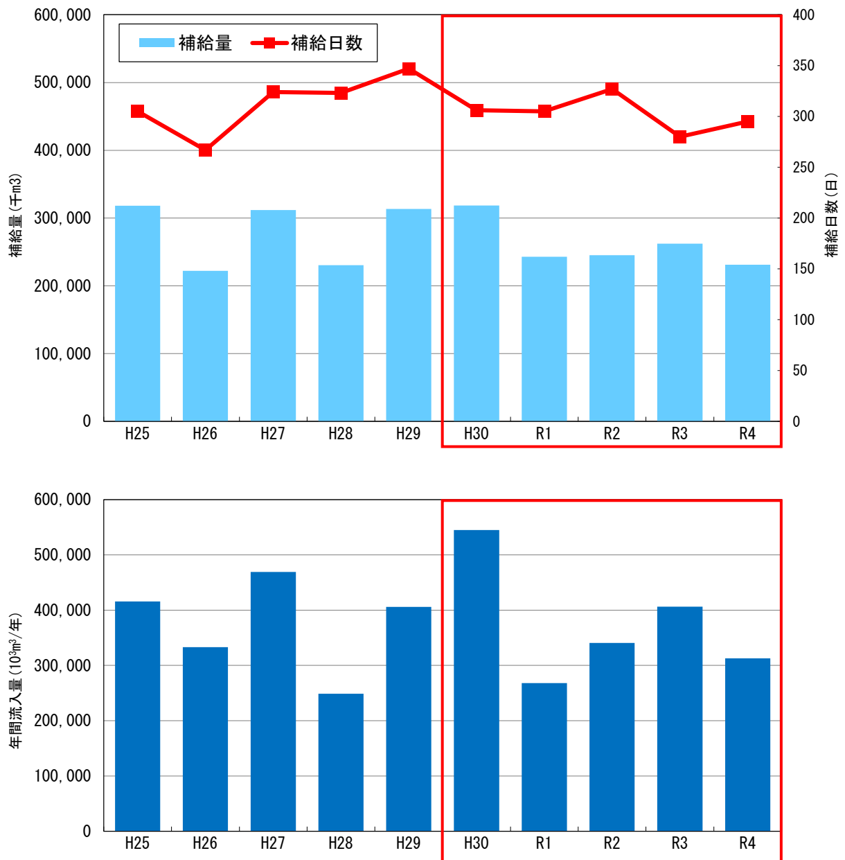
図 3.3-4 発電補給量実績(真名川発電所)と年間総流入量
