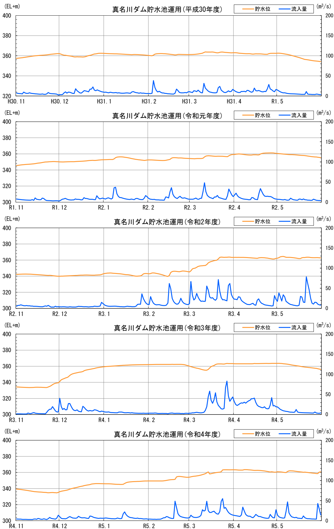
図 3.4-9 貯水池運用（真名川ダム）
