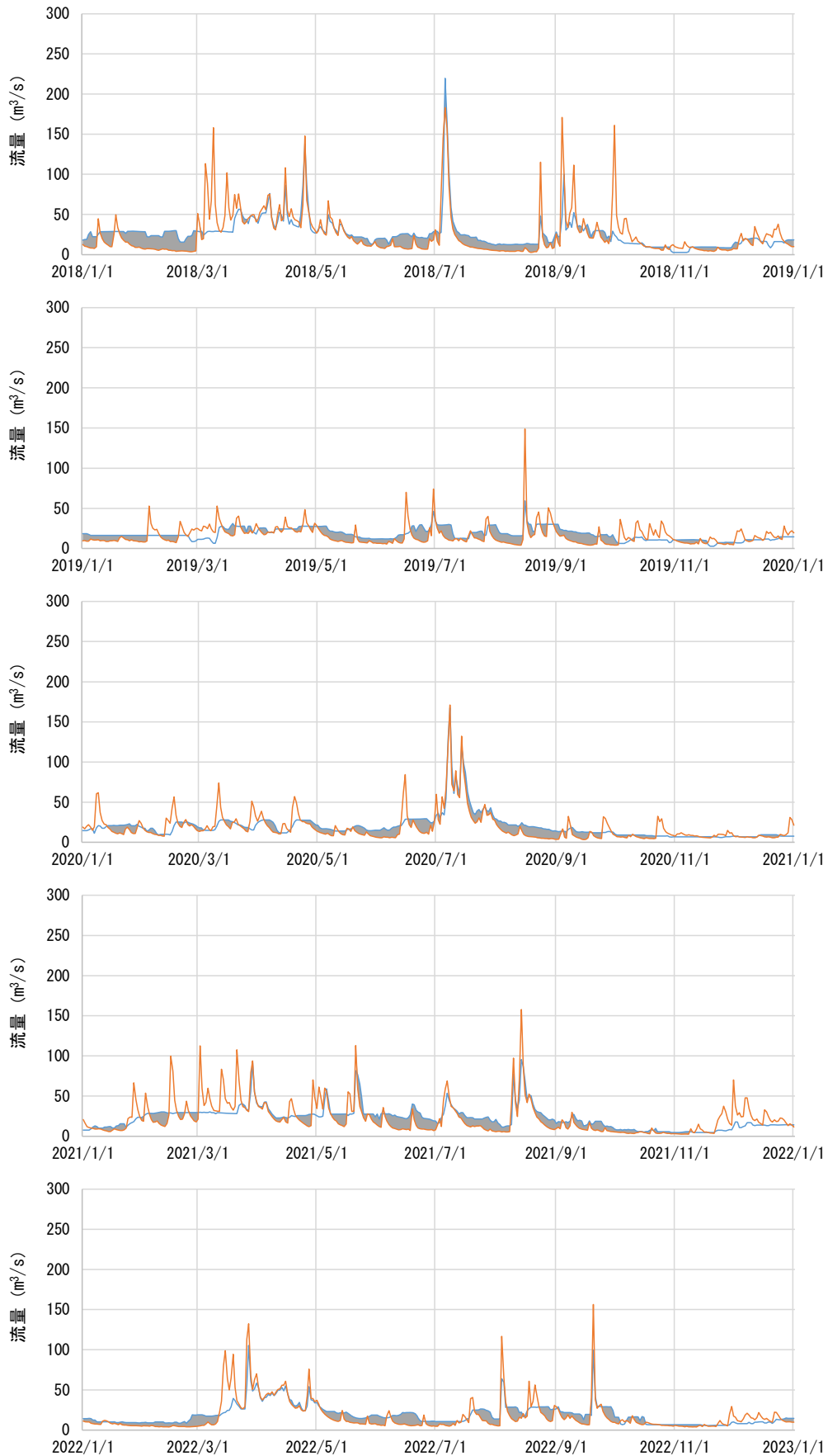
図 3.4-2 五条方下流におけるダムありなしの流量比較（平成30年～令和4年）
