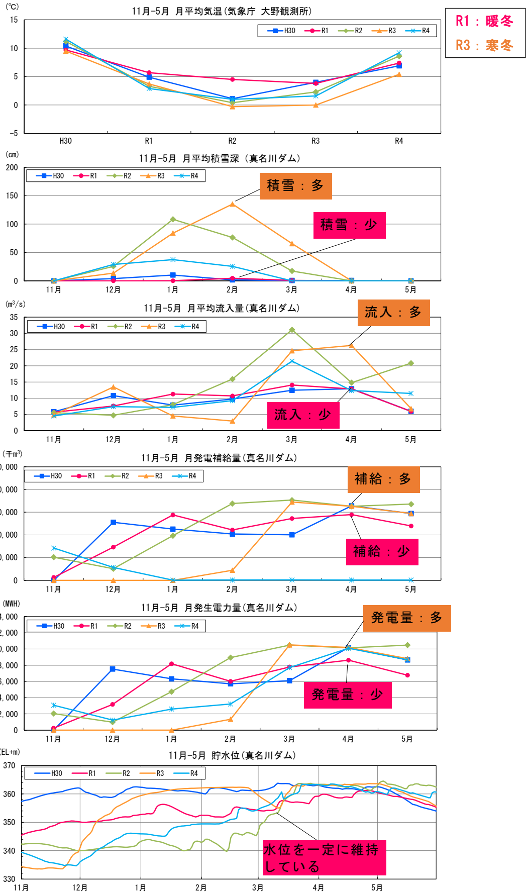
図 3.4-11 暖冬・寒冬と発電電力量の関係 (真名川ダム)
