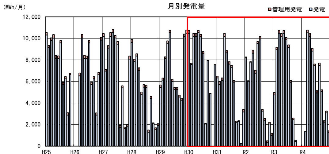
図 3.3-6 発電電力量実績(月別)
