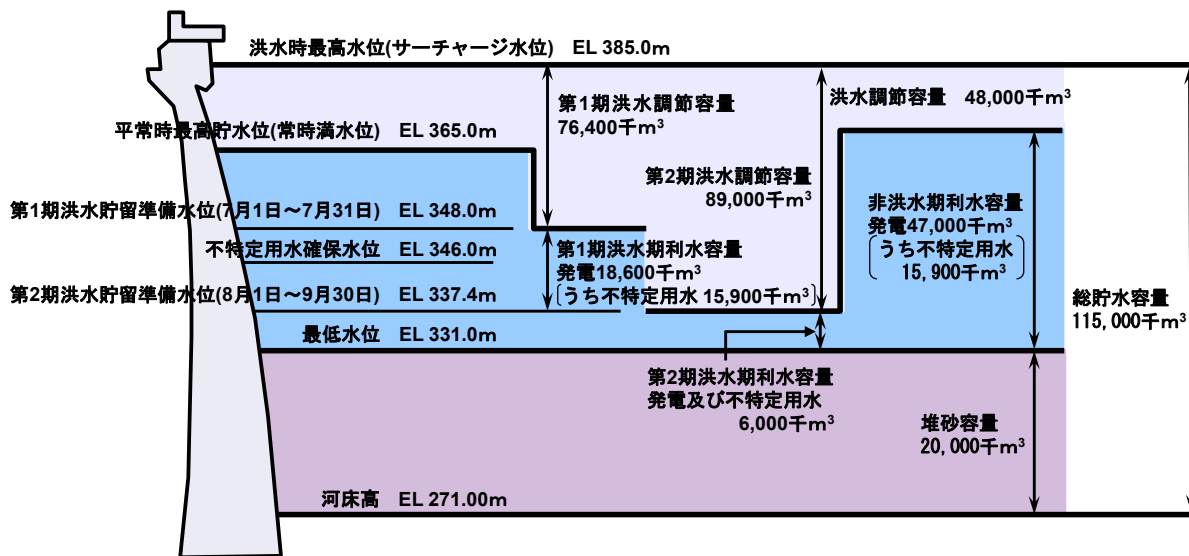
図 3.2-1 真名川ダム貯水池容量配分図
