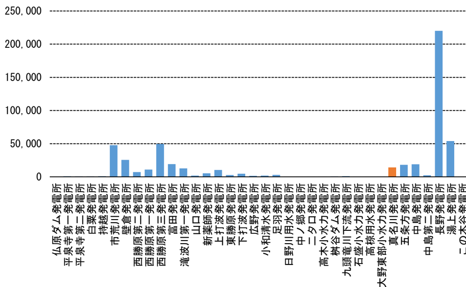
図 3.4-4 九頭竜川水系水量発電所 最大出力
