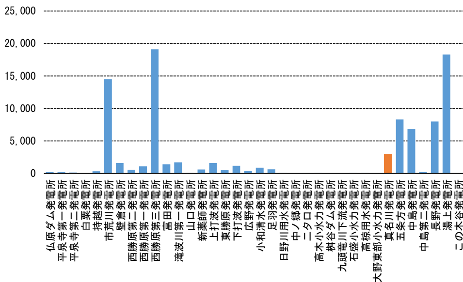
図 3.4-3 九頭竜川水系水量発電所 常時出力
