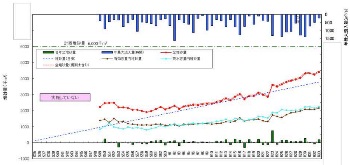
図 4.3-1 猿谷ダム貯水池堆砂量の経年変化
