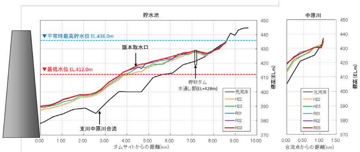
図 4.4-1 堆砂縦断面図
