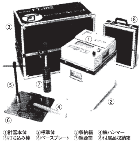
図-4 計器の構成例（透過型）
