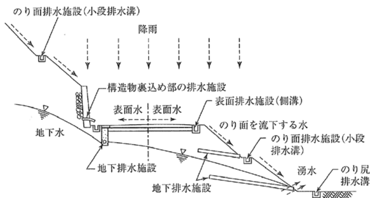
図 4-3-2 排水の種類
