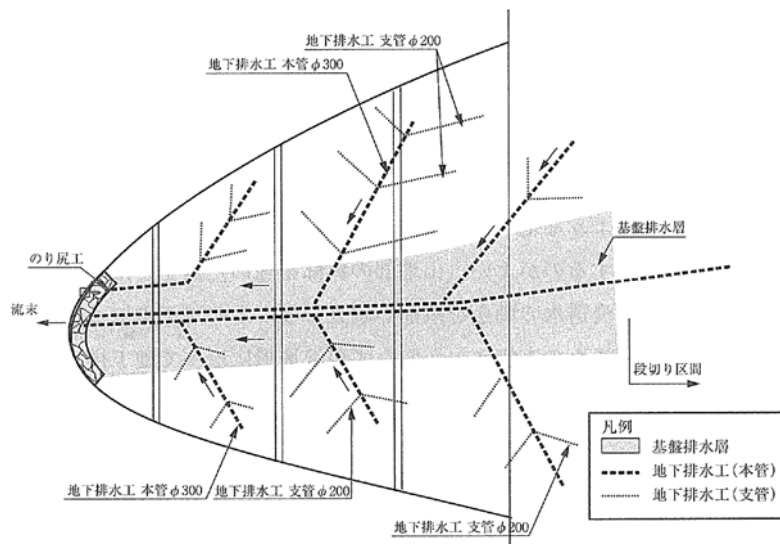
図 4-7-5 沢埋め盛土における地下排水溝及び基礎排水層の設置例
