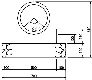
P1型 90度固定基礎
