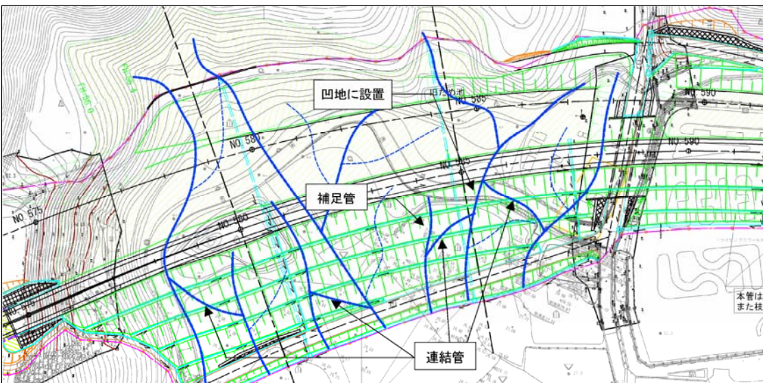
図 4-8-8 盛土面が平坦な場合の暗渠排水配置計画例
