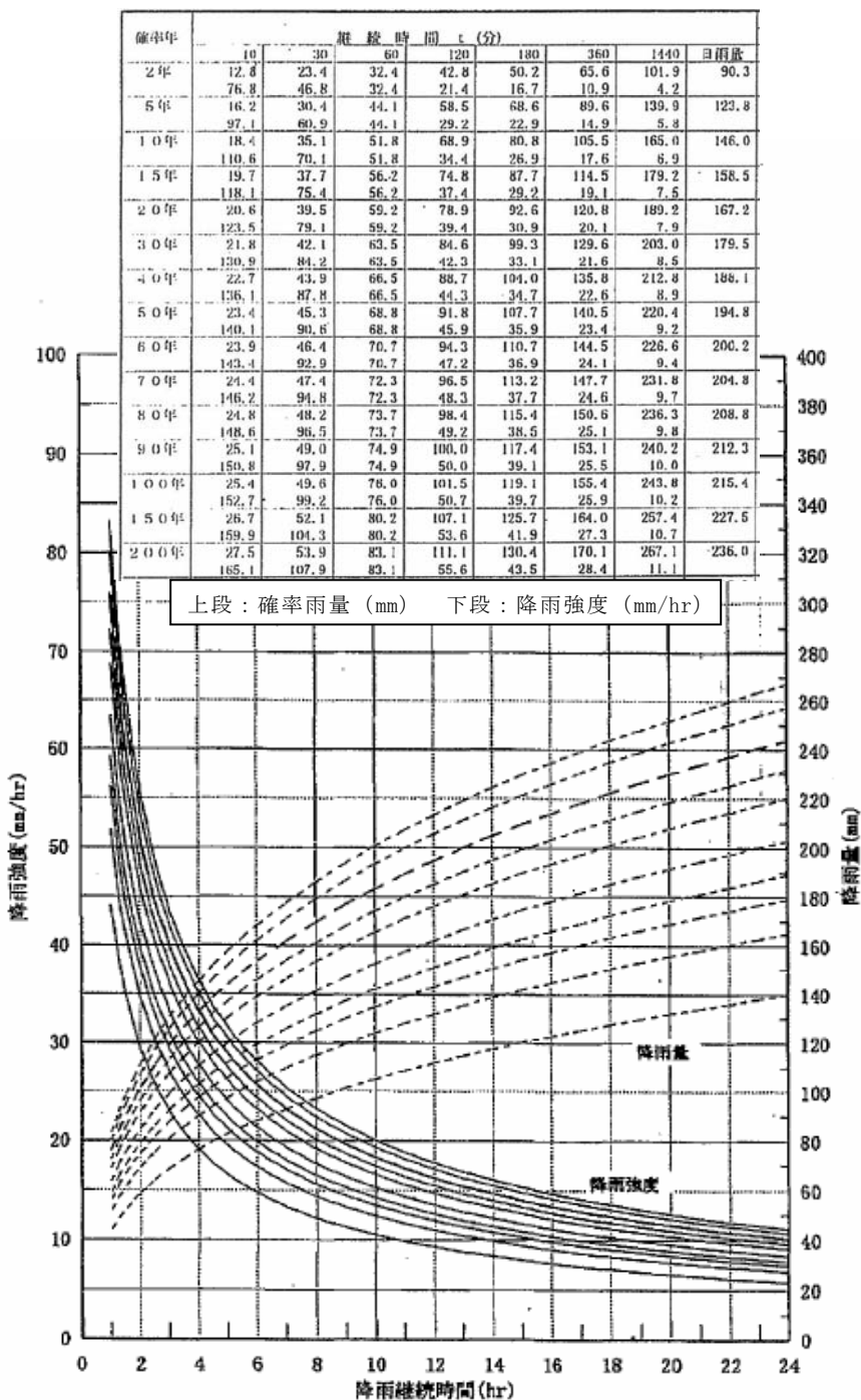
図 4-10-4 降雨強度曲線 (大阪府) 河内地区
