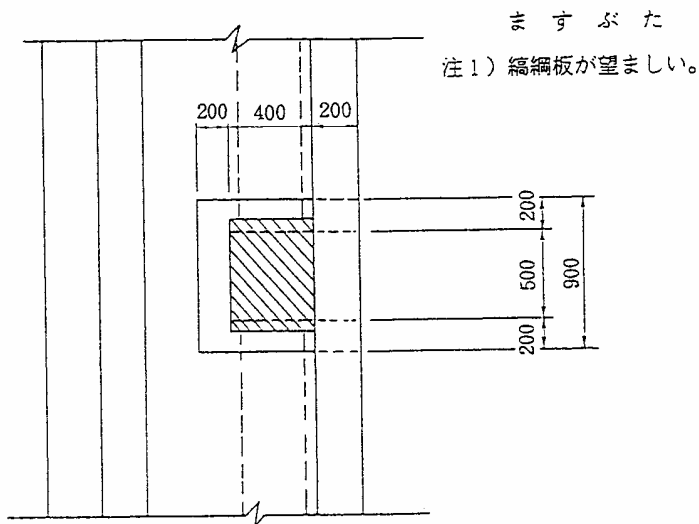
図 4-5-3 (b) 縦断管
