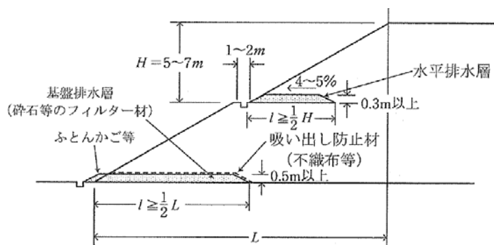
図 4-7-6 水平排水層及び基礎排水層の例
