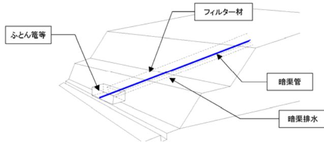
図 4-8-9 暗渠排水の流末処理の計画例
