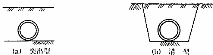
図4-6-1 埋設形式
