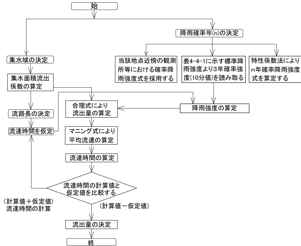
図 4-4-1 算出手順
