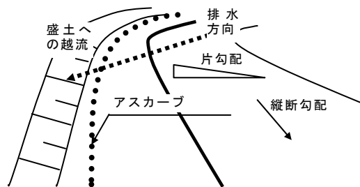
図 4-8-2 豪雨対策の例
