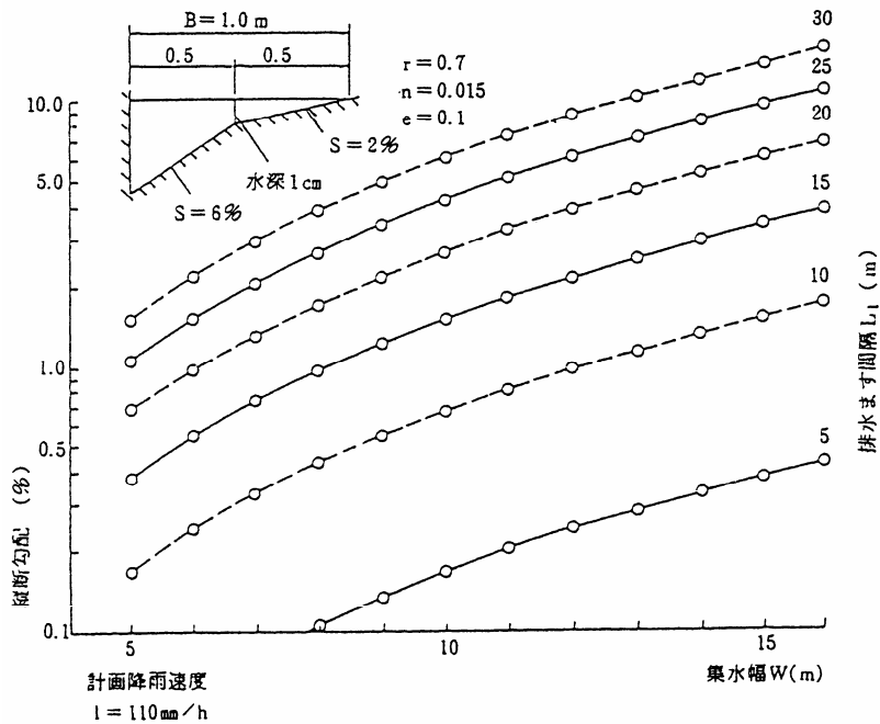
( 通水可能幅 B=1.0\text{m} 横断勾配 S=6\% (側溝部)、 2\% (道路部) マニングの粗度係数 n=0.015 落下率 \gamma=0.7 余裕率 e=0.1 ) 図 4-9-1(b) 集水ます間隔計算図表
