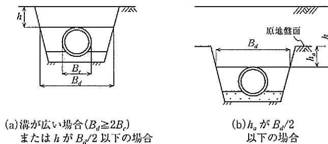
図4-6-2 突出型
