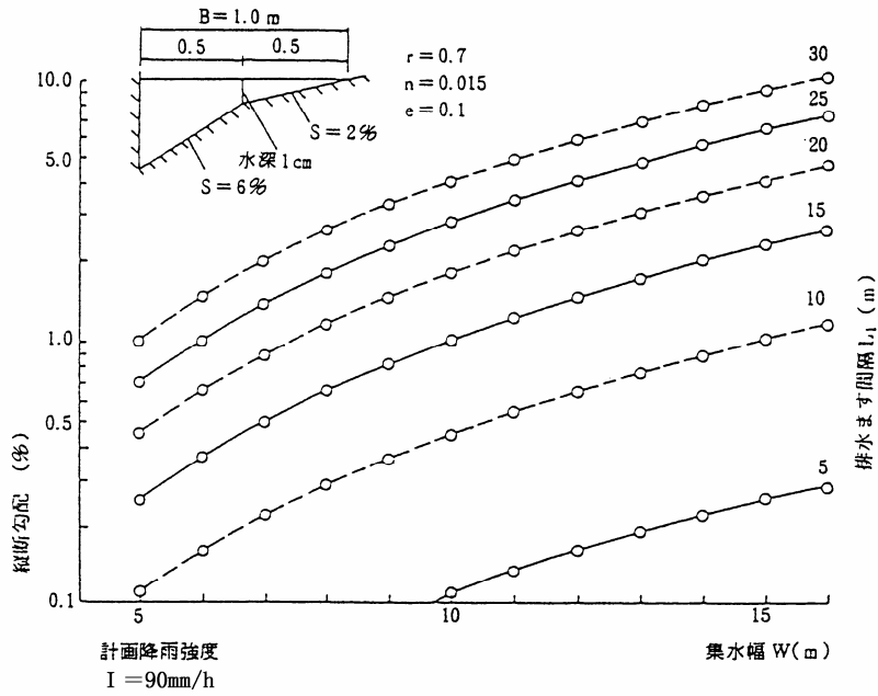
( 通水可能幅 B=1.0\text{m} 横断勾配 S=6\% (側溝部)、 2\% (道路部) マニングの粗度係数 n=0.015 落下率 \gamma=0.7 余裕率 e=0.1 ) 図 4-9-1(a) 集水ます間隔計算図表
