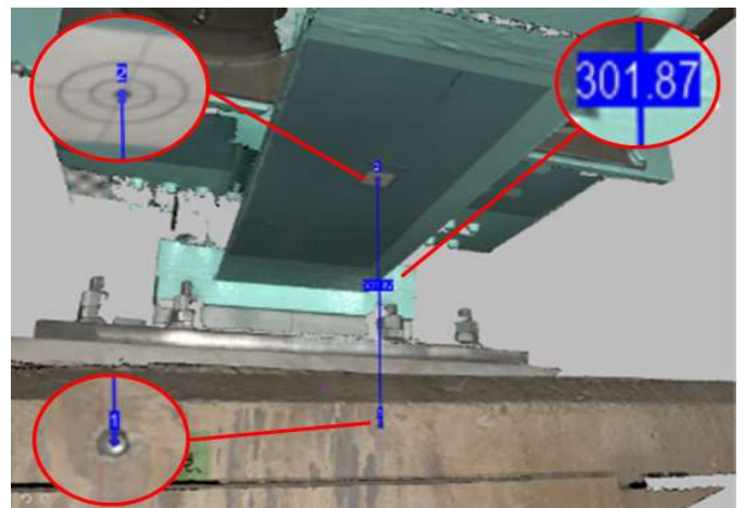
支承取替え後
