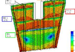
・P3橋脚
