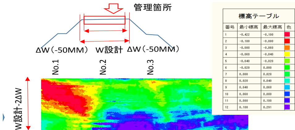
天端部出来形分布図
