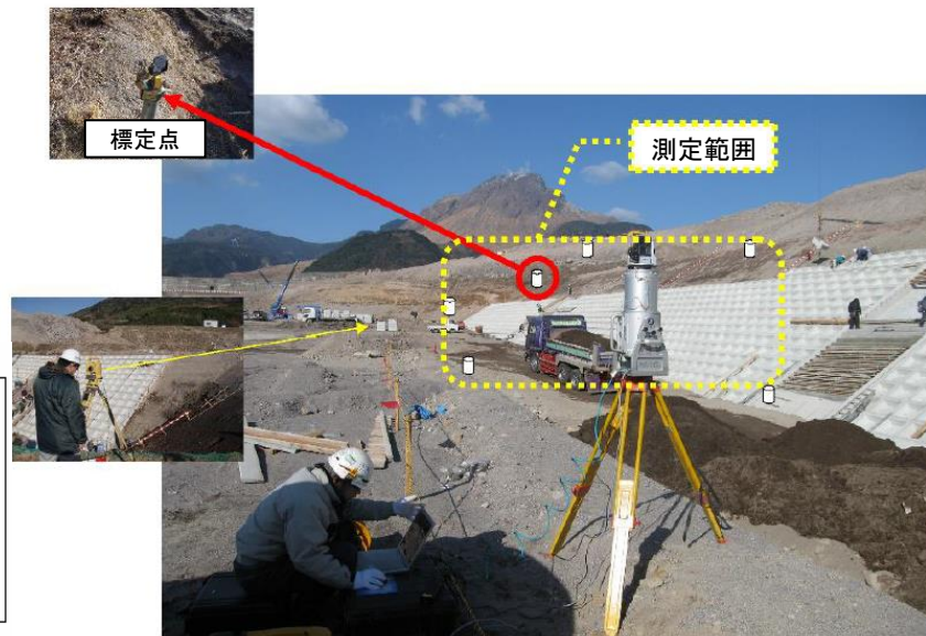
図 1-16 TLS と標定点の配置 (例)
