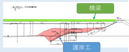
横断面図 (橋梁箇所)
