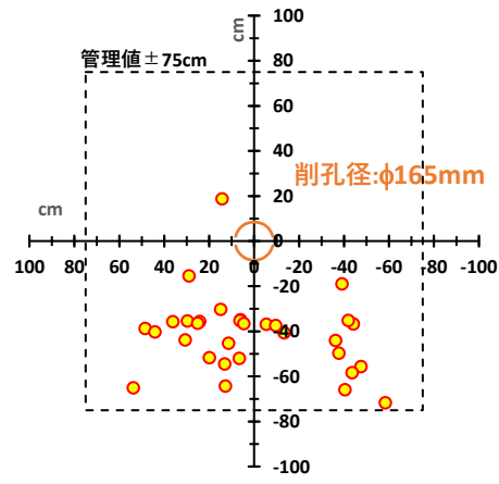
図-4 孔曲がり測定結果
