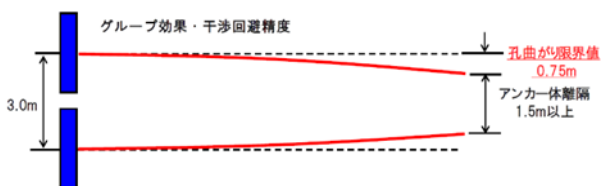
図-1 孔曲り概要図（水平方向の場合）
