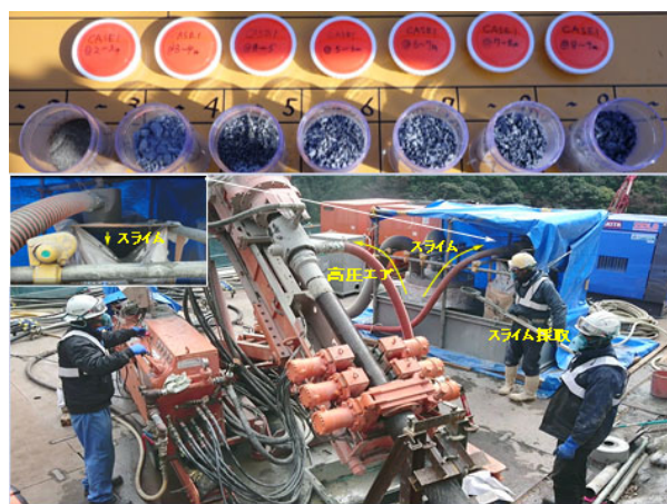
写真-3 削孔スライム採取状況
