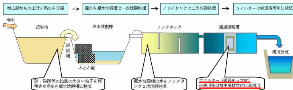
伐採材の木製チップを濁水濾過フィルターとして使用
