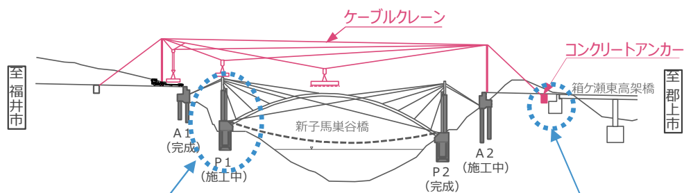
<縦断面図>
