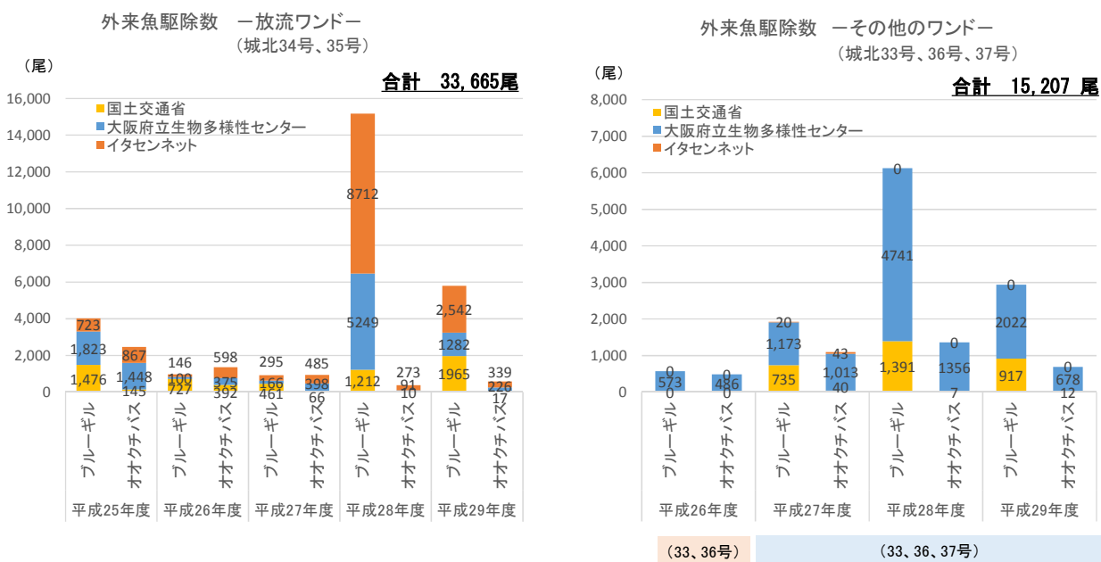
図3 城北地区における外来魚駆除
