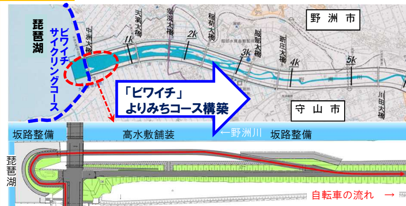
野洲川河口部の河川管理用通路整備状況
