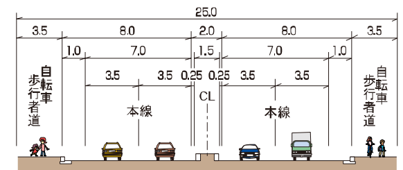
[ 標準断面図 ] 単位:m
