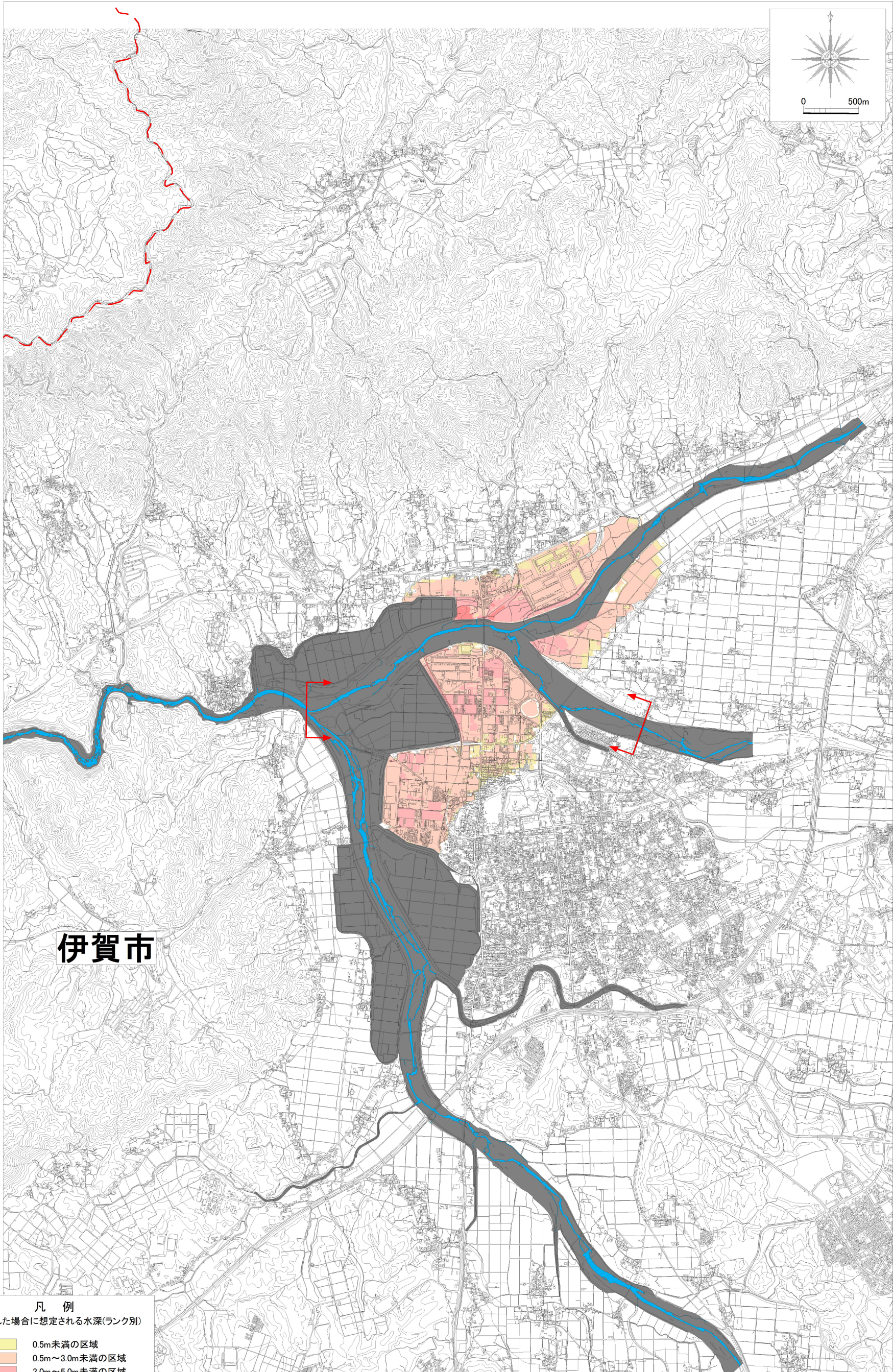
淀川水系服部川 洪水浸水想定区域図 (計画規模)
