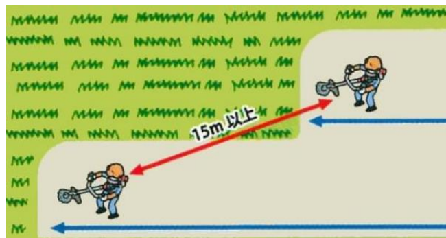
図 2.5 肩掛け式草刈機の離隔と法面での作業位置例 (参考図)
